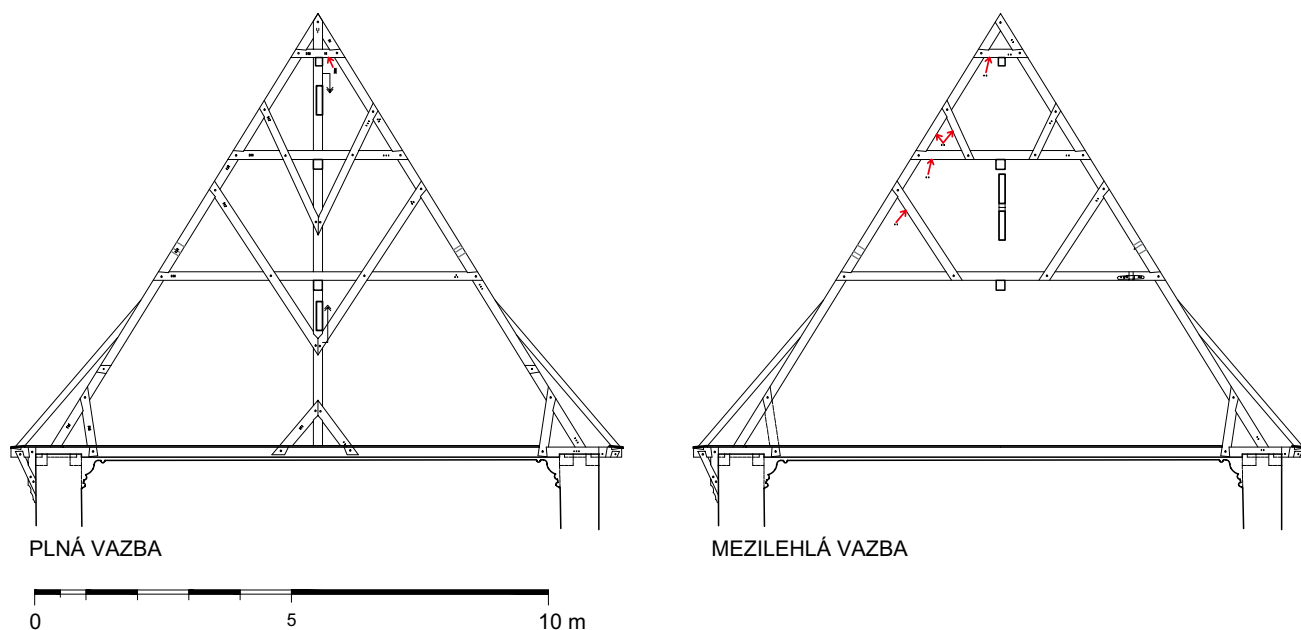
Obr. 6: Krov nad lodí, příčné vazby. Zobrazeny jsou vazby č. 2 a 5, včetně identifikovaných tesařských značek a dalších detailů.
