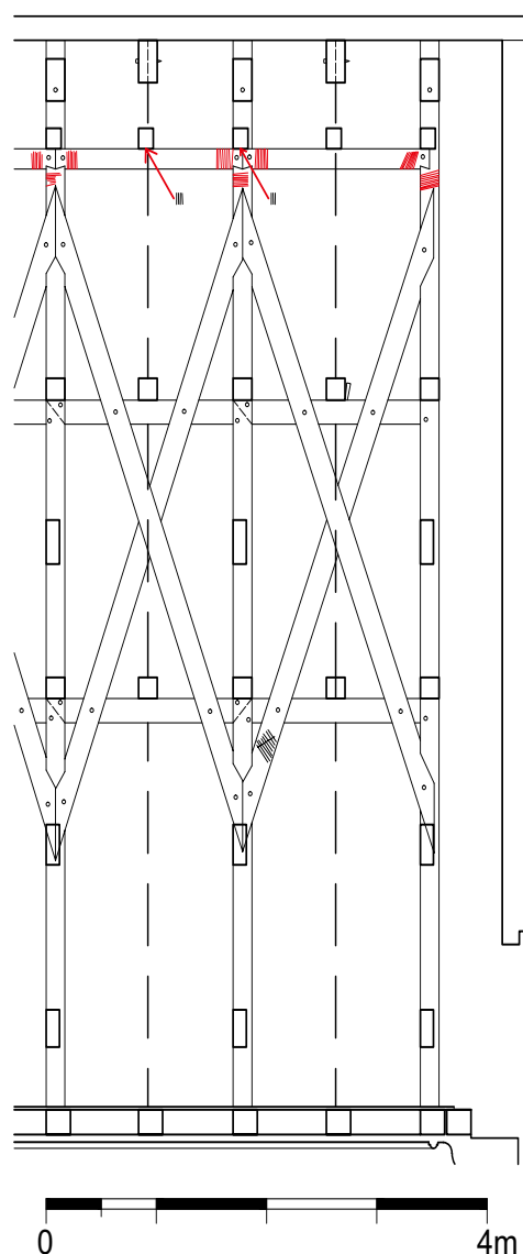
Obr. 7: Krov nad lodí, výřez z podélného vázání v rozsahu vazeb č. 1–5. Vyznačeny jsou dnes patrné kreslené značky
