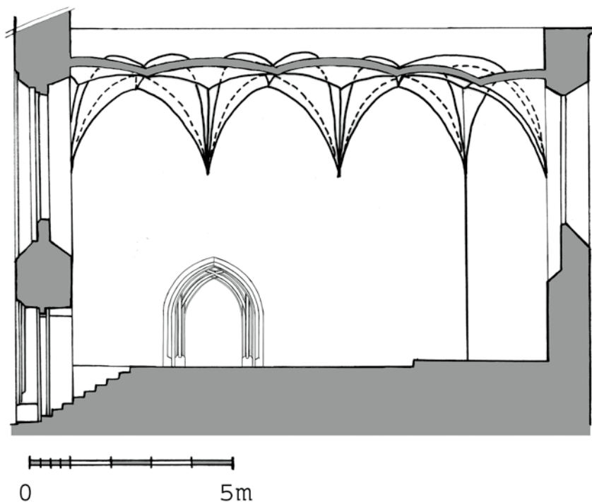
Obr. 7: Bor u Tachova, řez špitální kaplí sv. Alžběty, dnes sv. Jana Křtitele – pohled na severní stěnu (kresba R. Lavička, 2020).
