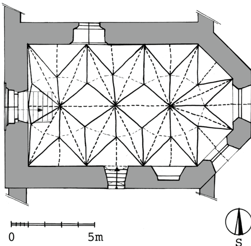
Obr. 6: Bor u Tachova, půdorys špitální kaple sv. Alžběty, dnes sv. Jana Křtitele (kresba R. Lavička, 2020).
