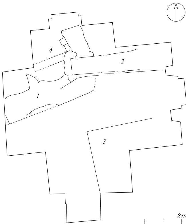
Obr. 11: Prazský hrad, bývalý areál Lvího dvorku, přizemí pod kaplí sv. Václava. Konstrukce nalezené v letech 1985–1986. Legenda: 1 a 3 – objekty předcházející stavbě kaple; 2 – konstrukce zřejmě související se stavbou kaple; 4 – fragmenty schodiště (podle I. Boháčová, o. c. v pozn. 47; upravit autor).
