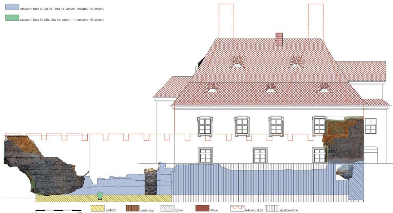
Obr. 32: Opava, Müllerův dům čp. 1, archeologický výzkum 2013, operativní průzkum a dokumentace 2016–2017. Východní fasáda objektu s vyznačením hlavních nálezových situací z období středověku. Barevně vyznačeny dochované podpovrchové i nadzemní relikty spojovací hradby městského opevnění a hradu (v řezu) a městské parkánové hradby ze závěru 14. století (transparentní modrá) a propust v hlavní hradbě z přelomu 14. a 15. století až první poloviny 15. století (transparentní zelená). Červenou čárkovanou linií rekonstrukce možné podoby hradních kuchyní s dvojicí dymníkových komínů a navazující průběh městské parkánové hradby (zaměření fasády M. Struhala, fotogrammetrie R. Kadlubiec, úpravy a celkové zpracování F. Kolář, 2021).
