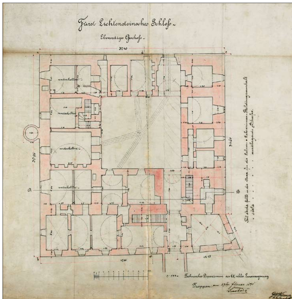
Obr. 8: Zaměření opavského zámku (přízemí) před plánovanou demolicí z února 1891, perokresba (ZA v Opavě, fond Zemská školní rada Opava, kart. 405).
