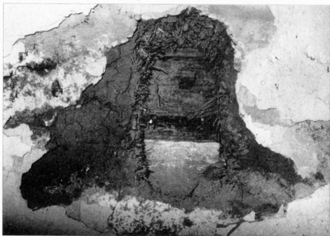
Obr. 9: Sonda v hliněné omazávce na stěně světnice s fragmenty starší úpravy povrchu. Zčernalý, původně oblý trám s bílenou spárou je dodatečně ztesaný se zatlučeným kolíkem pro přichycení hliněné omazávky.
