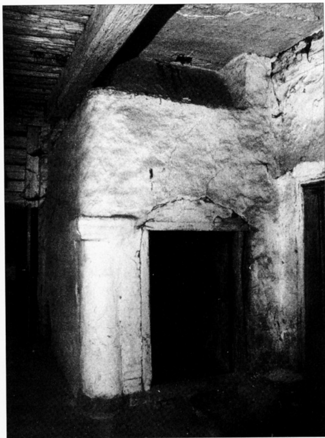
Obr. 6: Celkový pohled na kuchyň, vestavěnou do koutu síně. V nároží je původně volný kamenný sloup, nad kuchyní je spodní část komína. Vlevo jsou dveře průchodu na dvůr, vpravo vstup do světnice.
