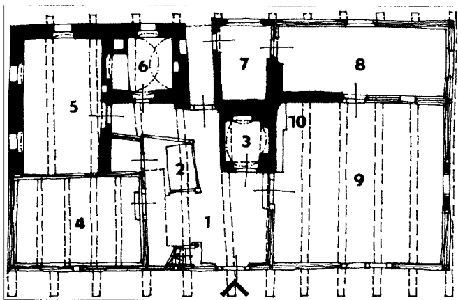
Obr. 4: Orientační půdorys přízemí domu.
