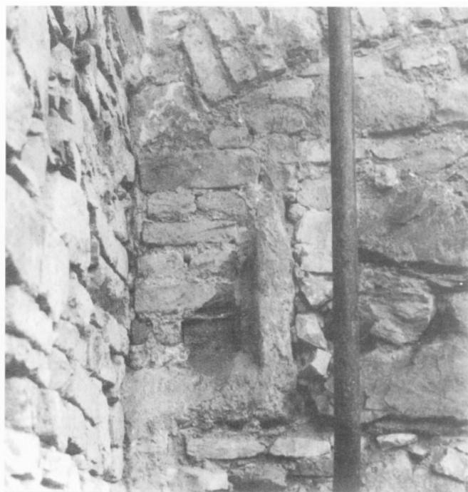
Obr. 9: Pohled na gotické ostění okénka vpravo od předstíně. Vpravo původní lomové zdivo, vlevo zdivo sínce, nad okénkem barokní zdivo s cihelným pasem.
