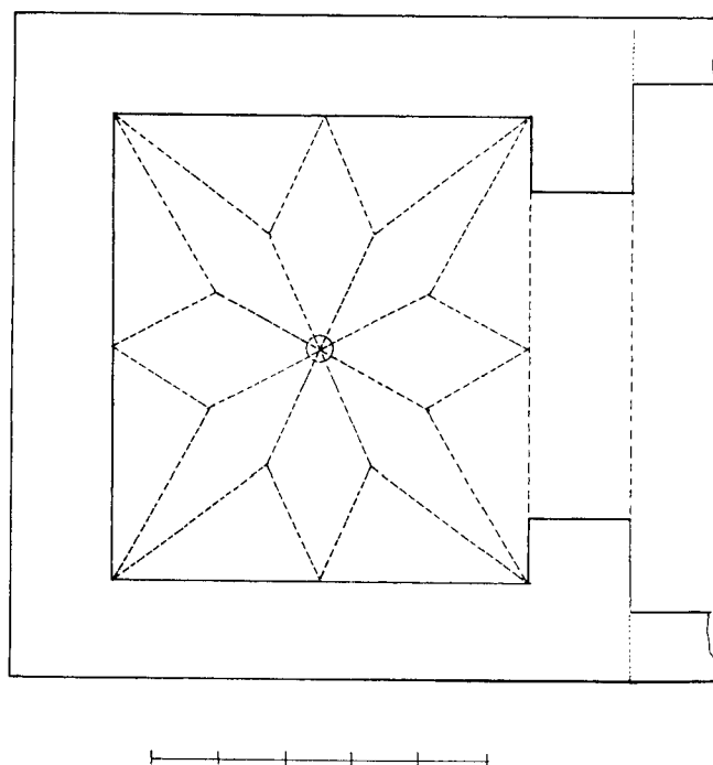
Obr. 13: Kostel sv. Martina ve Zbečně. Pravděpodobná podoba klenby v presbytáři - půdorys. (kresba Jan Žižka)
