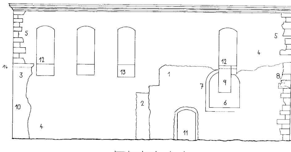
Obr. 3: Kostel sv. Martina ve Zbečně, jižní průčelí se zakreslením nálezů (kresba Jan Žižka 1992):
