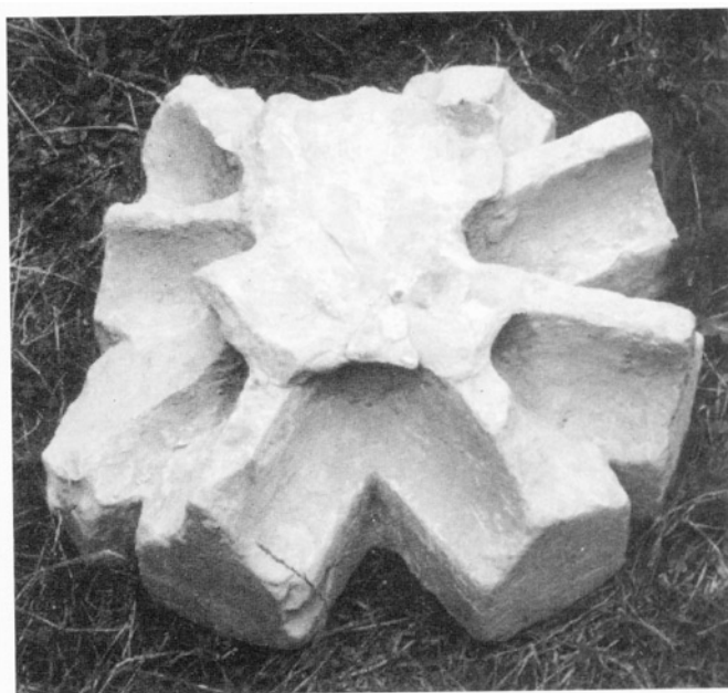
Obr. 12: Svorník po vyjmutí ze zdiva.
