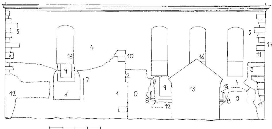
Obr. 7: Kostel sv. Martina ve Zbečně, severní průčelí se zakreslením náleží:
