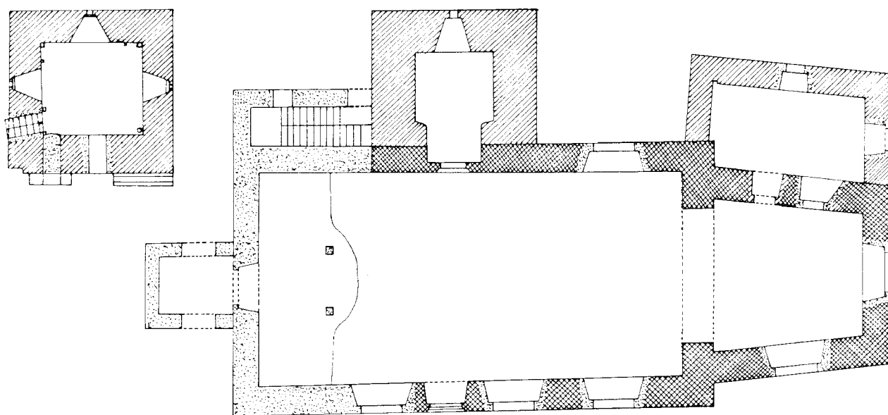
Obr. 1: Půdorys kostela podle zaměření v Soupisu a půdorys 2. patra věže. Mřížkovane ranne gotické, šrafovane pozdne gotické a tečkovanne barokni zdivo.
