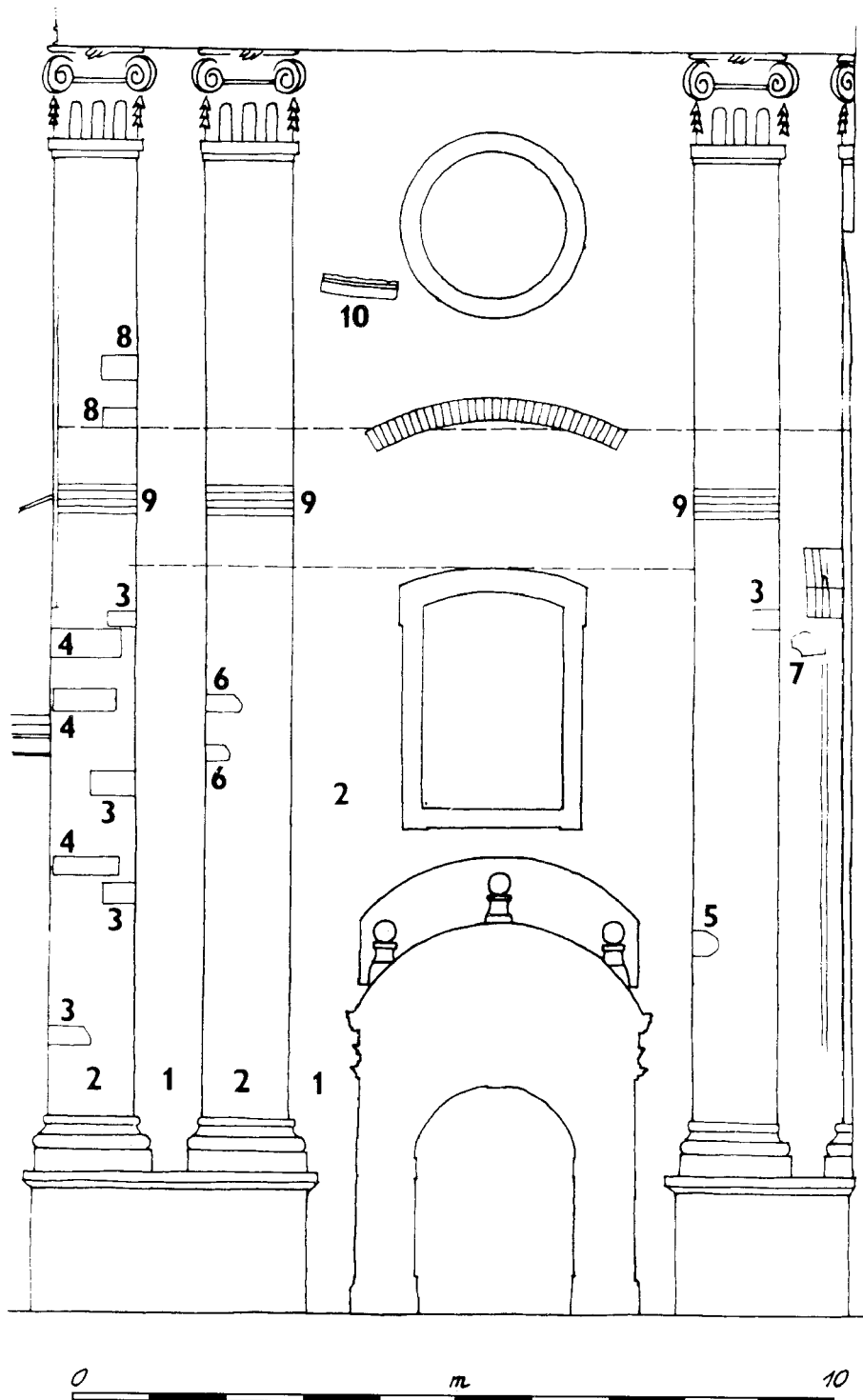
Obr. 1: Sázava (okr. Kutná Hora), kostel sv. Prokopa. Výsledky průzkumu zdiva západního průčelí hlavní lodi.
