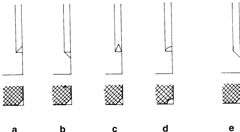
Obr. 8: Typy portálových soklů tábořských sklepů.
