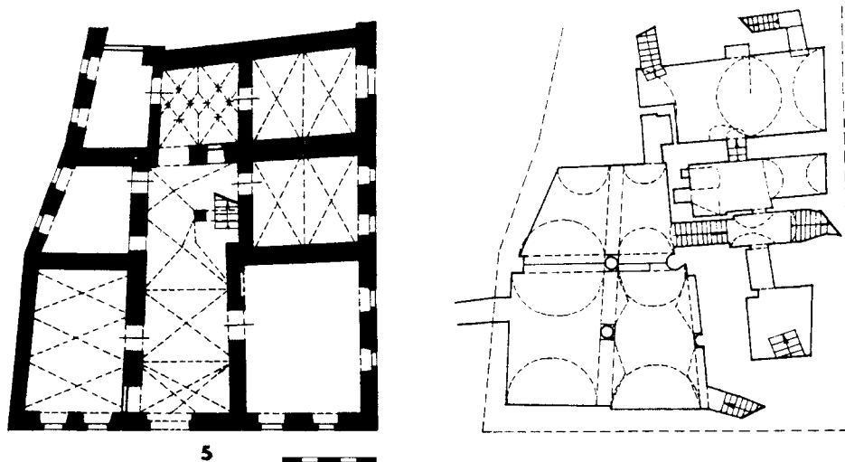
Obr. 5: Lichvicův dům čp. 5, přízemí a sklepy po roce 1532.
