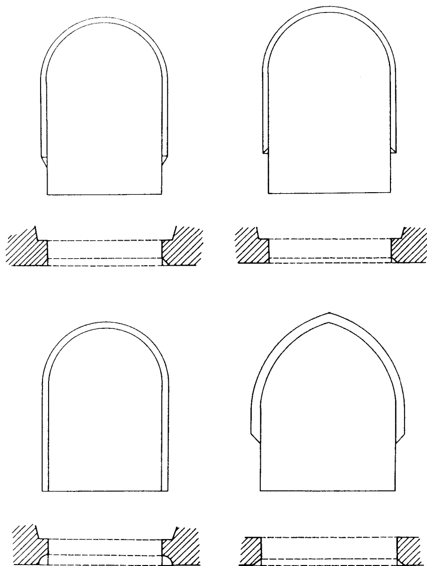
Obr. 7: Typy portálů tábořských sklepů.
