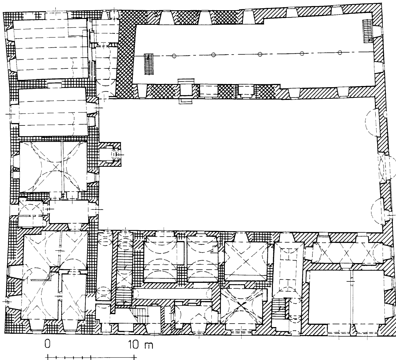
Obr. 5: Čečovice, zámek, půdorys 1. nadzemního podlaží. Křížkovaně šikmo zdivo gotické, křížkovaně kolmo renesanční. Šrafované svisle manýristické, šrafované šikmo barokní, šrafované přerušovaně klasicistní, bíle mladší a neurčené. (Zpracoval J. Anderle)
