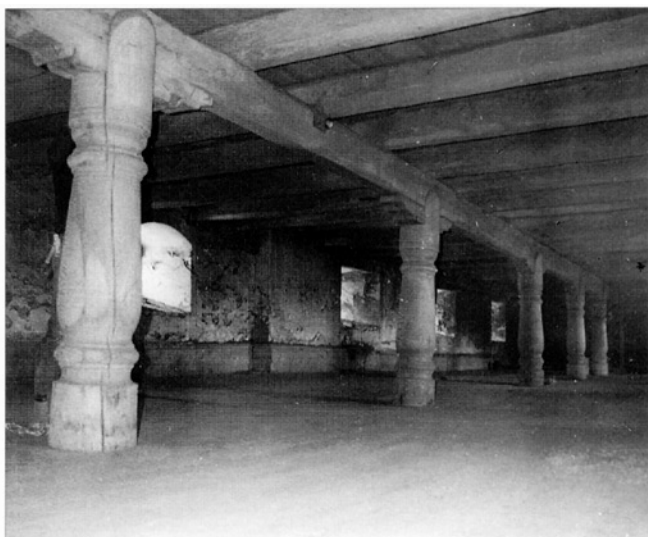
Obr. 6: Čechovice, zámek, 2. nadzemní podlaží sýpky. Stav r. 1991.
