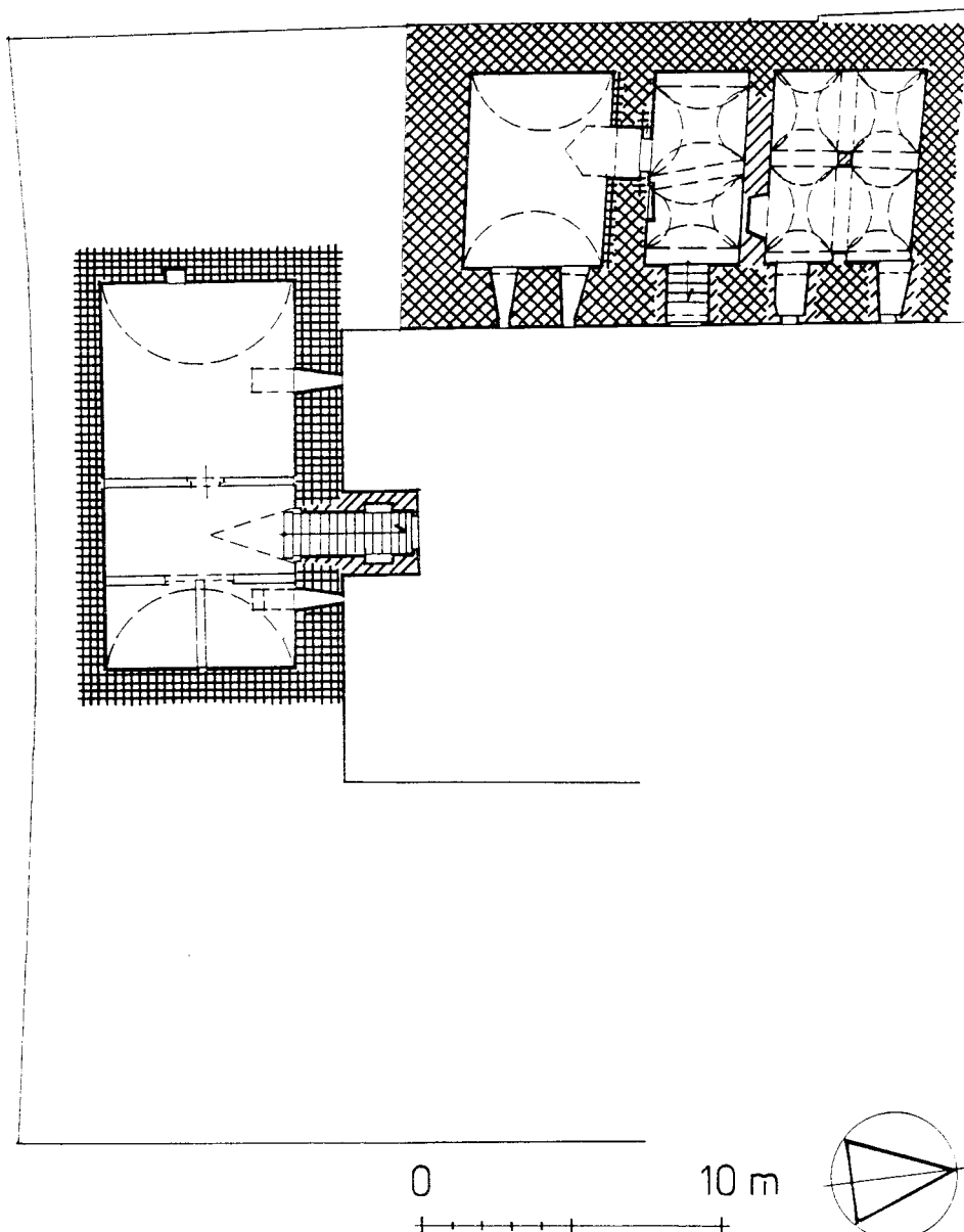
Obr. 4: Čečovice, zámek, půdorys suterénu. Křížkovane šikmo zdivo gotické, křížkovane kolmo renesanční, šikmo sraňované barokní. (Zpracoval J. Anderle)
