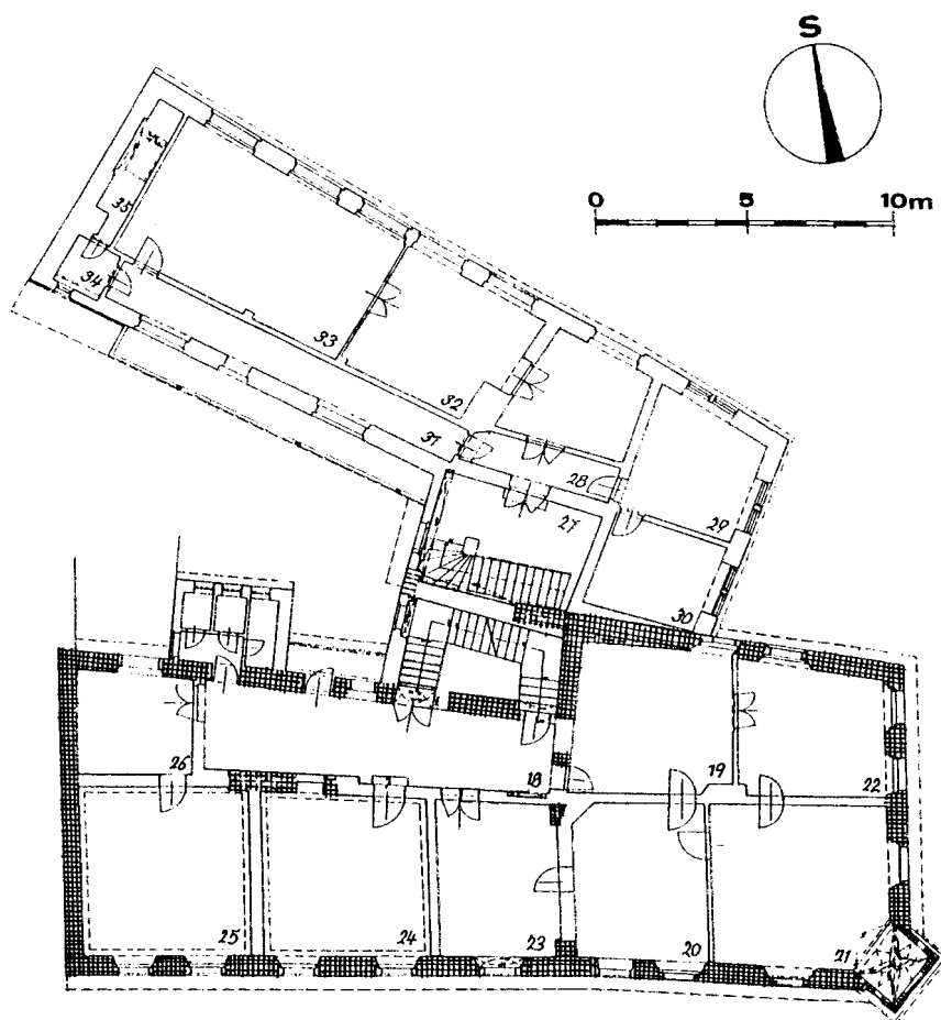
Obr. 6: Půdorys 1. patra ve stavebně historické analýze (mřížkovně značeno zdivo renesanční, ostatní je barokní a mladší).
