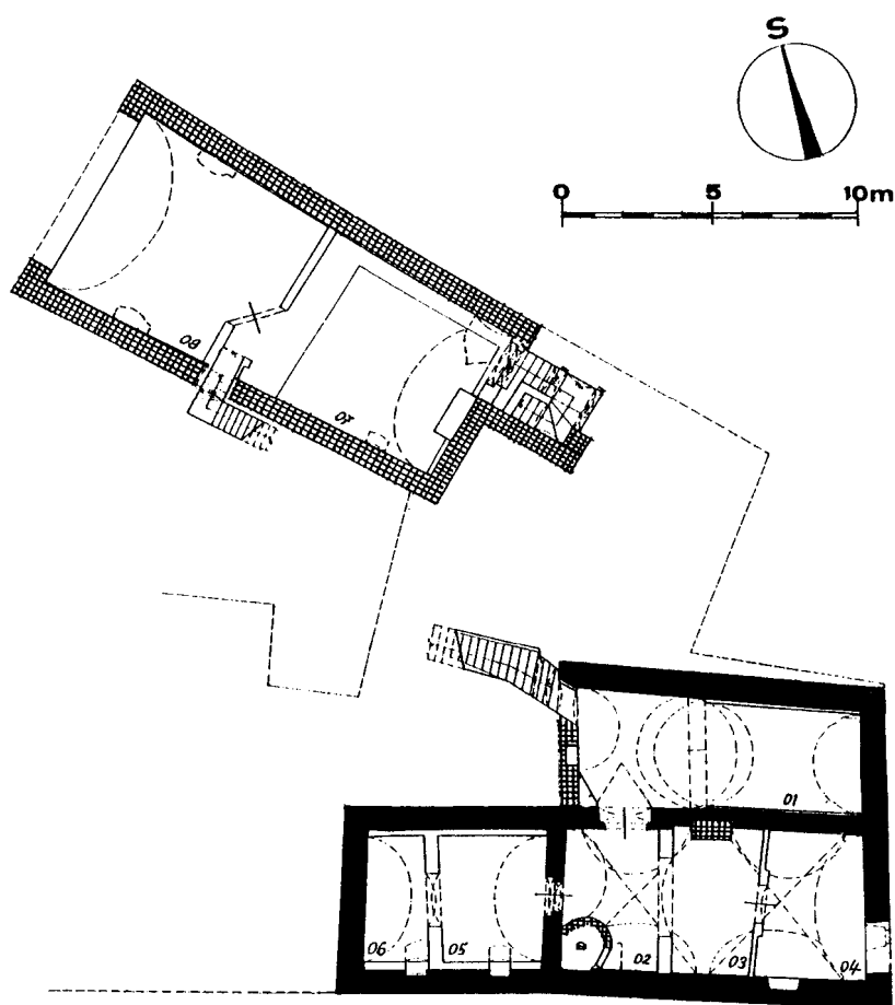
Obr. 4: Půdorys sklepů ve stavebně historické analýze (černě značeno zdivo gotické, mřížkovane renesanční, ostatní - mladší).
