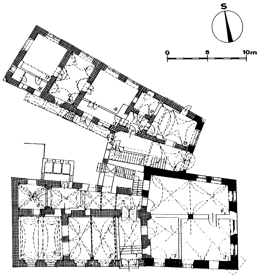
Obr. 5: Půdorys přízemí ve stavebně historické analýze (černě značeno zdivo gotické, mřížkované renesanční, ostatní - mladší).
