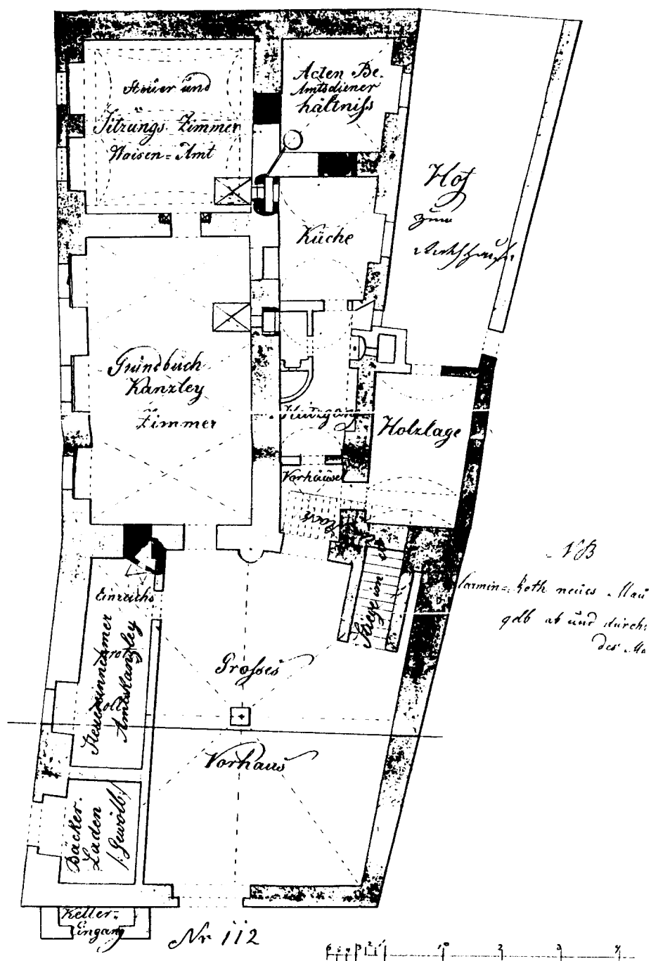
Obr. 7: Plán předního dílu staré radnice (čp. 4) z r. 1848 od stav. Hanse, dosud s čelním vstupem do mázhausu a se starým schodištěm. (MZA - VZS 1850 - 1897, sg. B 8 - A 8).
