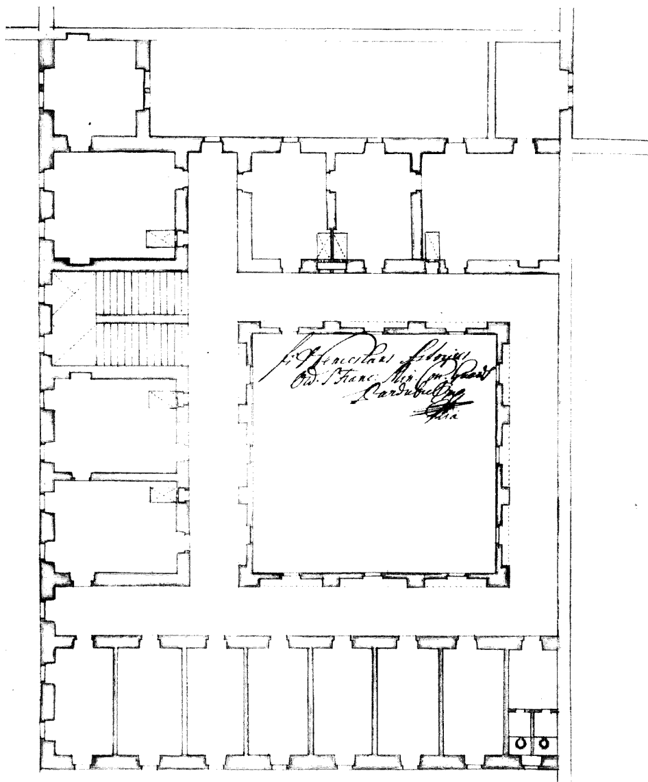
Obr. 3: Plán 1. patra z roku 1695 na stavbu minoritského kláštera v Pardubicích - Giovanni Domenico Canevalle (SÚA, NM, sg. K 2 M 2/4/7). Realizováno 1699 - 1703.
