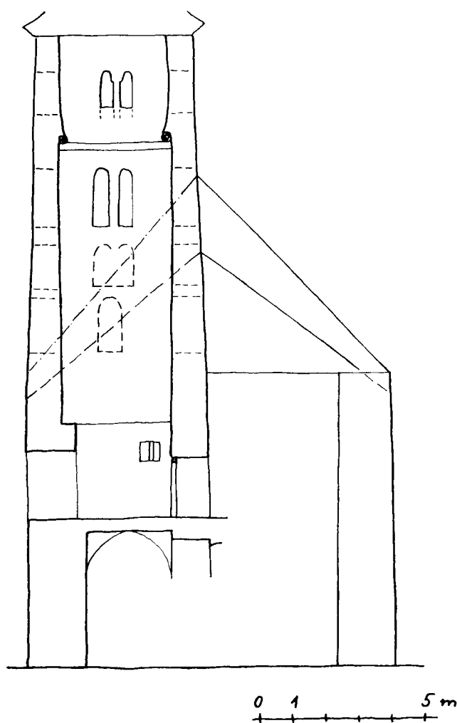
Obr. 3: Řez kostelní věží v pohledu k západu. Částečné pracovní zaměření pískem autor, 1994.
