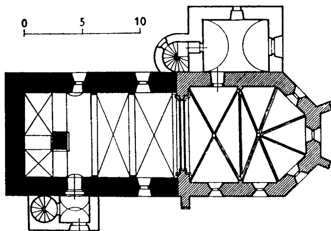
Obr. 2: Půdorys kostela (podle A. Merhautové, Raně středověká architektura v Čechách, Praha 1971, s. 110 (revidováno).
