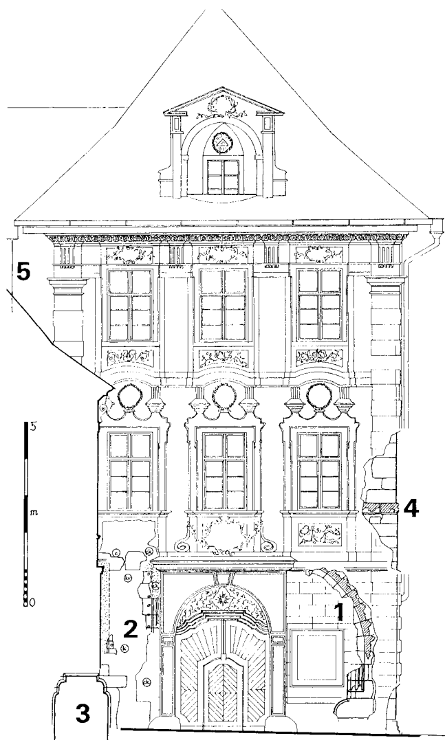
Obr. 2: Praha, dům č. p. 634/I. Náčrty v jižním průčelí. 1 - Zachovaná část ostění portálu, 2 - pozůstatky dvojice obdélných oken přízemí, 3 - portál sklepa, 4 - kordonová římsa, 5 - kvádrová nároží (zdivo vlevo od spáry pozdější). Ostatní označení dle obr. 1. (Zakresleno do zaměření SÚRPMO, doměření náčrtů Jan Sommer, 1994.).
