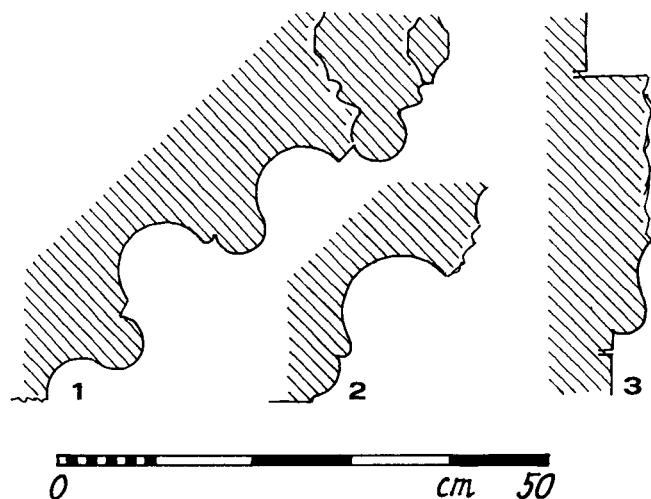
Obr. 8: Praha, dům č. p. 634/I. Detaily architektonického členění zaniklých gotických průčelí. 1 - profilace ostění zrušeného gotického okna ve východní stěně prvního patra, 2 - profilace ostění zrušeného obdélného okna v jižní stěně přízemí, 3 - zachovaná část profilace kordonové římsy. (Zaměření Jan Sommer, 1994).
