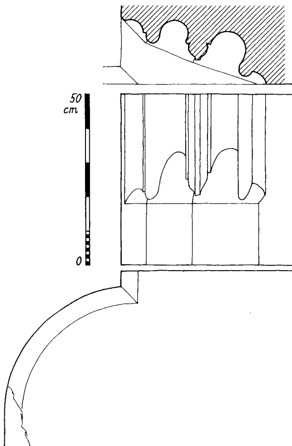
Obr. 6: Praha, dům č. p. 634/I. Profilace ostění zrušeného gotického vstupního portálu a čelní pohled na dolní část ostění. (Zaměření Jan Sommer, 1994.)
