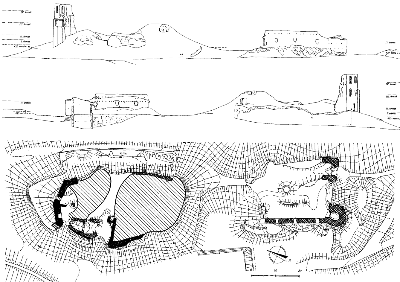
Obr. 2: Cimburk, jihozápadní a severovýchodní pohled na hrad a půdorys ve 2. úrovni se stavebně historickou analýzou: zrněné zdivo gotické, křížkované pozdně gotické, přerušované značeno hypotetické zařazení. (Zpracoval L. Svoboda s použitím zaměření PŮ Pardubice.)
