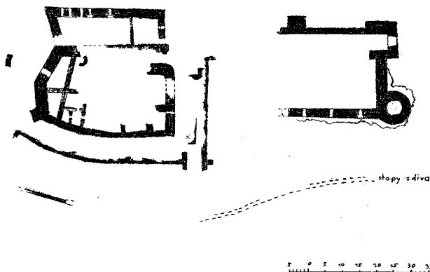
Obr. 8: Cimburk, půdorys hradu údajně z roku 1912 (podle E. Tuče).
