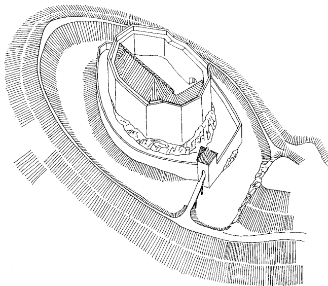
Obr. 4: Cimburk, pokus o rekonstrukci podoby hradu na konci 14. století - kavalirní pohled od jihu. (Kresba L. Svoboda).
