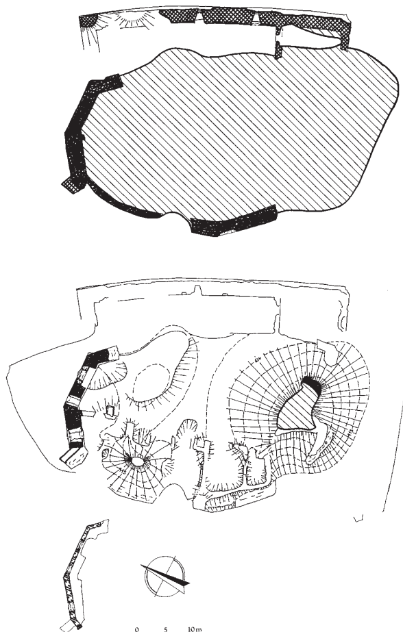
Obr. 3: Cimburk, půdorys (shora) v 1., 3. a 4. úrovni se stavebně historickou analýzou. Legenda jako u obr. 2, šrafovou značeno zdivo renesanční a tečkováním novodobé.
