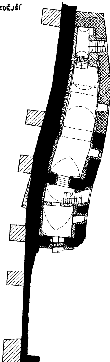
Obr. 9: Analýza sklepů Horního zámku.
