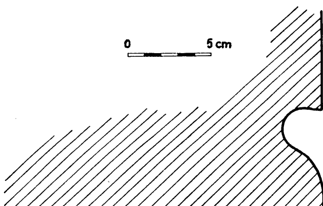
Obr. 17: Půdorys obranného patra „hodinové“ věže štítové zdi a řez gotickým ostěním portálu v patře východní fasády.
