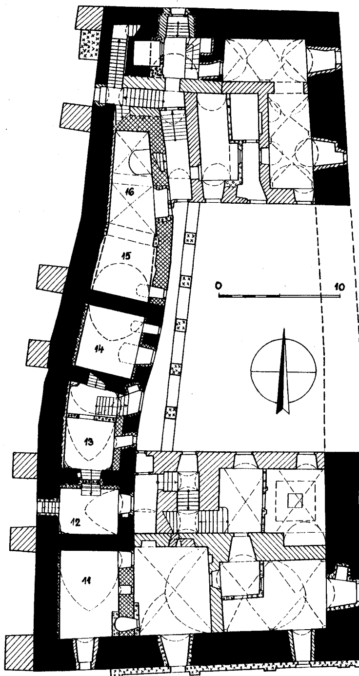
Obr. 10: Analýza přízemí Horního zámku.
