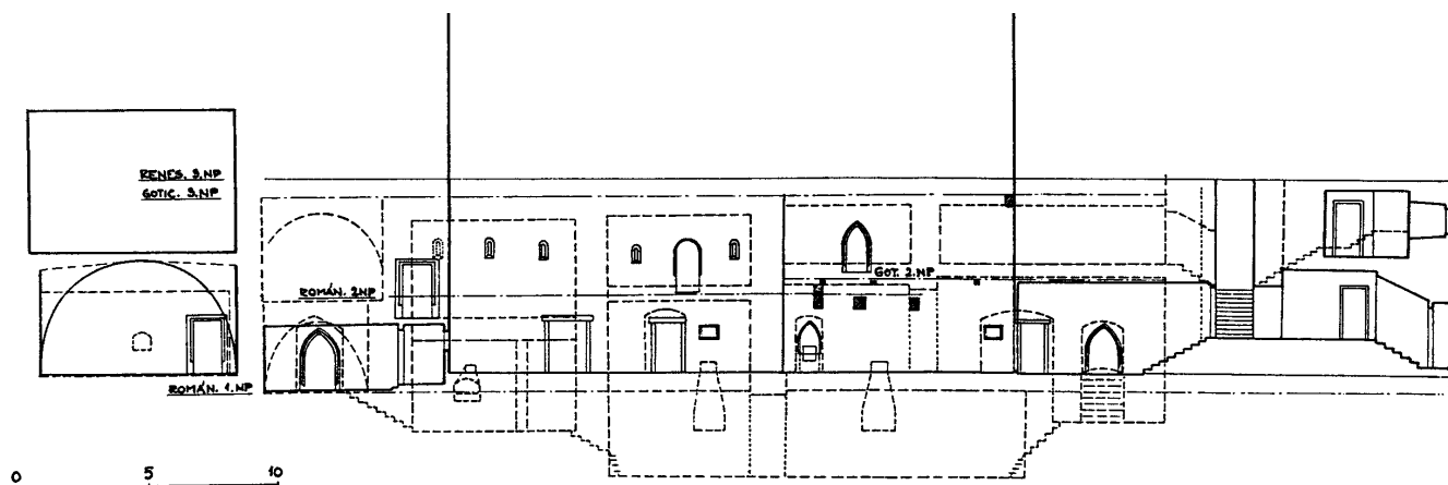
Obr. 13: Řez sever - jih vedený arkádovou chodbou Horního zámku s pohledem k západu.
