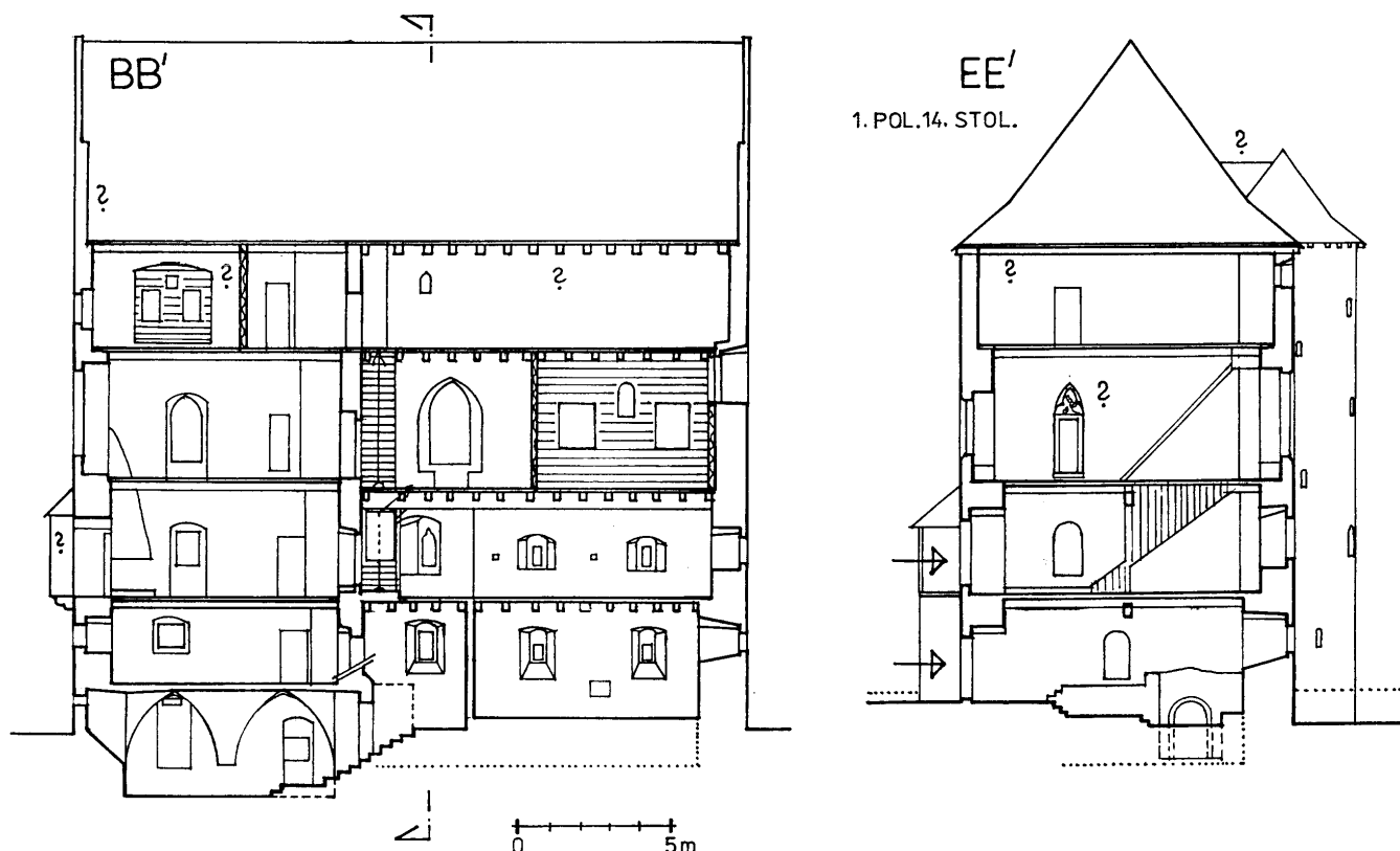
Obr. 20: Rekonstrukční řezy paláce tvrze. Čárkované obrysy jsou mimo rovinu řezu, tečkované úrovně podlah a terénu označují dnešní stav. Poloha stropních trámů je vyznačena schematicky, otazníkem označené konstrukce jsou předpokládány nebo neznámé.
