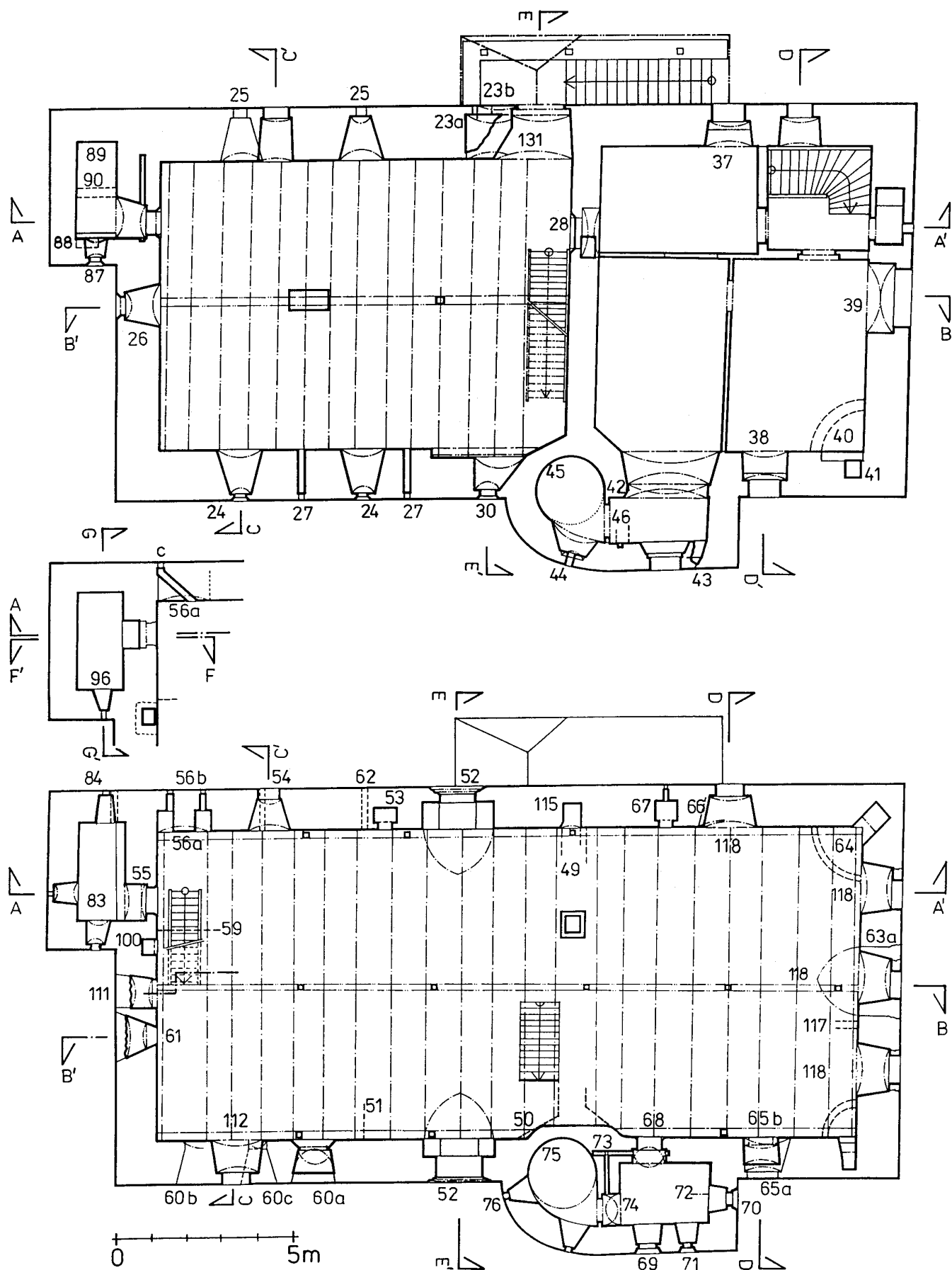
Obr. 4: Půdorysy paláce tvrze s vyznačením náleзовých situací. Nahoře 1. patro, dole 2. patro, uprostřed komůrka nad 2. patrem v záchodovém rizalitu.
