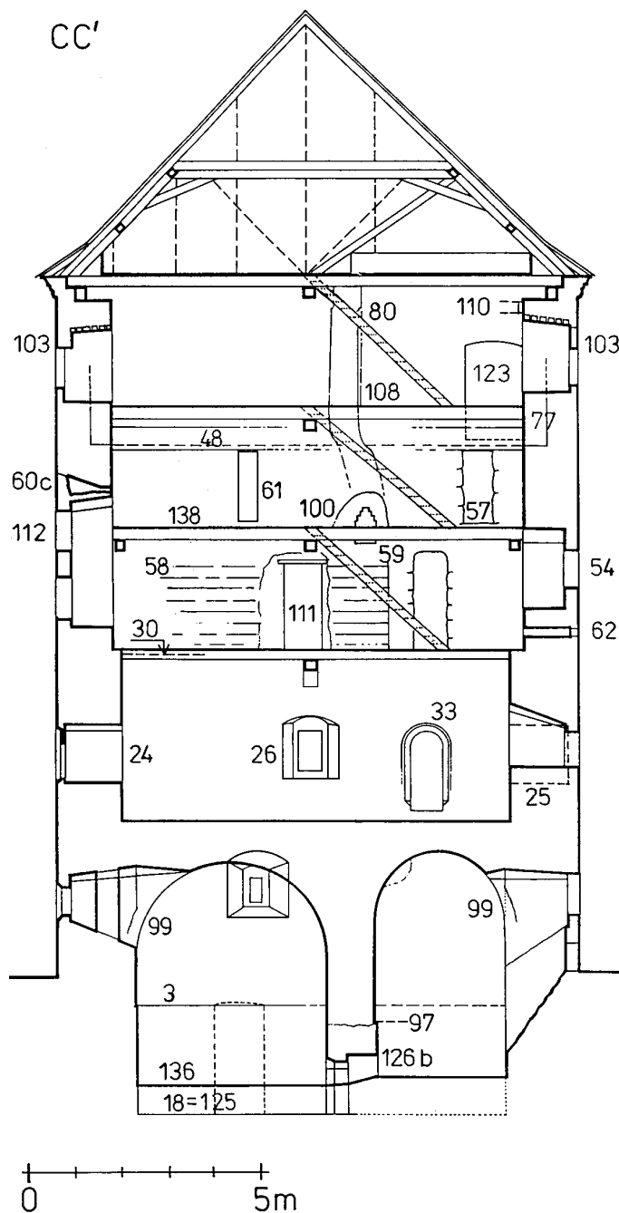
Obr. 13: Příčný řez s pohledem k západu s vyznačením nálezových situací.
