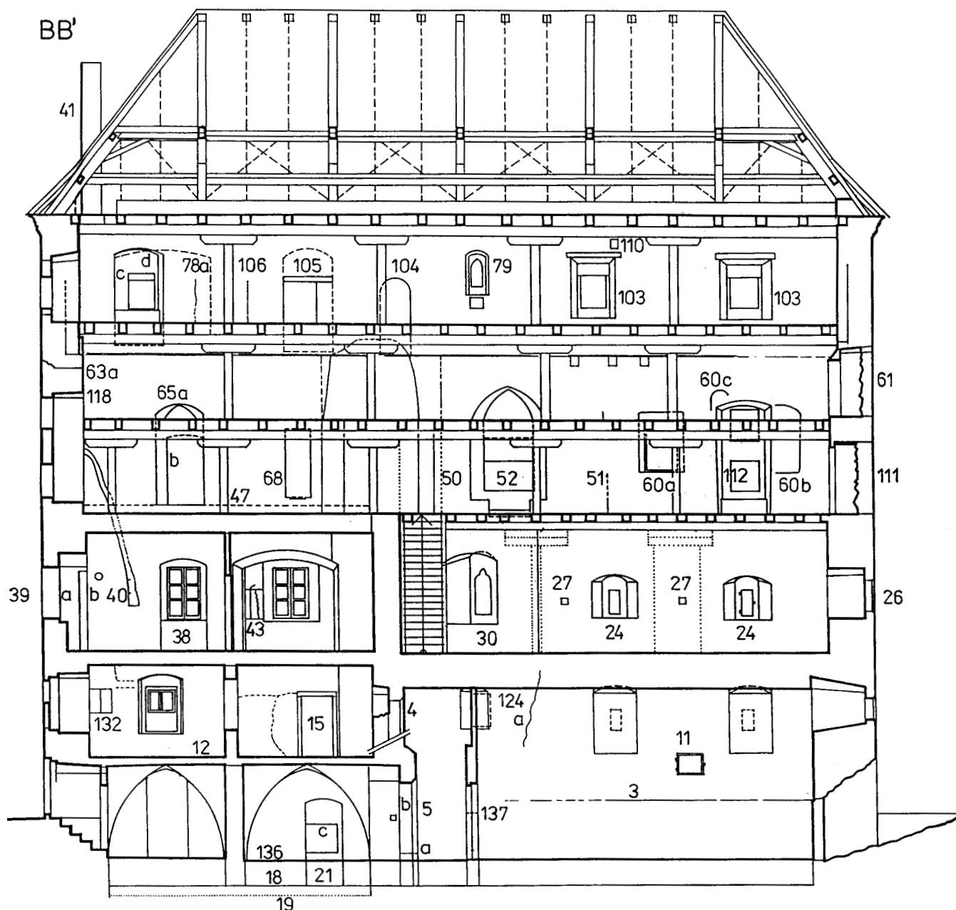
Obr. 12: Podélný řez s pohledem k jihu s vyznačením nálezových situací.
