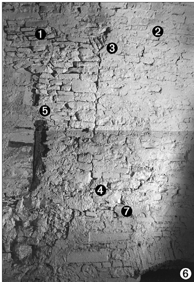
Obr. 21: Podélná střední zeď sklepa, rozdělující západní část půdorysu. Pohled od jihu na situaci mezi novodobým pilířem a východním průřezem, 1 - renesanční zdivo, 2 - zdivo přezděné v baroku, 3 - špaleta a zbytek záklenku renesančního průchodu mezi sklepy, 4 - úroveň renesanční podlahy, 5 - podchycení havárie druhotně použitými kamennými kvádry, 6 - východní průřez mezi sklepy, 7 - podezdění ze smíšeného zdiva s kusy druhotně použitého olišovaného ostění.
