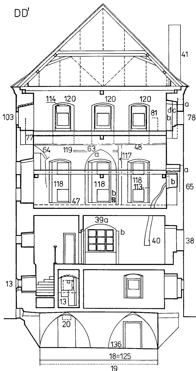
Obr. 14: Příčný řez s pohledem k východu s vyznačením nálezových situací.
