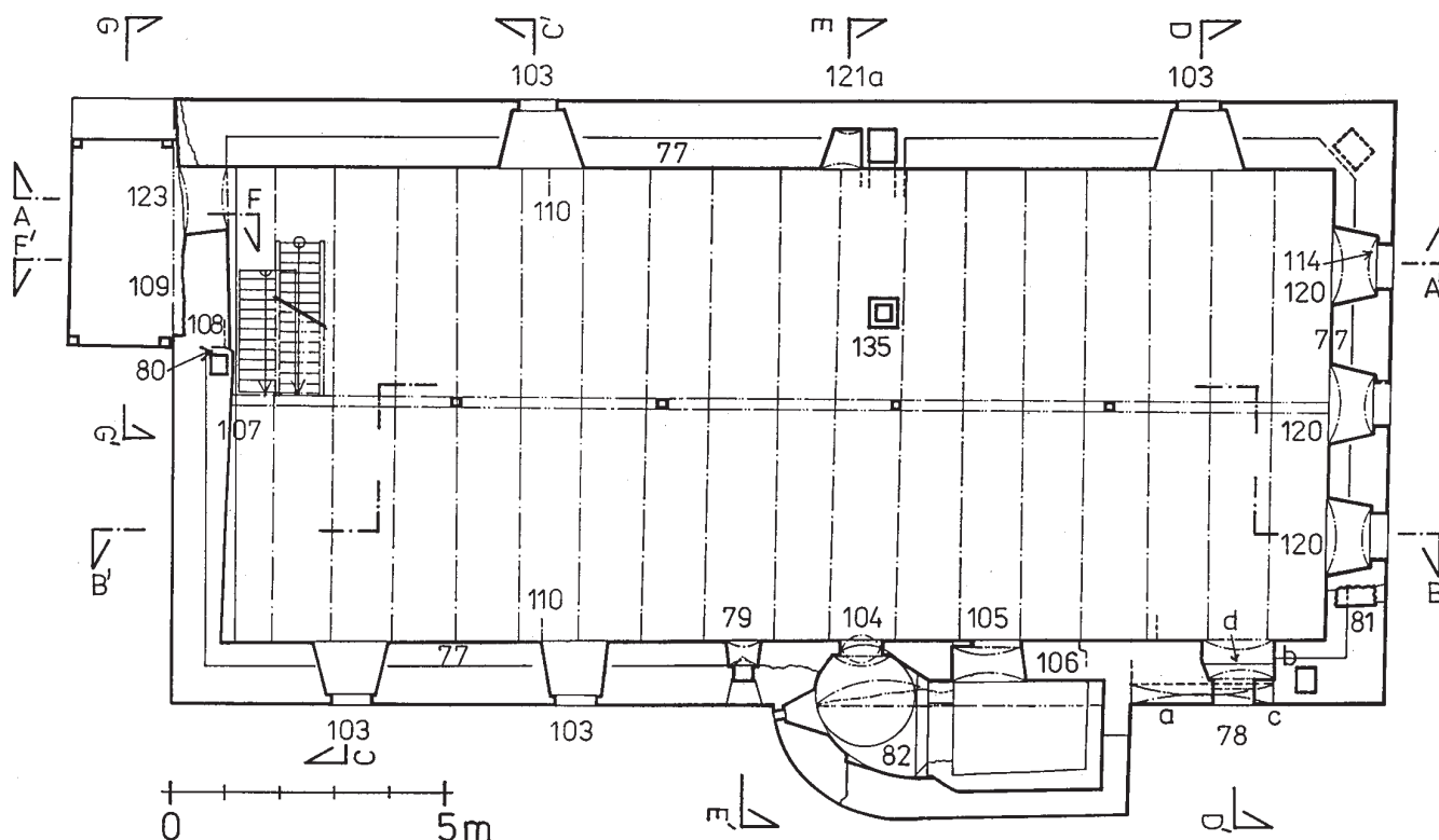
Obr. 5: Půdorys 3. patra paláce tvrže s vyznačením náleзовých situací.
