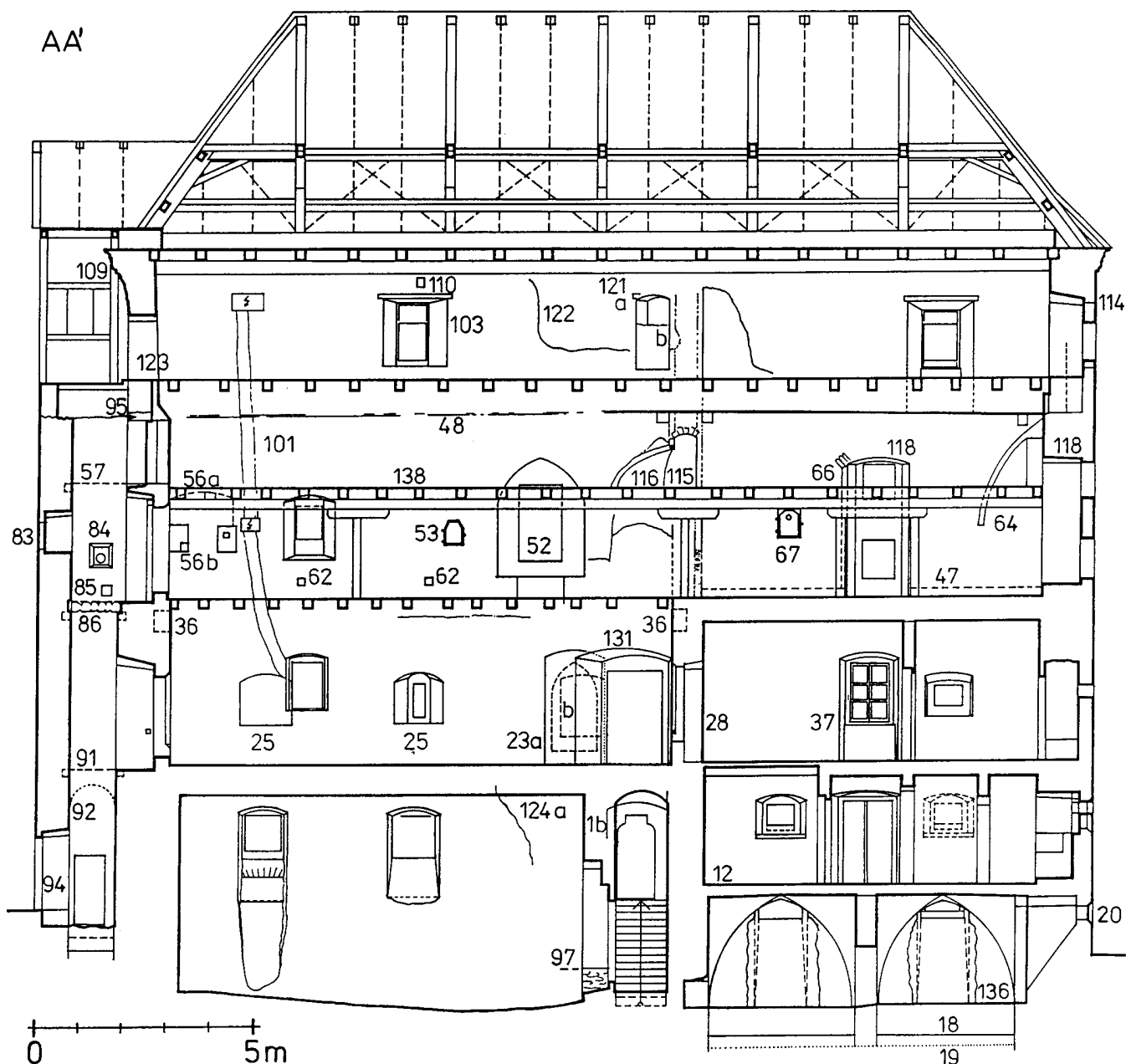
Obr. 11: Podélný řez s pohledem k severu s vyznačením nálezoových situací.
