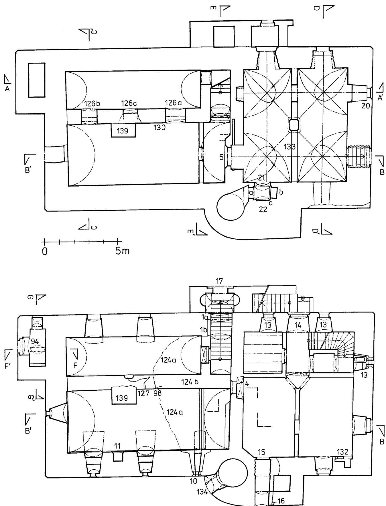
Obr. 3: Půdorys paláce tvrze s vyznačením nálezových situací. Nahoře úroveň sklepa, dole úroveň přízemí. (Autor veškeré plánové dokumentace M. Rykl, 1995.)
