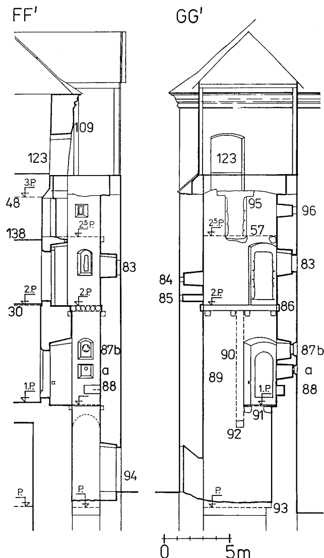
Obr. 16: Řezy záchodovým rizalitem - vlevo s pohledem k jihu, vpravo s pohledem k východu.
