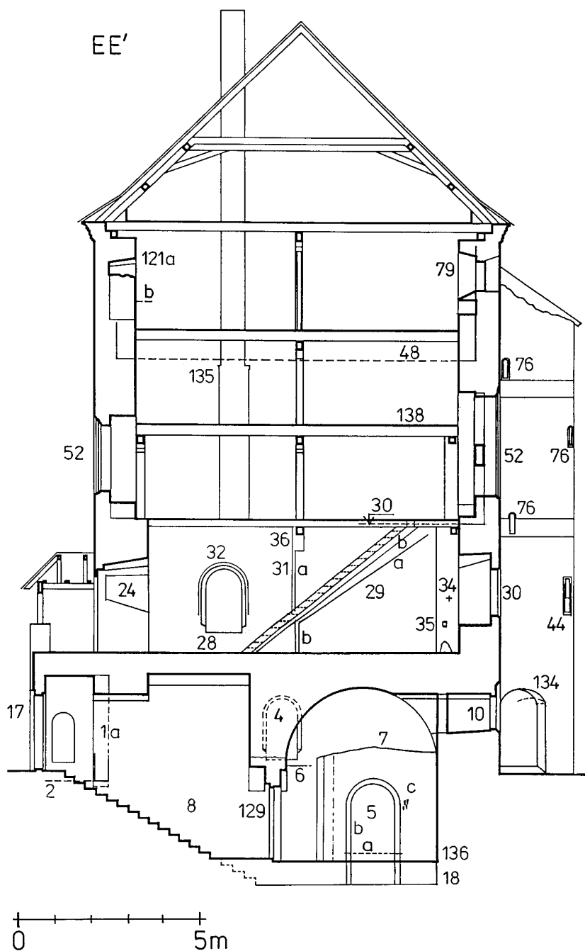
Obr. 15: Příčný řez s pohledem k východu na střední zeď s vyznačením nálezových situací.
