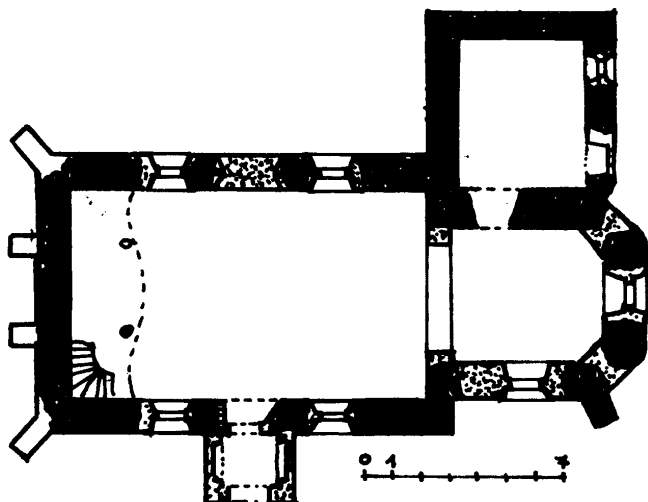
Obr. 1: Skica půdorysu kostela, dle Soupisu památek..., okr. Kladenský s. 136. (půdorys korigován)
