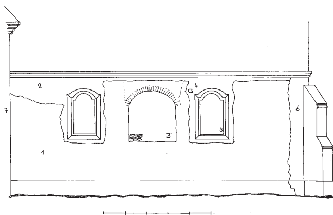
Obr. 3: Pohled na severní průčelí lodi - 1 - gotické zdivo, 2 - barokní zdivo, 3 - zazděné renesanční okno, 4 - fragment arch. článku, 5 - stávající okna, 6 - statické zajištění z roku 1902, 7 - věž. (Zaměření a kresba autor.)
