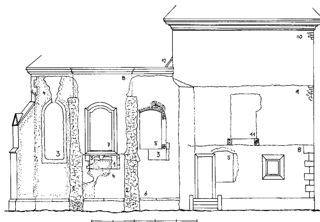
Obr. 2: Pohled na východní průčelí kostela 1 - nejstarší okno presbytáře, 2 - osekané opěrky, 3 - pozdně gotická okna s paspartami, 4 - pozdně gotická omítka, 5 - raně barokní okna, 6 - raně barokní omítka, 7 - stávající okno z roku 1777, 8 - zdivo sakristie, 9 - první a 10 - druhá fáze zdiva věže, 11 - vstup do zvonice, 12 - námětky původní dřevěné zvonice. (Zaměření a kresba autor.)
