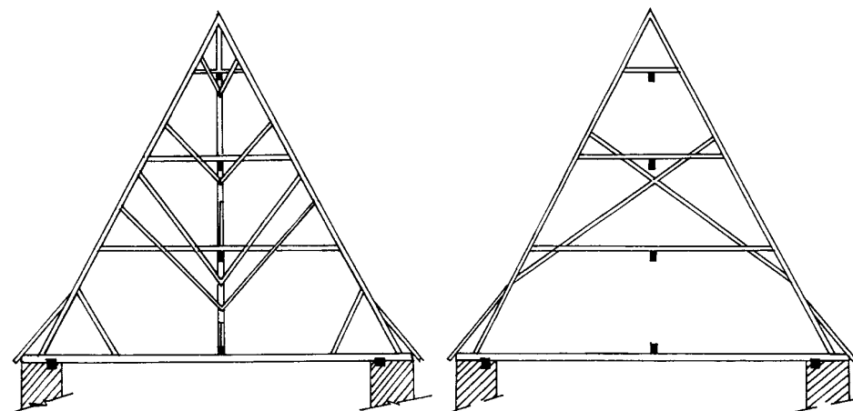
Obr. 4: Krov nad lodí - plná a prázdná vazba a podélný řez.
