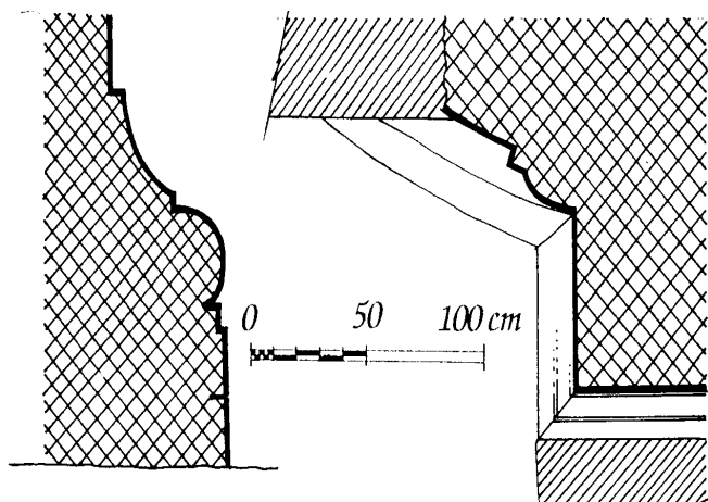
Obr. 2: Profil románské soklové římsy.
