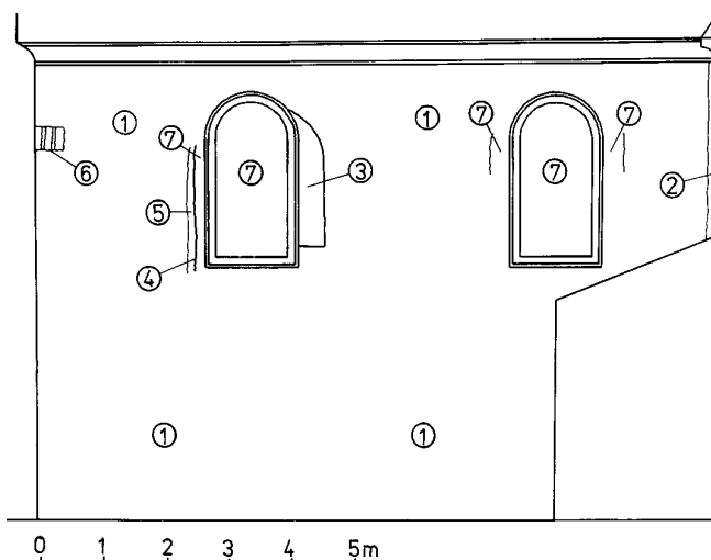
Obr. 5: Kostel Pozdvížení sv. Kříže v Pyšelicích, jižní stěna lodi, nálezková situace po sejmutí vrchních vrstev omítek. 1 - gotické zdivo, 2 - barokní zdivo, 3 - gotický okenní otvor, 4 - hrana levé špalety pozdně gotického okenního otvoru, 5 - cihelné zdivo, 6 - druhotně zazděný žulový clánek, 7 - okenní otvory z romantické přestavby s přilehlým zdivem. (Zakreslil P. Kroupa.)
