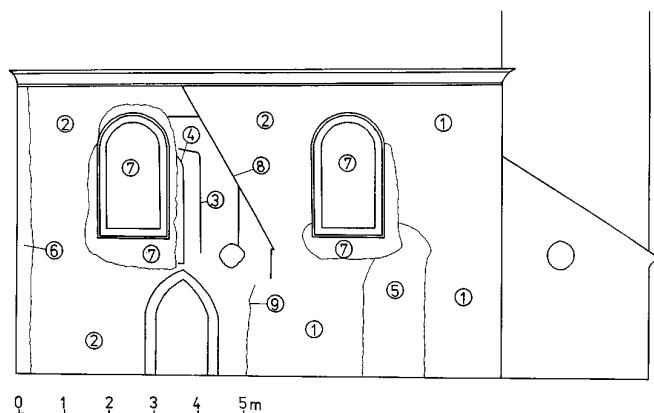
Obr. 2: Kostel Pozdvížení sv. Kříže v Pyšelic, severní stěna lodi, nálezořová situace po sejmutí vrchních vrstev omítek. 1 - románské zdivo, 2 - gotické zdivo, 3 - špaletový otvor, 4 - okenní otvor, 5 - odkrytý (pozděně románský) vstup, 6 - barokní zdivo, 7 - okenní otvory z romantické přestavby s přilehlým zdivem, 8 - otisk gotické přístavby, 9 - předpokládané rozhraní románského a gotického zdiva. (Zakreslil P. Kroupa.)
