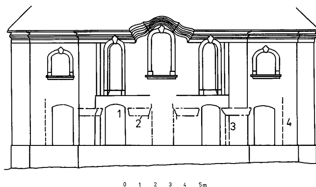
Obr. 7: Kostel Pozdvížení sv. Kříže v Pyšelicích, skica východního průčelí. 1 - zazděné průchody, 2 - osekane výběhy klenby, 3 - čtvrtpilířky, 4 - odbourané výběhy zdi. (Zakreslil J. Žizka.)
