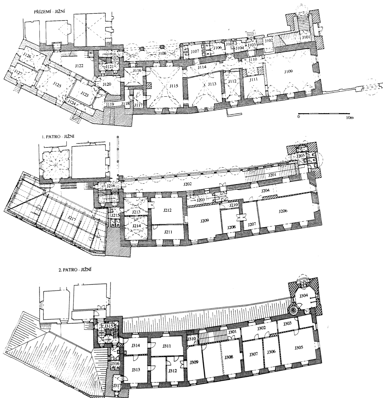
Obr. 5: Púdorys prízemí, 1. a 2. patra jižního křídla zámku. Označení zdiva: křížkovaně šikmo - 1. renesanční fáze (40. léta 16. stol.), křížkovaně kolmo - 2. renesanční fáze (2. pol. 16. stol.), šrafovaně - 1. barokní fáze (2. pol. 17. stol.), šrafovaně přerušovanou čarou - 2. barokní fáze (2. čtvrtina 18. stol.), šrafovaně dvojitou čarou 1. fáze novogotických úprav (1800 - 1820), tečkovaně - 2. fáze novogotických úprav (2. pol. 19. stol.), bíle - 20. století.
