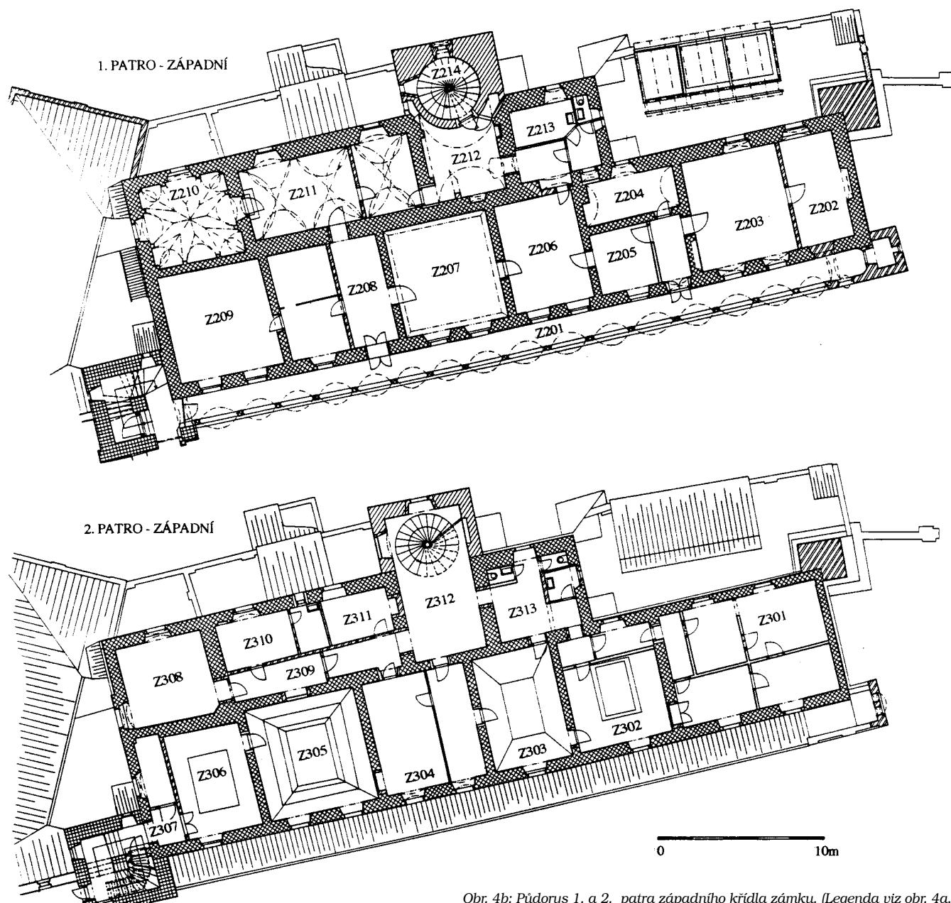
Obr. 4b: Půdorys 1. a 2. patra západního křídla zámku. (Legenda viz obr. 4a.)
