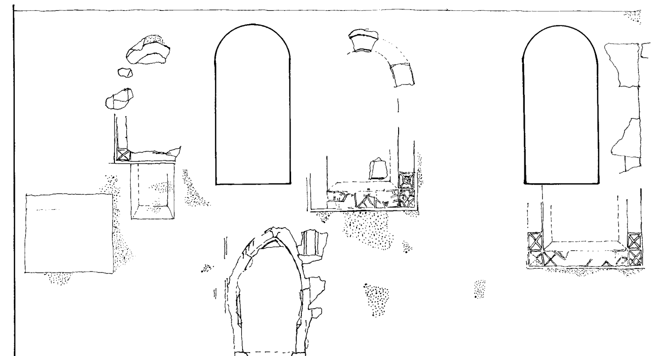
Obr. 8: Křivsoudov - kostel Narození Panny Marie - jižní průčelí lodě. Podrobné zakreslení nálezů pozdně gotické fasády. Průzkum, zaměření a kresba autor.
