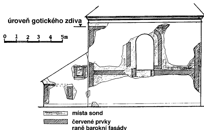
Obr. 7: Křivsoudov - kostel Narození Panny Marie - východní průčelí presbyteria a sakristie. Zaměření a vyhodnocení průzkumu Ing. J. Žižka, kreslil autor.
