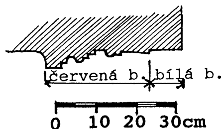
Obr. 18: Křivsoudov - kostel Narození Panny Marie. Profilace vrcholné barokní šambrány z jižního průčelí presbyteria. Zaměřil Ing. J. Žižka, kresba autor.
