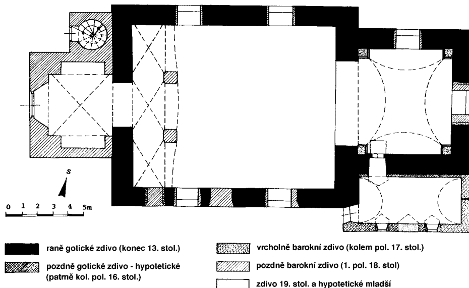
Obr. 3: Krivsoudov - kostel Narození Panny Marie. Zaměření a vyhodnocení po průzkumu jižního a východního průčelí autor.
