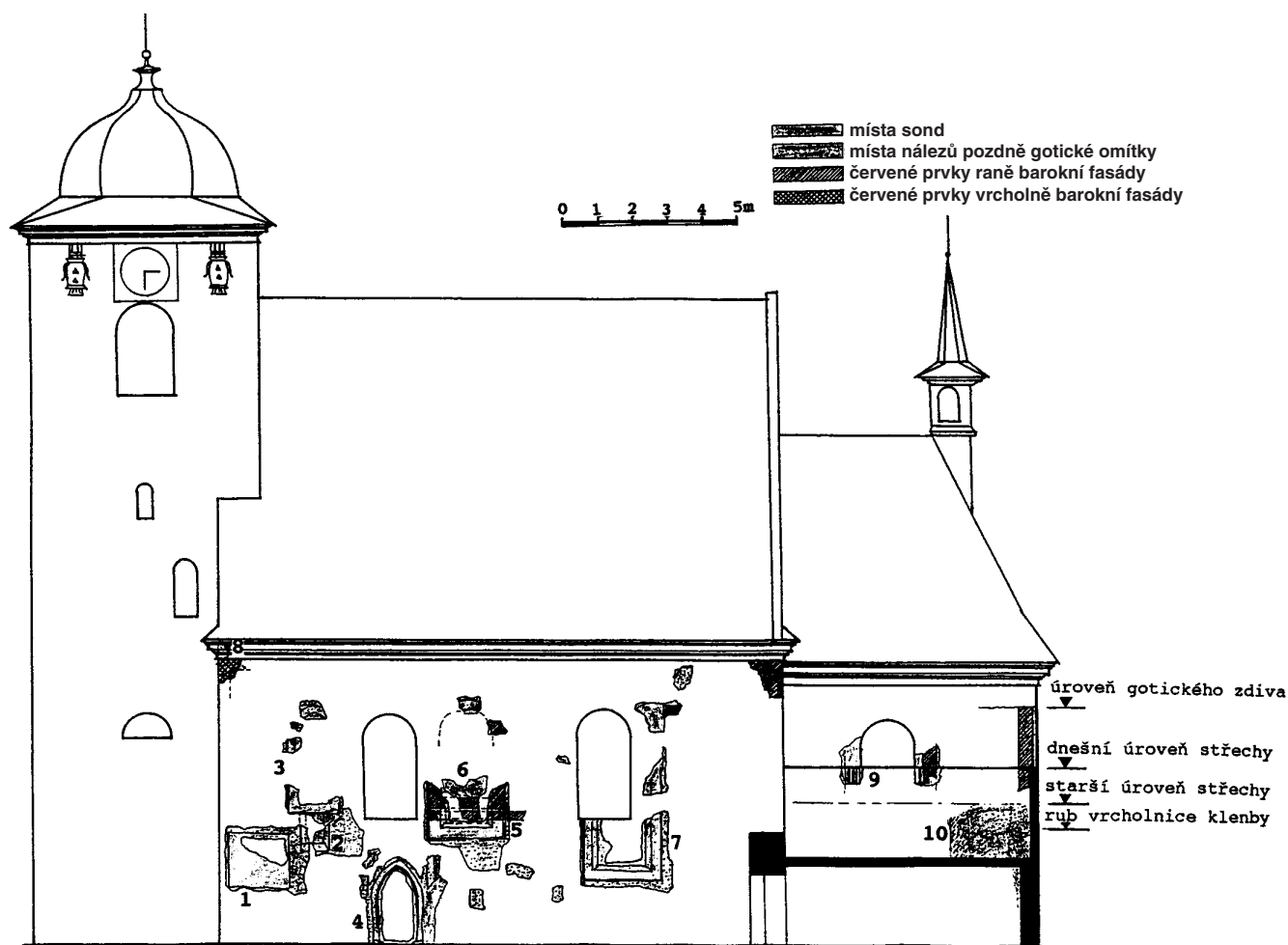
Obr. 6: Krivsoudov - kostel Narození Panny Marie, jižní průčelí lodi a presbyteria (s řezem sakristií a pohledem na jižní stěnu presbyteria na půdě sakristie). Zaměření a vyhodnocení průzkumu autor a Ing. J. Žižka, kreslil autor.
