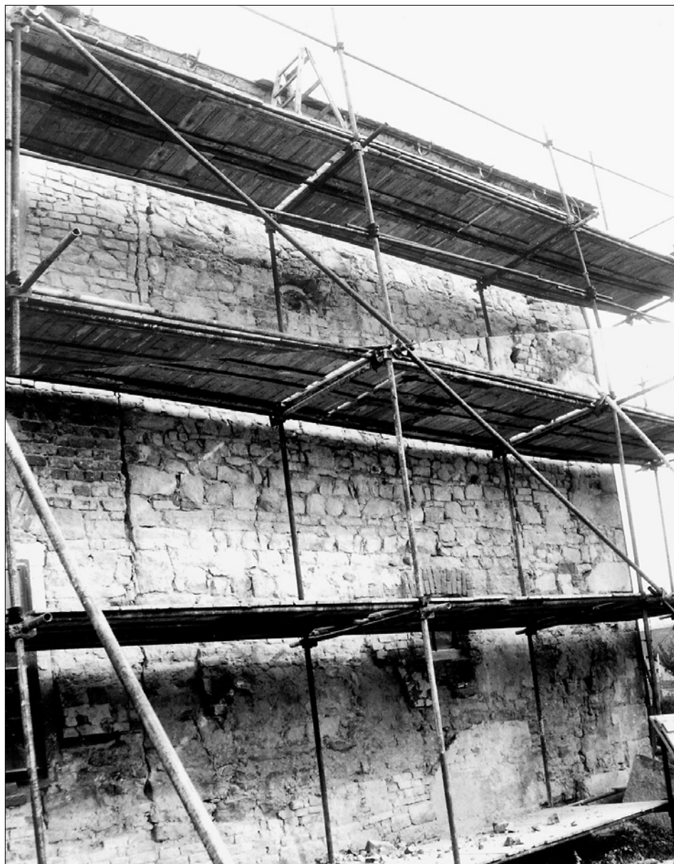
Obr. 2: Jižní nároží západního průčelí se spárou oddělující tvrz.
