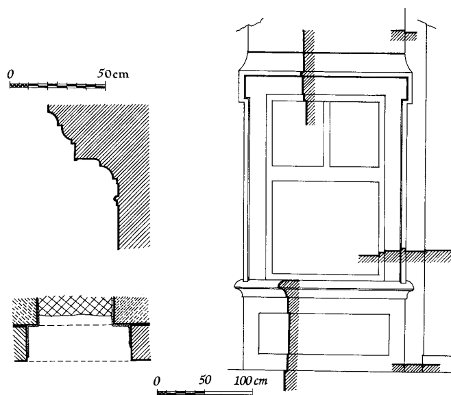
Obr. 3: Profilace korunní římsy, půdorys okénka tvrze a barokní okno.
