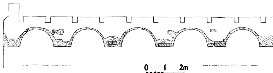
Obr. 2: Nákres vrchní části severního průčelí kostela. Tečkovaně vyznačen rozsah přisekaného zdiva, šrafováním pletování, černě nálezy dřeva, čerchovanou čarou úroveň vrcholů okenních špalet. (L. Svoboda).
