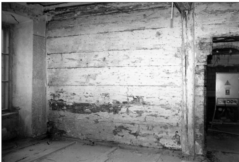
Obr. 9: Znojmo, dům čp. 15. Roubená obytná místnost v přízemí (místnost č. 105), východní stěna, levá část (viz obr. 7). (Foto autoři.)
