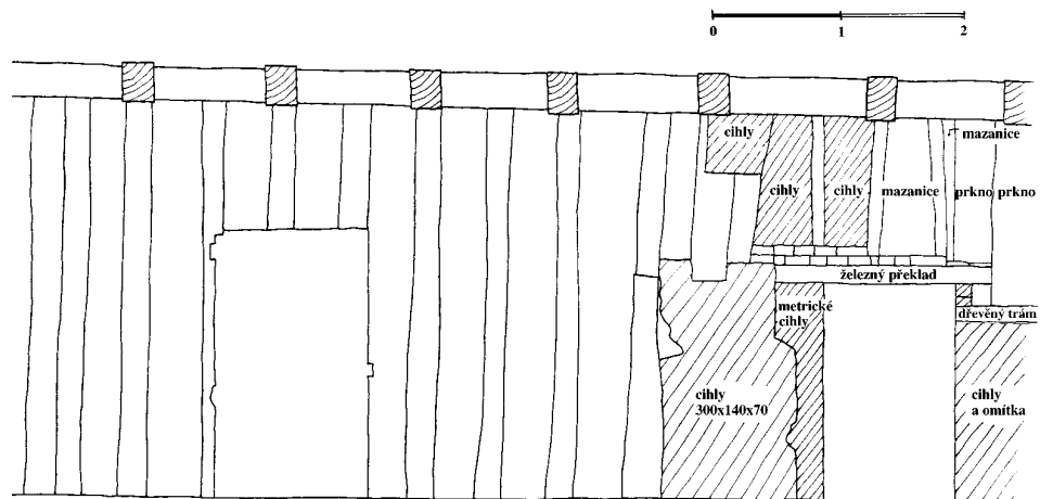
Obr. 12: Znojmo, dům čp. 15. Místnost č. 205 - východní stěna. (Kresba autoři, 1996.)
