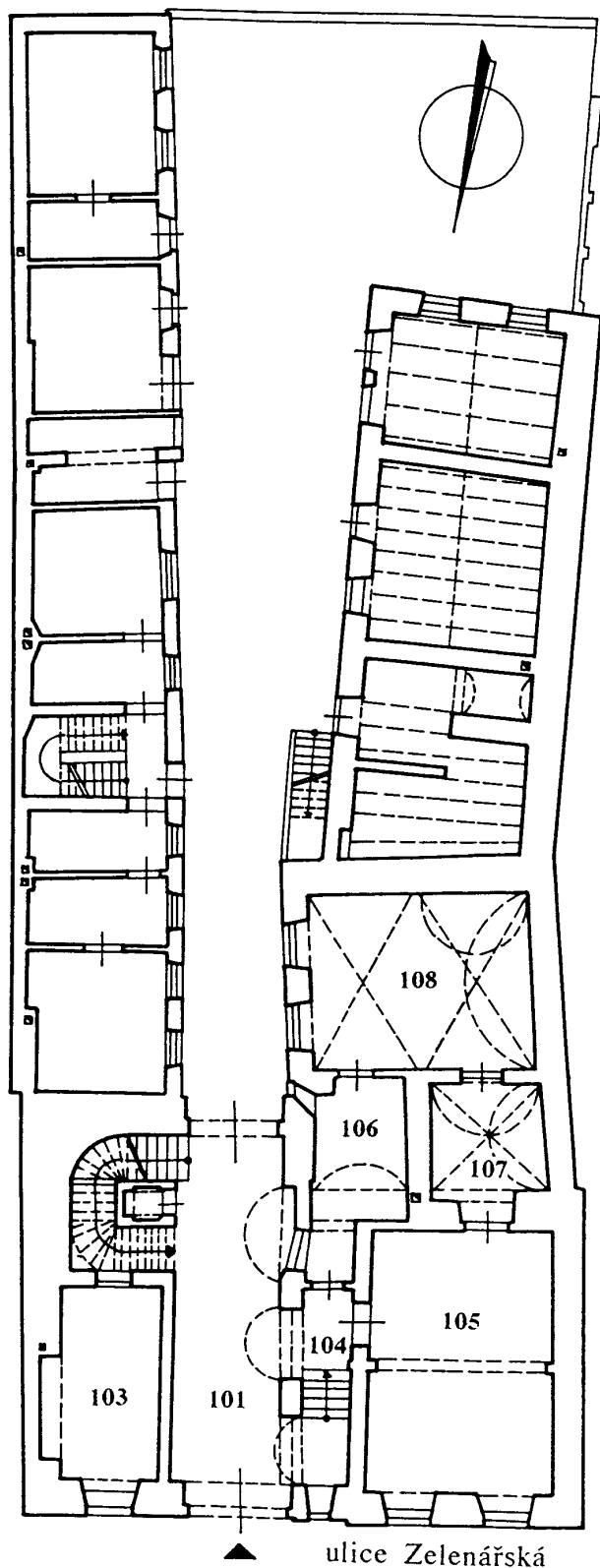
Obr. 2: Znojmo, dům čp. 15. Půdorysné schéma celého objektu (včetně zbouraných dvorních křídel). (Kresba D. Černoušková, 1996.)
