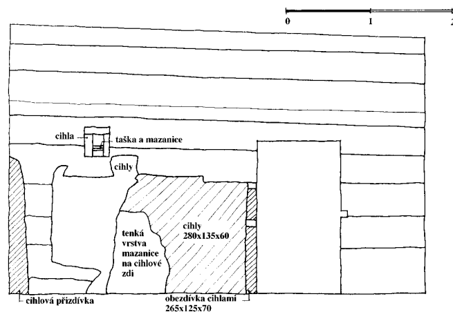
Obr. 6: Znojmo, dům čp. 15. Místnost č. 105 - jižní stěna.
