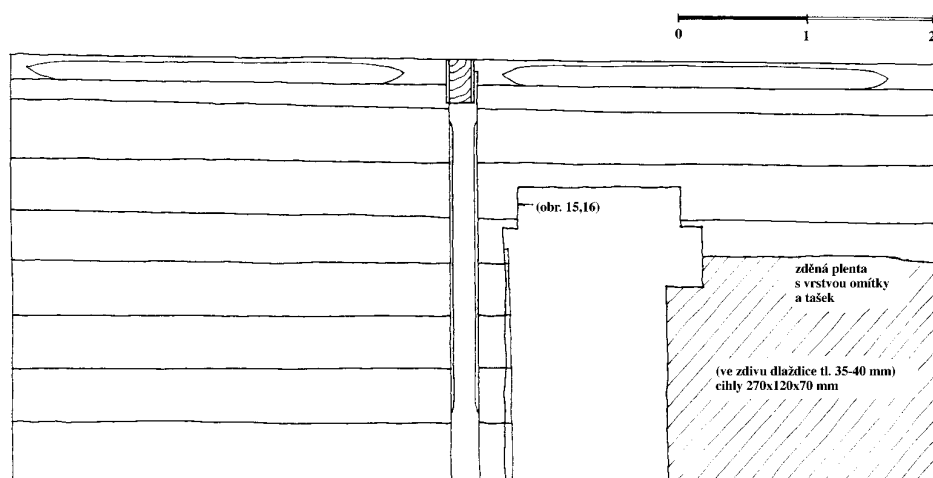
Obr. 7: Znojmo, dům čp. 15. Místnost č. 105 - východní stěna.
