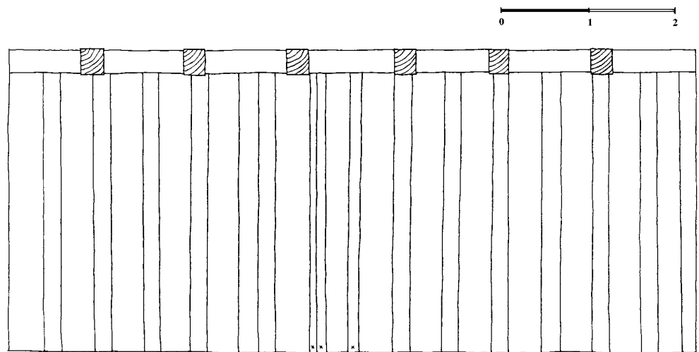
Obr. 13: Znojmo, dům čp. 15. Místnost č. 205 - západní stěna. (Kresba autoři, 1996.) x - nově vyměněné desky.
