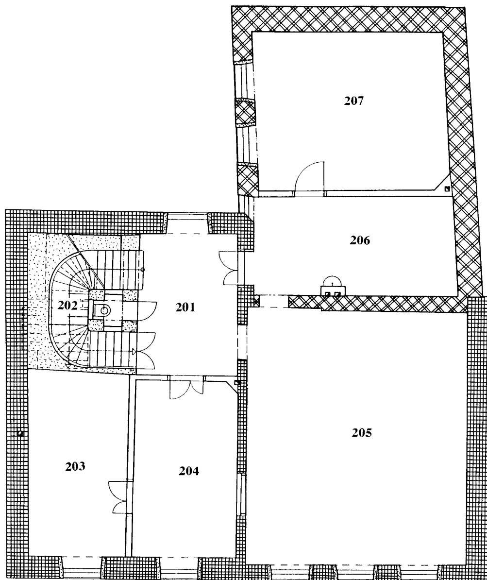
Obr. 5: Znojmo, dům čp. 15. Patro. (Kresba autoři, 1996.)
