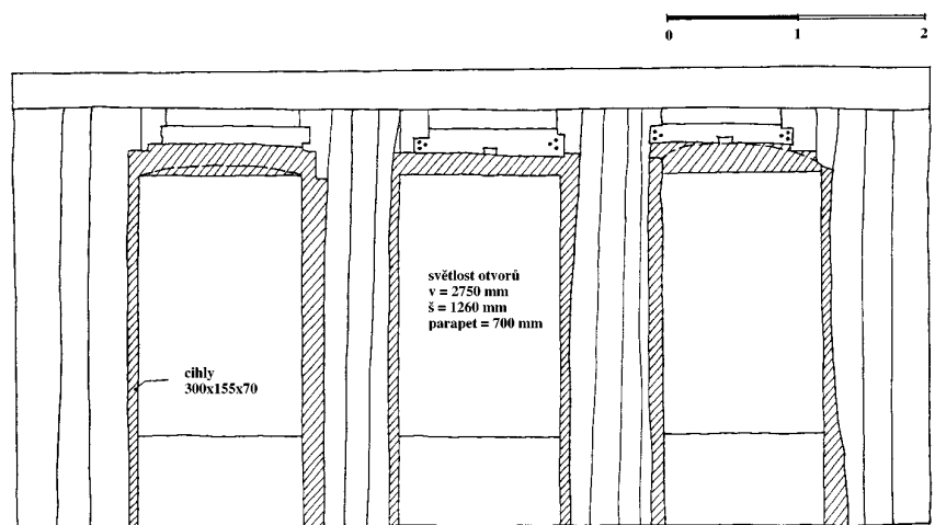
Obr. 14: Znojmo, dům čp. 15. Místnost č. 205 - severní stěna. (Kresba autoři, 1996.)
