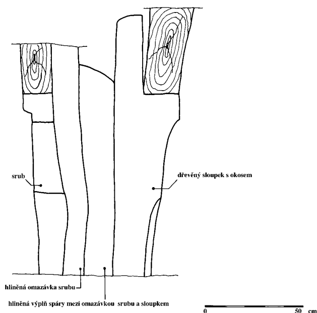
Obr. 19: Znojmo, dům čp. 15. Místnost č. 105 - řez horní částí východní zdi. (Kresba autoři, 1996.)
