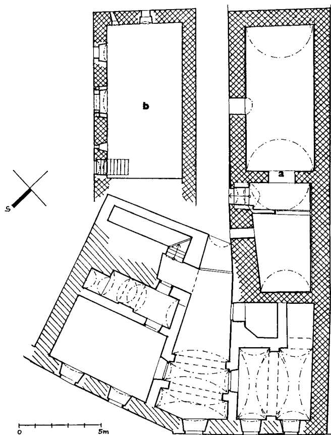
Obr. 12: Touškov, čp. 44, půdorys suterénu domu a patra špýcharu, křížkovaně zdivo pozdně gotické, šrafované předpokládané pozdně gotické zdivo.
