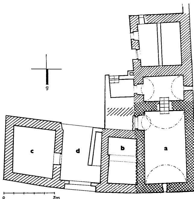
Obr. 11: Touškov, čp. 42, půdorys sklepů s vyznačením celkové dispozice, křížkovane zdivo pozdně gotické, šrafovane předpokládané pozdně gotické zdivo.
