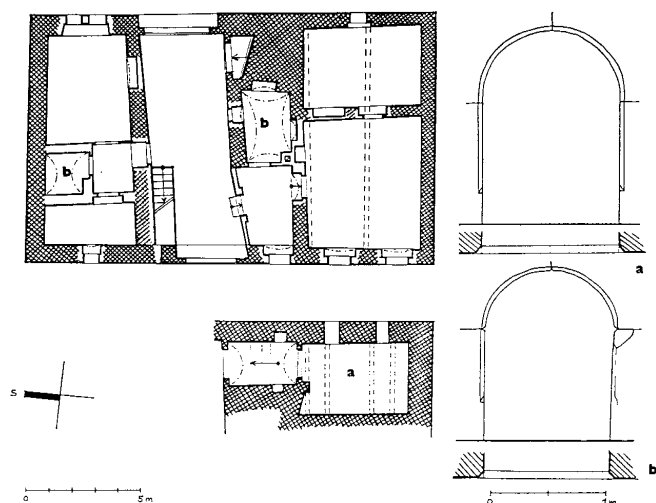
Obr. 4: Touškov, čp. 52, půdorysy přízemí a sklepa s analýzou stavebního vývoje, křížkovaně zdivo goticko - renesanční, šrafované barokní, tečkované klasicistní, ostatní mladší. (Všechna zaměření a kresby autor, 1996.)
