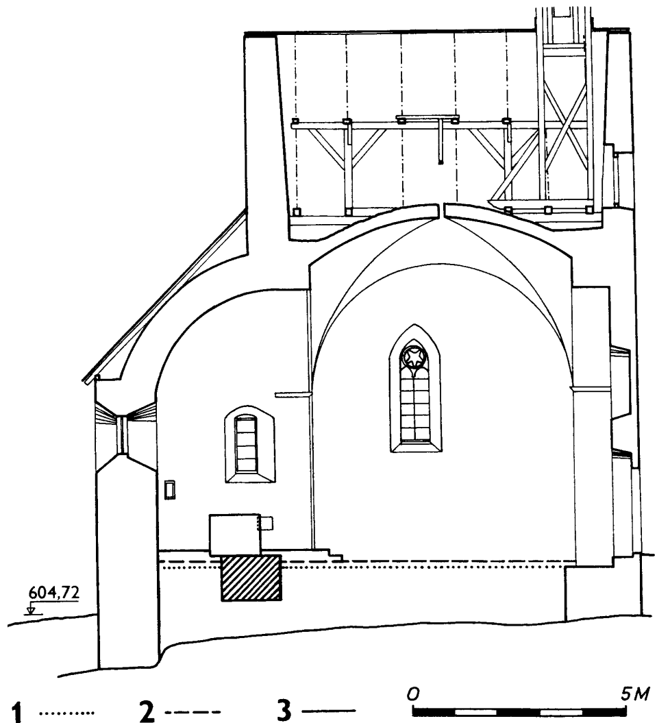
Obr. 5: Pomezí, řez chórem a apsidou kostela. Podle J. Muka a doplněno.
