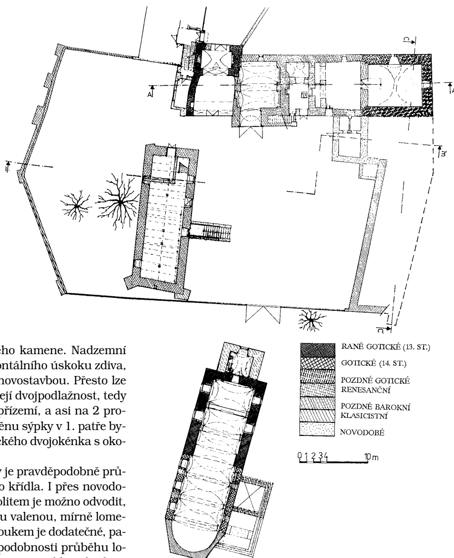
Obr. 12: Horní Kounice - kostel sv. Michala a hospodářský dvůr - 1. patro/přízemí, stavebně historická analýza. (Zaměření a průzkum V. Jesenský.)
