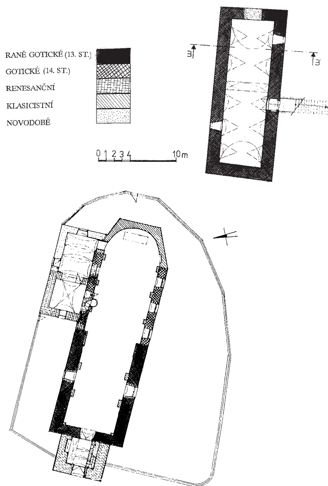
Obr. 13: Horní Kounice - kostel sv. Michala a hospodářský dvůr - přízemí/suterén, stavebně historická analýza. (Zaměření a průzkum V. Jesenský.)
