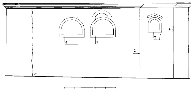
Obr. 1: Brandýs nad Labem, kostel sv. Petra. Pohled na jižní průčelí. 1 - zániklá okna lodi; 2 - horní úroveň kvádřové armatury nároží; 3 - zazděná část otvoru pod oknem presbytáře; 4 - osekaný kvádr na nároží (zbytek výzdoby ?); 5 - vertikální trhlina. (Zaměření a kresba autor, 1996.)
