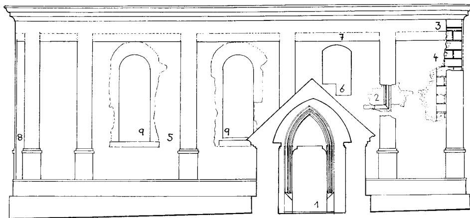
Obr. 2: Pohled na jižní průčelí kostela sv. Jakuba Větš. v Minicích. 1 - portál v předsíní do lodi, 2 - fragment gotického okna, 3 - římsový profil, 4 - omítka s malovaným kvádřovaným pásem, 5 - předpokládaná poloha jihozápadního nároží lodi, 6 - zazděné barokní okno, 7 - původní barokní lesenový pás, 8 - druhotně použité gotické kvádry, 9 - neorenesanční okna. (Zaměření autoři, 1995.)
