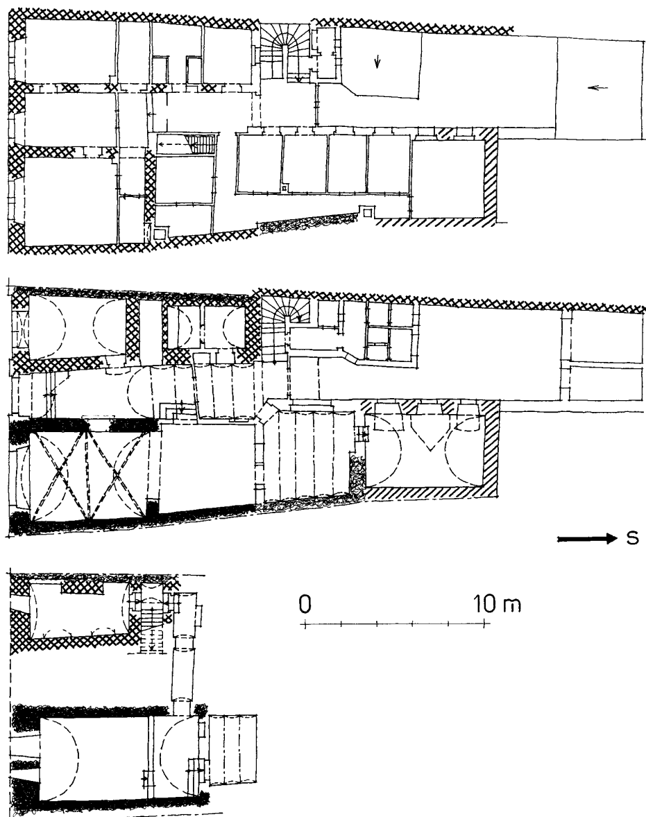
Obr. 2: Tachov čp. 59, zdola sklepy, přízemí, první patro. Černě - konstrukce pozdně gotické, respektive goticko renesanční (zrněně určené hypoteticky), křížem šrafované - pravděpodobně renesanční, šrafované - pravděpodobně barokní, bíle - mladší a neurčené. (Zaměření a kresba autor, 1996.)
