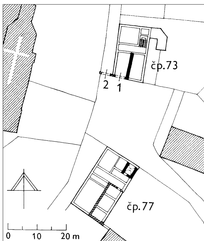
Obr. 1: Situace dle katastrální mapy z r. 1842 s vyznačením dochovaných nebo doložených konstrukcí. (Zaměření domu čp. 77/II s nálezy dle J. Žižky, 1983) 1 - pozdně gotická brána; 2 - renesanční brána; černě - pravděpodobně pozdně gotické zdívo; hustě šrafované - renesanční zdívo.
