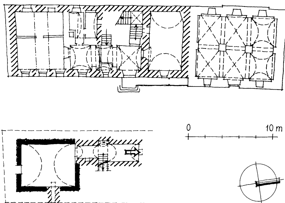
Obr. 1: Bor u Tachova, fara, půdorys sklepů a přízemí. Místo nálezu označeno šipkou. Předpokládané konstrukce gotické - černě, goticko renesanční - šrafovaně. (Kresba J. Anderle, 1996.)
