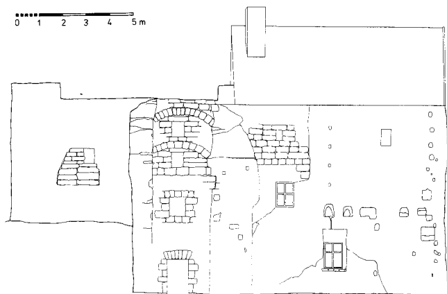
Obr. 2: Čp. 68 k. ú. Sosnová, pohled na severní průčelí. Zaměření K. Podroužek, P. Macháček, 1993.)
