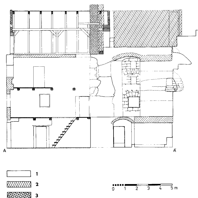
Obr. 6: Čp. 68 k. ú. Sosnová, řez A : A, grafické vyjádření viz obr. 3. Změřené K. Podroužek, P. Macháčková, 1993.)
