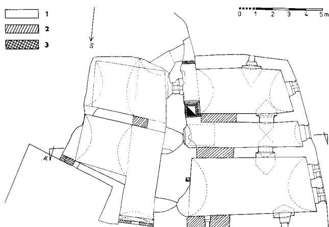
Obr. 5: Čp. 68 k. ú. Sosnová, půdorys 2. patra, grafické vyjádření viz obr. 3. (Zaměření K. Podroužek, P. Macháček, 1993.)
