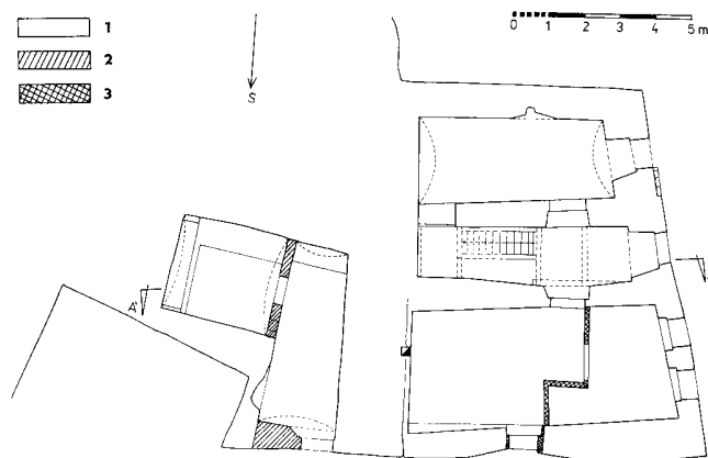
Obr. 3: Čp. 68 k. ú. Sosnová, půdorys přízemí, 1 - zdivo tvořeno skalní stěnou, 2 - zdivo z pískovcových kvádrů, 3 - cihlové zdivo. (Zaměření K. Podroužek, P. Macháček, 1993.)
