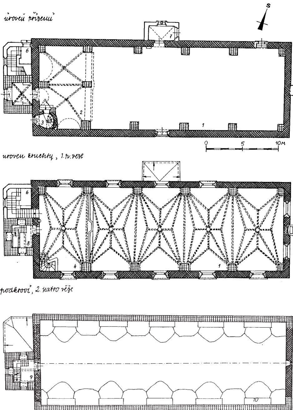
Obr. 4: Strakonice, kostel sv. Markéty, stavebně historický průzkum. Půdorys v úrovni přízemí, kruchtí a podkroví. Husté šikmé mřížky značí zdivo gotické, mřížky kolmé ke konstrukci - renesanční, mladší zdivo ponecháno bílé.
