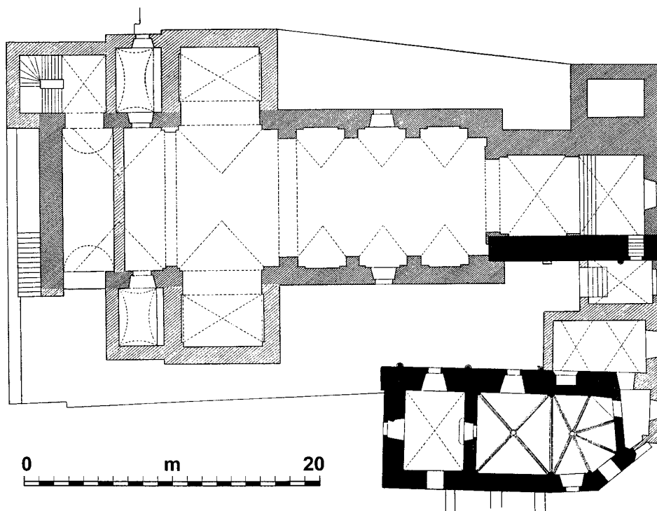
Obr. 2: Písek, kostel Povýšení sv. Kříže. Půdorys kostela a kaple - součásti domu čp. 122 (podle Soupisu památek, cit. v pozn. 1).
