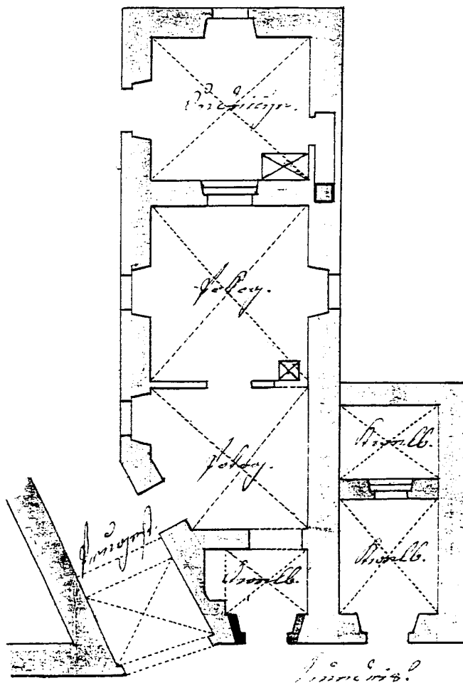
Obr. 16: Písek, kostel Povýšení sv. Kříže. Plán jižní boční kaple jako části domu čp. 122 po přestavbě na byty, datovaný do roku 1822 (Archiv písecký v Mirovicích).
