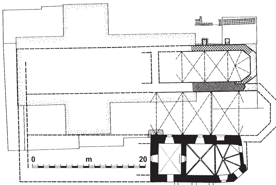
Obr. 13: Písek, kostel Povýšení sv. Kříže. Rekonstrukce půdorysu kostela před zničením gotické stavby na počátku 15. století. Černě je vyznačena jižní boční kaple, zakreslená podle půdorysu kostela v Soupisu památek (cit. v pozn. 1), hustším šikmým křížkováním zdivo ze 13. století obsažené v jižní zdi nynější vstupní prostory kostela, řídkým šikmým křížkováním dochované úseky zdiva severní kaple ze 14. století, šikmá šrafu- ra značí části zdiva doložené archeologickým průzkumem, přerušovaná šikmá šrafura označuje archeologicky doložené gotické základové zdivo, vodorovným křížkováním je označeno pozdně gotické či renesanční zdivo severně od kostela, doložené archeologickým a stavebním průzkumem. Tečkováním je zvýrazněn obrys nynějšího barokního kostela. Silné obrysové linie označují průběh gotických zdí, které lze pokládat za nepochybné, přerušovanou čarou jsou zakresleny hypotetické části dispozice gotického kostela (kresba Jan Sommer, 1997).
