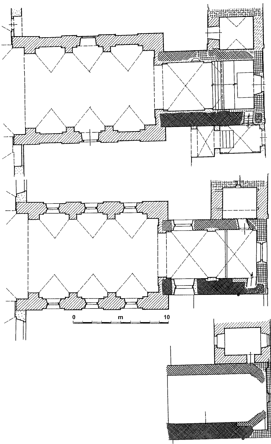
Obr. 19: Písek, kostel Povýšení sv. Kříže. Půdorys kostela a kaple. Nahoře půdorys východní části kostela v úrovni přízemí s vyznačením stáří jednotlivých konstrukcí (kresba s částečným využitím půdorysu kostela z roku 1902, doplnil Jan Sommer).
