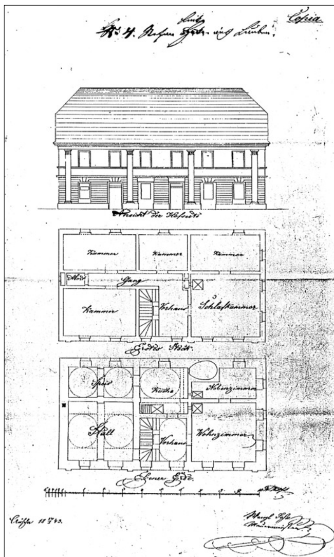
Obr. 10: Loubí, projekt novostavby domu menší usedlosti čp. 4: No 4 Stefan Linke aus Lauben, Copia, Ústěk 14. 5. 1843, zednický mistr Wenzl Jahn, grafické měřítko vídeňské sáhy, půdorys přízemí a prvního patra, pohled (SO-bA Děčín, Vs Česká Lípa, kt. 252, plán 4). Na dochovaném objektu je zajímavé provedení velmi plochých plackových klenb s přízedními pasy, realizovaných oproti projektu nejen ve stáji.
