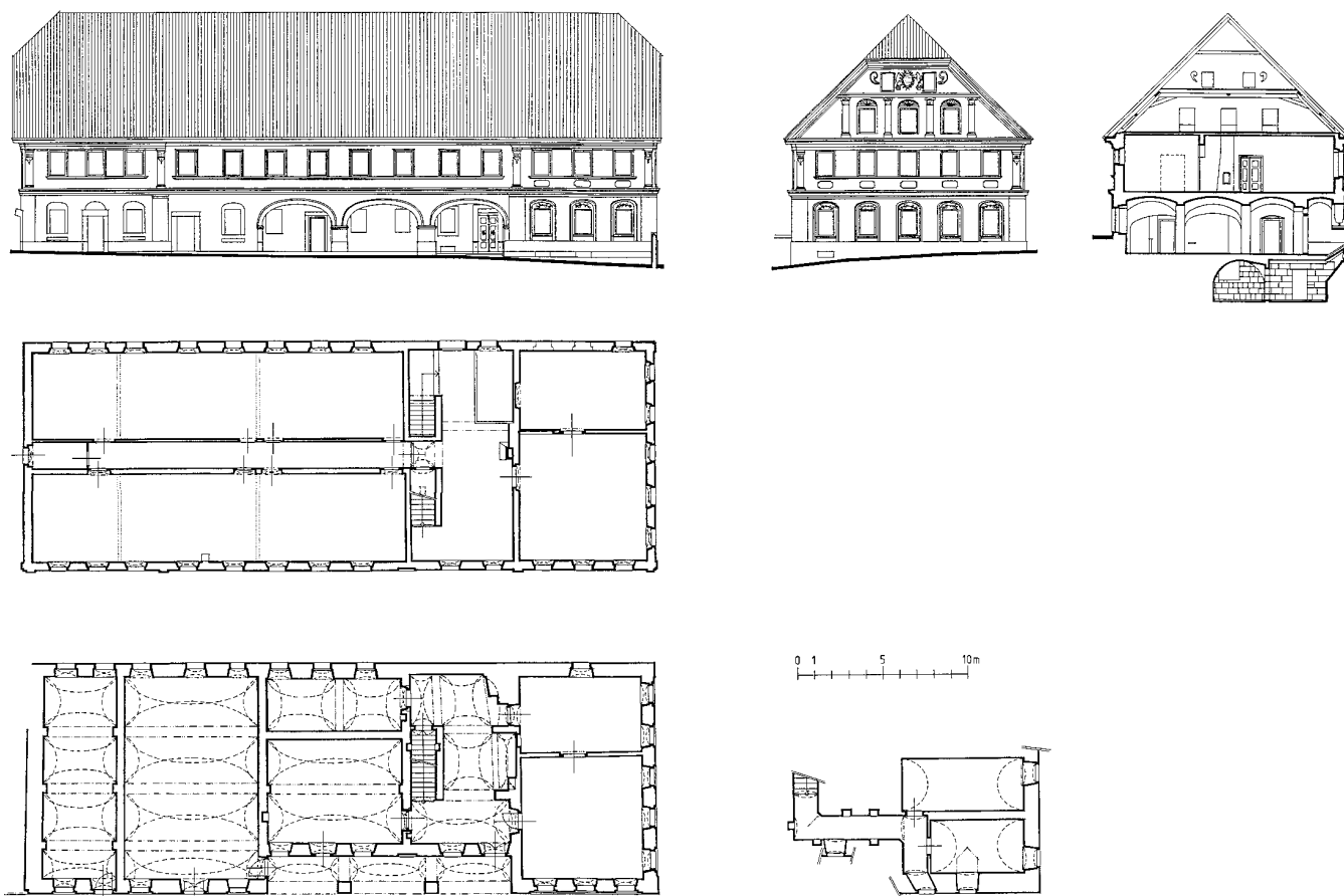
Obr. 6: Loubí, současná dokumentace domu usedlosti čp.1 s dobře patrnými diferencemi oproti navrženému stavu: levá arkáda ustoupila prodlouženému chlévu, trojdielné členění podélného průčelí bylo zvýrazněno řízalíťovým řešením a přidáním pilastrů. V zaměření jsou tečkovaně doplněny příčky mezi komorami v patře, odstraněné při adaptaci domu na drůbežárnu Státního statku Dubá (zaměření Š. Klobouková, J. Masák, J. Pešta, T. Russe a G. Steinová, 1995; kresba J. Pešta 1996).
