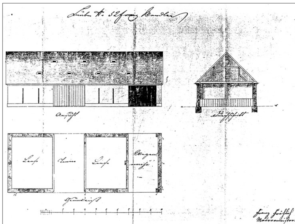
Obr. 33: Loubí, projekt stodoly pro čp. 52 (ve skutečnosti čp. 51): Lauben No 52 Franz Wendler, zednický mistr Franz Fröhlich, grafické měřítko (vídeňské sáhy), půdorys, pohled, řez (SOBa Děčín, Vs Česká Lípa, kt. 252, plán 1).
