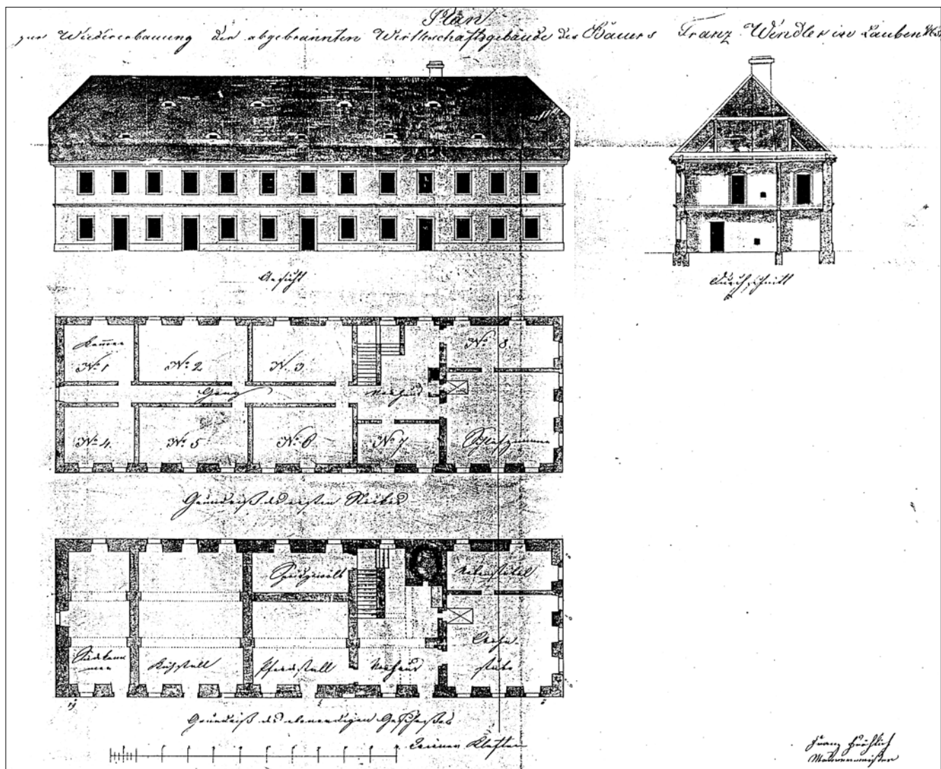
Obr. 28: Loubí, projekt novostavby domu usedlosti čp. 51: Plan zur Wiederaufbauung der abgebrannten Wirtschaftsgebäude des Bauers Franz Wendler in Lauben NC 51; s. d. (1843), Franz Fröhlich, grafické měřítko vídeňské sáhy, půdorysy přízemí a 1. patra, pohled (SOBA Děčín, Vs Česká Lípa, kt. 252, plán 10). Provedení plánu velkého domu je úsporné až schematické - podélné průčelí je nečleněné, štítové průčelí není zakresleno, plackové klenby v přízemí jsou jenom naznačeny situováním dělicích pasů.
