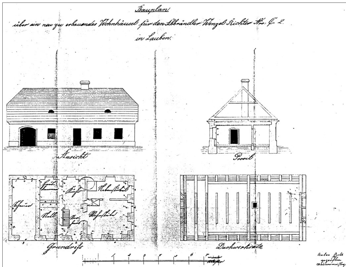
Obr. 9: Loubí, projekt na novou stavbu chalupy čp. 2: Bauplan über ein neu zu erbauendes Wohnhäusl für den Abbrändler Wenzel Richter Nro C 2 in Lauben, s. d. (1843), zednický mistr Anton Eisel, grafické měřítko vídeňské sáhy, půdorys, pohled, řez (SOBA Děčín, Vs Česká Lípa, kt. 252, plán 2). Pokud byl objekt (bohužel nedochovaný) postaven podle projektu a ve shodě s regulačním plánem z roku 1843, byla jeho čelní obytná strana směřována nevýhodně k severu a navíc do boční stěny domu sousední usedlosti čp. 3.
