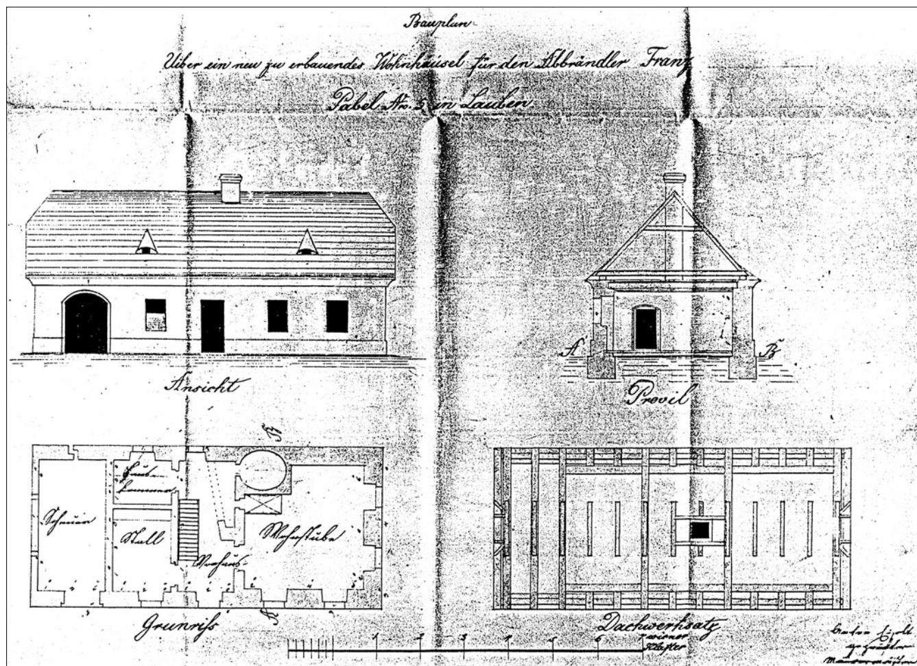
Obr. 11: Loubí, projekt na stavbu přemístěné chalupy čp. 5: Bauplan über ein neu zu erbauendes Wohnhäusel für den Abbrändler Franz Pabel Nro 5 in Lauben, s. d. (1843), zednický mistr Anton Eiselt, grafické měřítko vídeňské sáhy, půdorys přízemí, pohled, řez, vazba (SObA Děčín, Vs Česká Lípa, kt. 252, plán 8).
