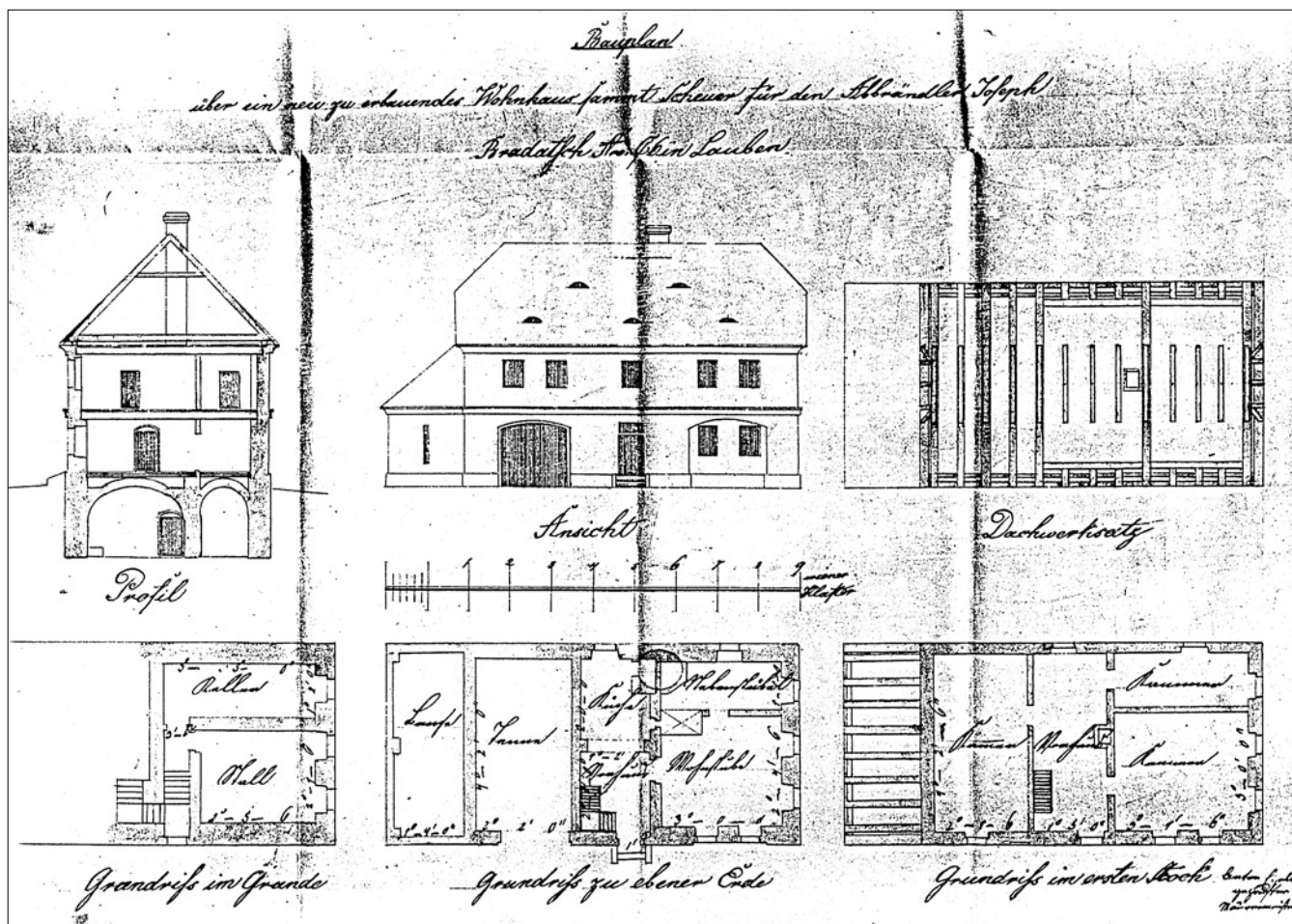
Obr. 12: Louboř, projekt na stavbu přemístěné chalupy čp. 6: Bauplan über ein neu zu erbauendes Wohnhaus sammt Scheuer für den Abbbrändler Joseph Bradatsch Nro C 6 in Lauben, s. d. (1843) zednický mistr Anton Eiselt, grafické měřítko vídeňské sáhy, půdorys sklepa, přízemí a prvního patra, pohled, řez, vazba (SOBa Děčín, Vs Česká Lípa, kt. 252, plán 9). Tento projekt (narozdíl od sousedního čp. 5) navrhoval patrové řešení objektu a reagoval na terénní situaci přemístěného staveniště situováním prostorných sklepů pod obytnou částí domu.
