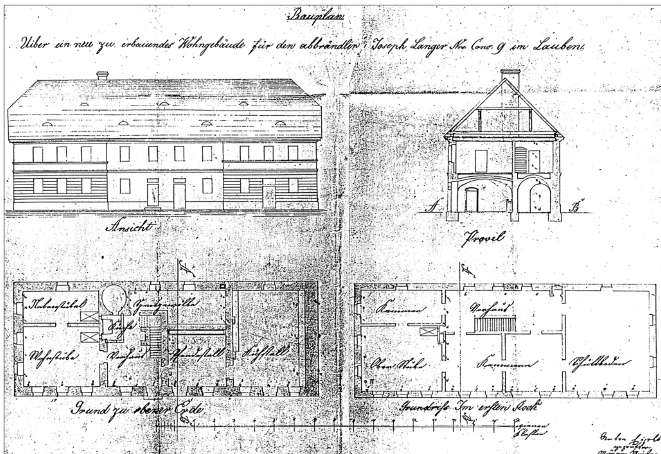
Obr. 18: Loubí, projekt nedochovaného domu usedlosti čp. 9: Bauplan über ein neu zu erbauendes Wohngebäude für den abbrändler Joseph Langer Nro Conv. 9 im Lauben, s. d. (1843), zednický mistr Anton Eisel, grafické měřítko vídeňské sáhy, půdorys přízemí a prvního patra, pohled, řez (SOBA Děčín, Vs Česká Lípa, kt. 252, plán 6). Kromě výrazného trojdílného řešení podélného průčelí je projekt zajímavý archaickým vynesením otevřeného dymníkového ústí komína nad topeništi v přízemí jenom úhlovou sestavou trámů a také umístění horní síně při zadní podélné stěně. Klenby nejsou v půdorysu vlastně vůbec vyznačeny - jejich samozřejmé užití je patrné jenom z řezu.
