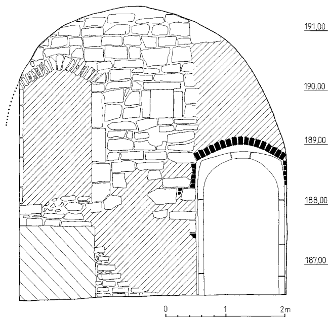
Obr. 2: Praha, Staré Město, dům čp. 456/I. Jižní, interiérový líc severní stěny nejstaršího objektu. Černě jsou vyznačeny cihly, šrafováním omítnuté partie, řidší šrafovou vystupující blok mladšího zdiva a tečkovaně předpokládaný průběh klenby za mladší přizdívkou. Silnější čarou zvýrazněn obrys odkládací niky (kresba M. Růžička a S. Matoušová, 1997).
