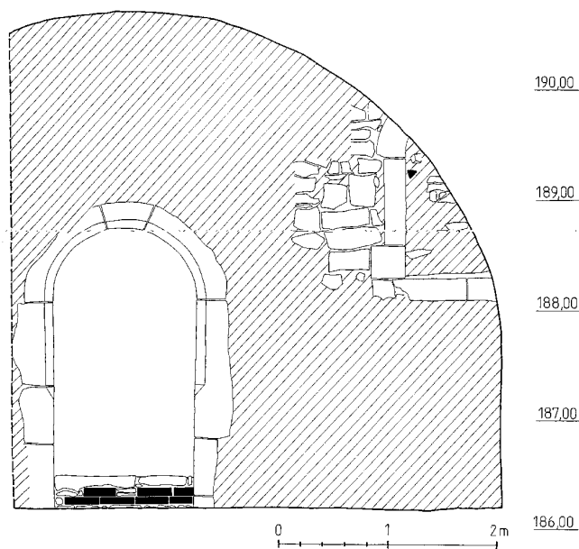
Obr. 3: Praha, Staré Město, dům čp. 456/I. Západní část severního, exteriérového líce severní stěny nejstaršího objektu. Černě značeny cihly, šrafovou omítané partie (kresba S. Matoušová, 1997).
