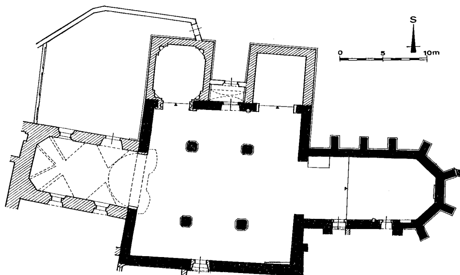
Obr. 5: Kadaň, půdorys přízemí klášterního kostela ve stavebně historické analýze, černě - zdivo gotické, šikmo šrafované - barokní (2 etapy), ostatní - mladší (kresba F. Kašička, 1997).
