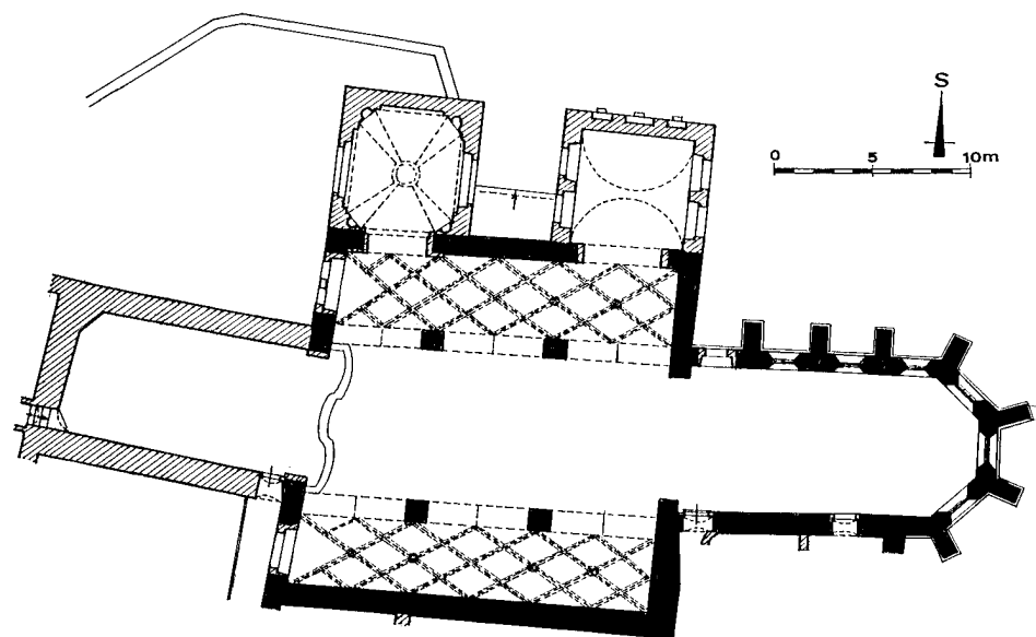
Obr. 6: Kadaň, půdorys 1. patra klášterního kostela ve stavebně historické analýze, značení zdiva viz přízemí (kresba F. Kašička, 1997).
