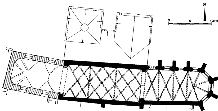
Obr. 7: Kadaň, půdorys v úrovni 2. patra klášterního kostela ve stavebně historické analýze, značení zdiva viz přízemí (kresba F. Kašička, 1997).
