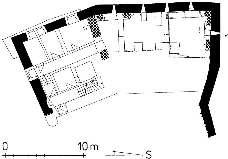
Obr. 6: Hrad Loket, tzv. Markrabský dům, půdorys suterénu. Černě zdivo pozdně románské, křížem šrafováno pozdně gotické.
