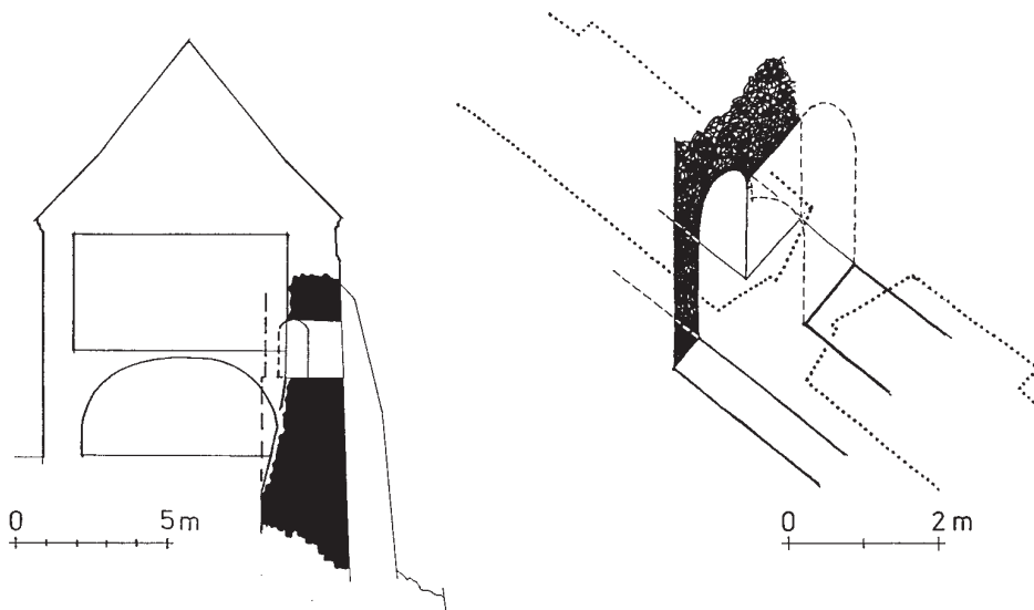
Obr. 14: Hrad Loket, východní křídlo. Vlevo schematický řez objektem - černě označeny pozdně románské konstrukce obsahující v patře chodbičku v síle zdiva, čárkováně předpokládaný původní stav. Vpravo chodbička s odbočkou v síle pozdně románské zdi, částečná rekonstrukce nalezeného stavu, tečkovaně dnešní půdorys zdi zeslabené z vnitřku a překryté přízdívkou z vnějšku (všechny kresby a fotografie autor, 1998).
