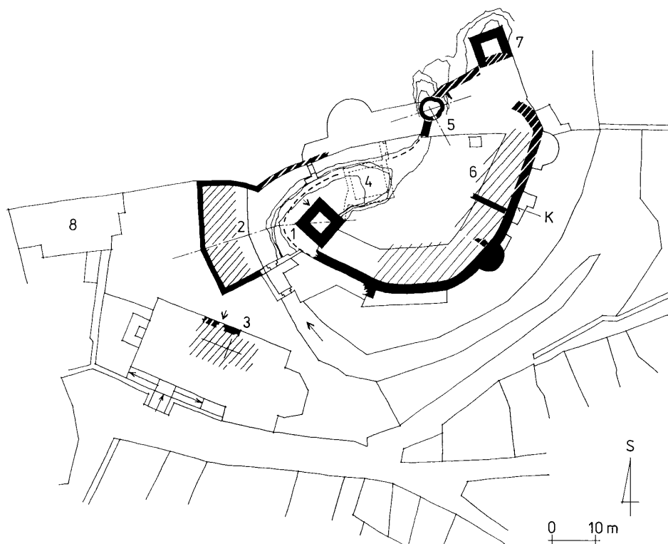
Obr. 4: Půdorysné schéma hradu Loket s vyznačením pozdně románských objektů podle stavu průzkumu k r. 1997. Zvýrazněna je předpokládaná kompoziční osa svazující starší jádro hradu - bergfrit a tzv. Markrabský dům; dále vyznačena podélná osa rotundy a osa jejího vstupu natočená k východu. Natočení osy vstupu vypovídá o koexistenci rotundy a hradby, která k ní přiléhá. 1 - bergfrit, 2 - tzv. Markrabský dům, 3 - románský kostel na místě děkanského chrámu sv. Václava, 4 - tzv. Skalní světnice (románský původ není doložen!), 5 - rotunda, 6 - přemyslovský palác s chodbičkou v síle zdiva - K, 7 - stavení na severní výšce, snad věž, 8 - děkanství. Černé zdivo pozdně románské, přerušované zdivo pravděpodobně pozdně románské nebo půdorysná stopa pozdně románského zdiva. Šrafované je znázorněn hypotetický rozsah objektů.
