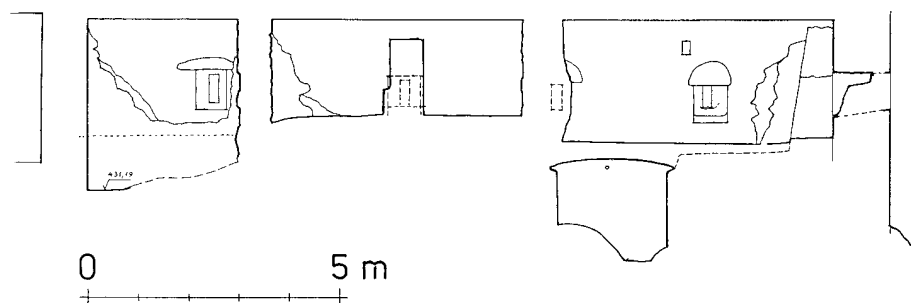
Obr. 7: Hrad Loket, tzv. Markrabský dům, podélný řez nově zpřístupněnou částí suterénu s pohledem na západní stěnu s okny.
