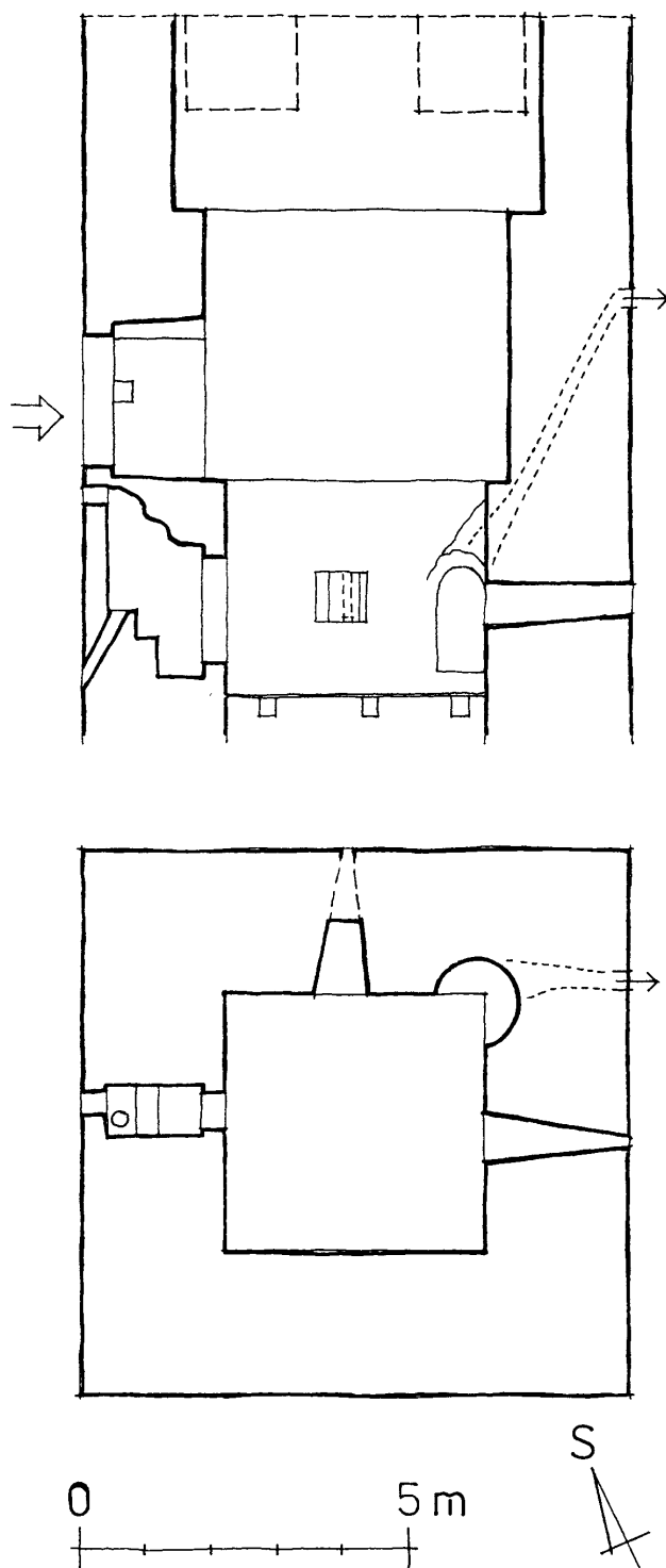
Obr. 11: Hrad Loket, horní část pozdně románského bergfritu - řez a půdorys refugia se záchodem a krbem s vyznačením dochovaného vyústění dymníku krbu do vnějšího lince věže románského vstupu do věže (velká šipka) a dochovaného románského cimbuří (čárkovaně).
