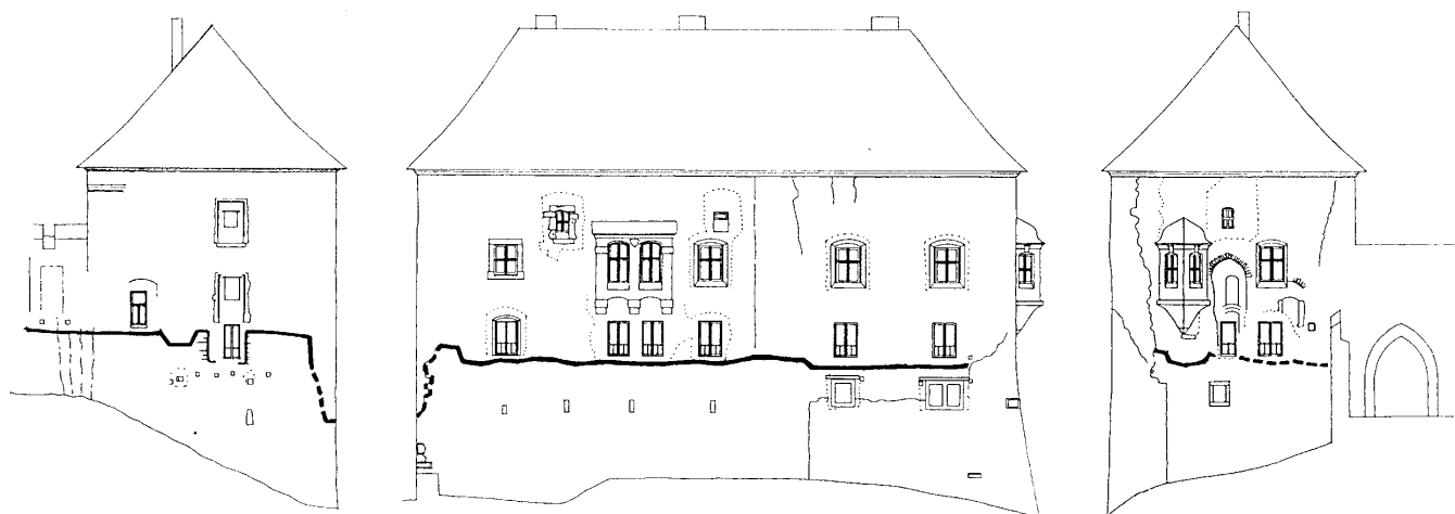
Obr. 8: Hrad Loket, tzv. Markrabský dům; zleva: severní, západní a jižní průčelí. Pod silnou linií se nalézají pozdně románské konstrukce (s mladšími velkými okny a přízdívkami opěráku při jihozápadním nároží).
