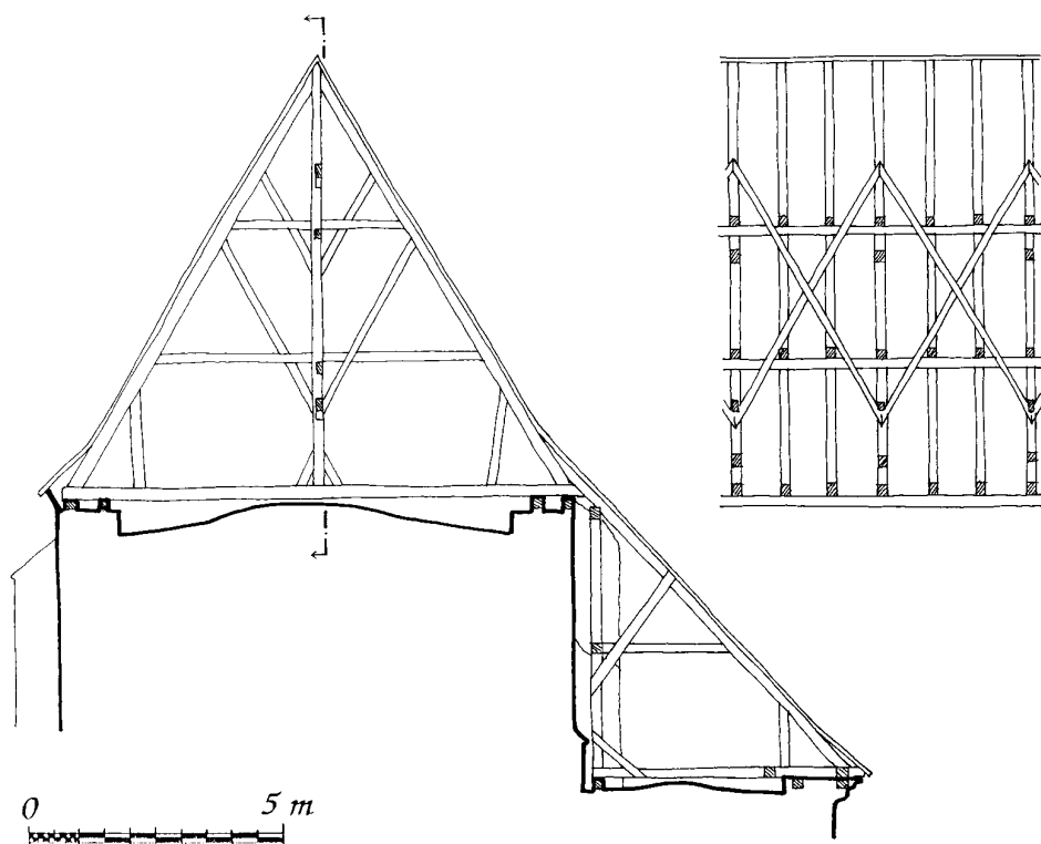
Obr. 10: Pohled, schéma příčného řezu krovem kostela sv. Ondřeje a přilehlé chodby a podélného řezu krovem kostela (zpracoval L. Svoboda).
