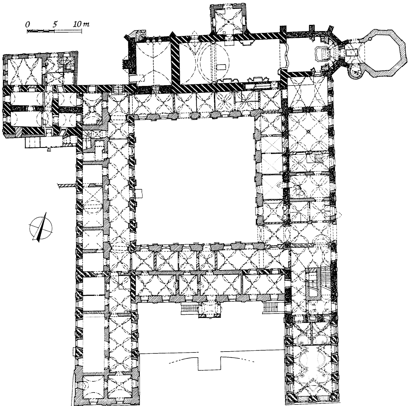
Obr. 4: Pohled, půdorys přízemí bývalého kláštera a kostela sv. Ondřeje se stavebně historickou analýzou. Černě položené zdivo z doby před rokem 1265, zrněné zdivo gotické, křížkované renesanční, šrafované barokní, dvojité šrafované klasicistní a tečkované novodobé. Prerušované značeno zdivo hypoteticky zařazené (plánový podklad zpracovala J. Svobodová, odbornou náplň L. Svoboda).
