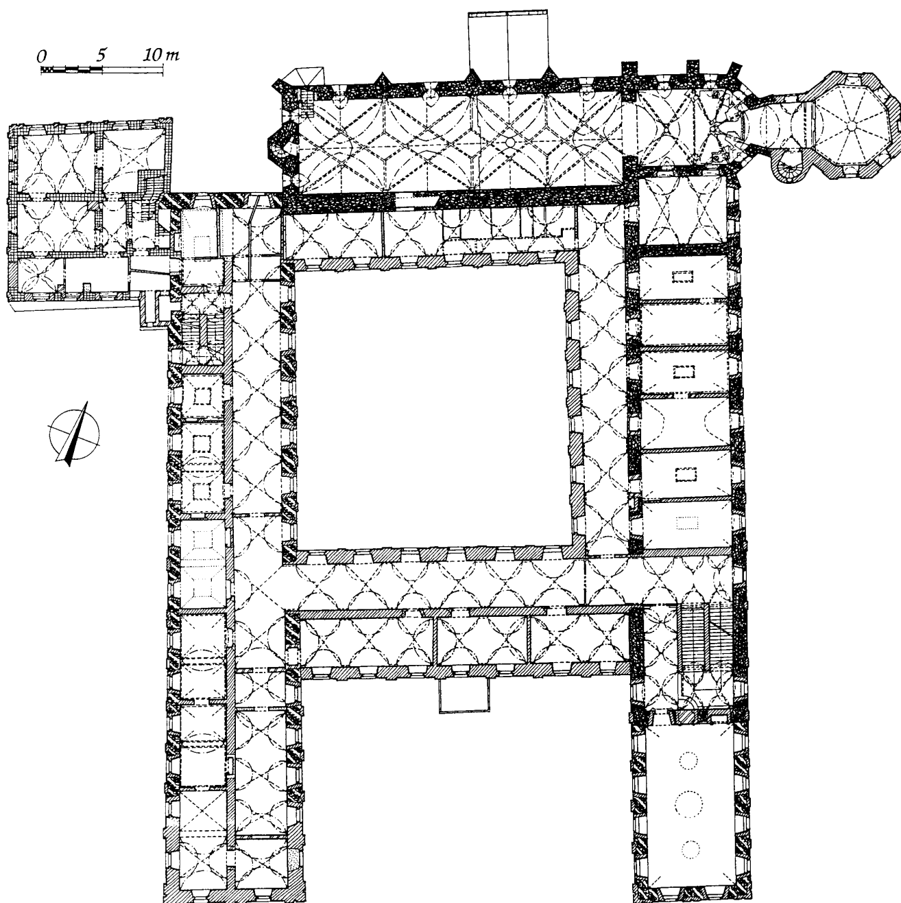
Obr. 5: Pohled, půdorys 1. patra bývalého kláštera a kostela sv. Ondřeje se stavebně historickou analýzou. Zrněné zdivo gotické, křížkované renesanční, šrafované barokní, dvojité šrafované klasicistní a tečkované novodobé. Přerušované značeno zdivo hypoteticky zařazené (plánový podklad zpracovala J. Svobodová, odbornou náplň L. Svoboda).
