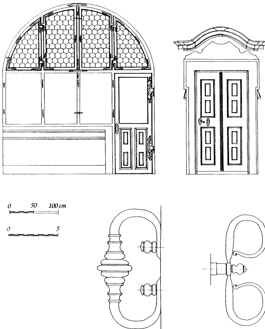
Obr. 17: Pohled, nárys přičky mezi hlavním schodištěm a chodbou v 1. patře klášterního konventu, portál letního refektáře (nahore) a detaily kování přičky (dole; zpracovala J. Svobodová).
