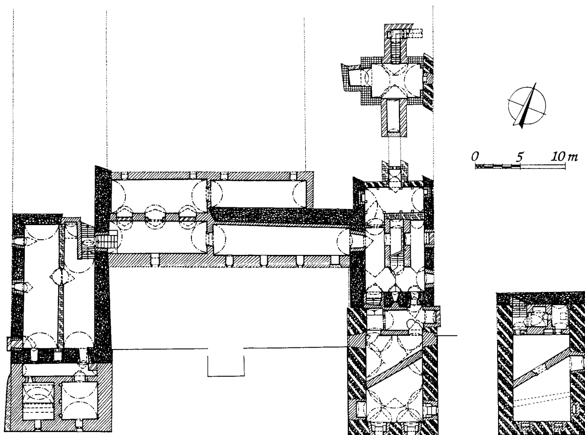
Obr. 3: Pohled, bývalý klášter. Půdorys sklepů bývalého kláštera (vpravo dole spodní úroveň jižního konce východního křídla) se stavebně historickou analýzou. Zrněné zdivo gotické, křížkované renesanční, šrafované barokní, dvojité šrafované klasicistní a tečkované novodobé. Prerušované značeno zdivo hypoteticky zařazené (plánový podklad zpracovala J. Svobodová, odbornou náplň L. Svoboda).
