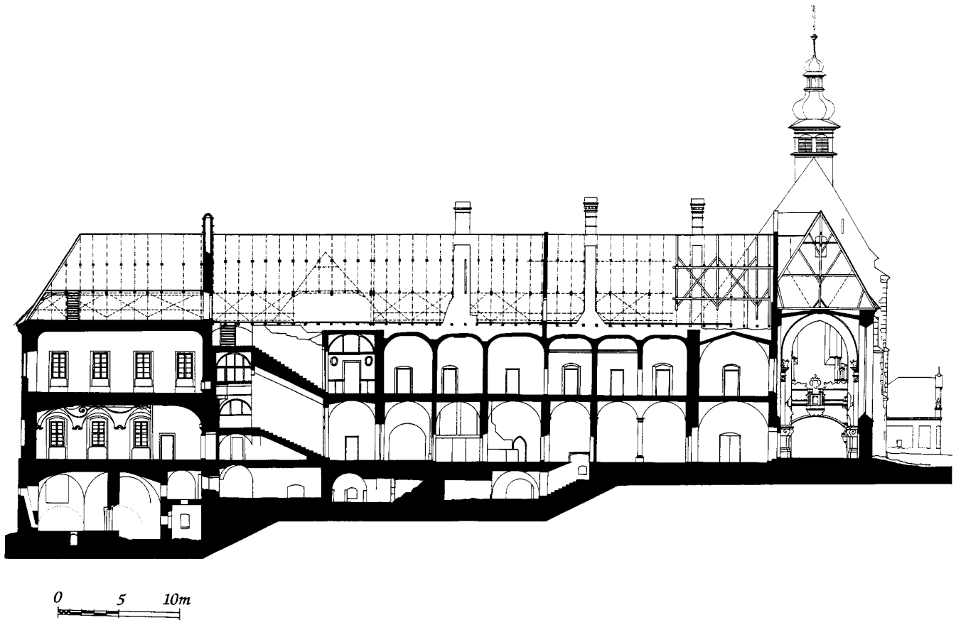
Obr. 11: Pohled, podélný řez hlavním traktem východního křídla klášterního konventu s navazujícím příčným řezem presbytářem kostela sv. Ondřeje (zpracovala J. Svobodová).
