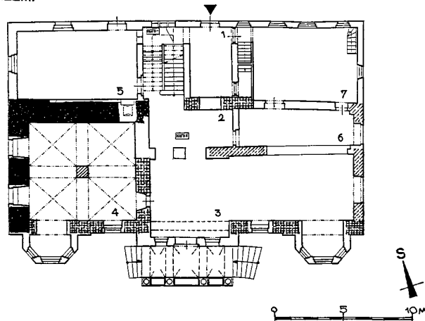
Obr. 4: Michalovice (okr. Mladá Boleslav), novorenesanční vila. Půdorys přízemí a 1. patra ve stavebně historické analýze; černá - předpokládané konstrukce středověké, mřížky - renesanční, šikmá šrafování - barokní, ostatní - novodobé, přerušovaná šrafování - zařazení hypotetické.
