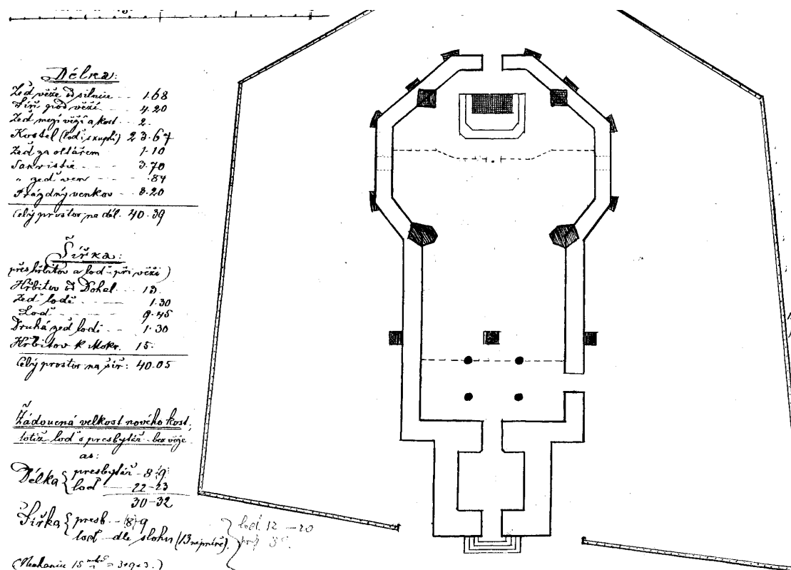
Obr. 18: Dohaličky (okr. Hradec Králové), kostel sv. Jana Křtitele, půdorys z roku 1888 od P. Jana Macháčka (SOBA Zámorsk, Vs Sadová, kart. 392).
