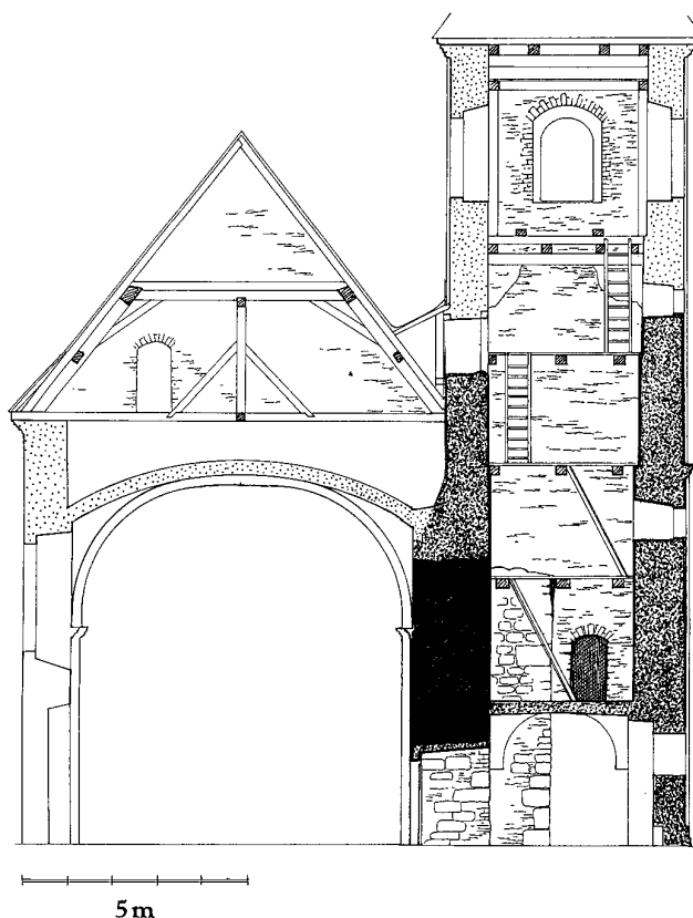
Obr. 3: Kostel sv. Prokopa v Lestkově. Rez a - b černě označeno předpokládané románské zdivo, hustě tečkována starší barokní fáze, řídce tečkována mladší barokní fáze.
