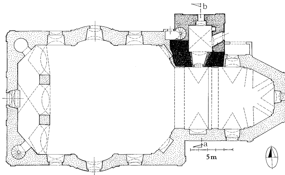
Obr. 4: Kostel sv. Prokopa v Lestkově. Černě označeno předpokládané románské zdivo, hustě tečkována starší barokní fáze, řídce tečkována mladší barokní fáze (zaměření autor, 1998)
