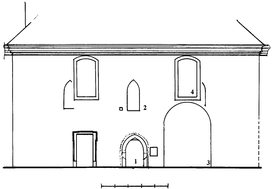
Obr. 3: Všeradice, kostel sv. Bartoloměje, pohled na jižní průčelí lodi se zákresem odkrytých otvorů. 1 - gotický portál, 2 - gotická okna, 3 - oblouk, původně otevřený do přistavěné kaple, 4 - barokní okna z roku 1765 (zaměření a kresba autor).
