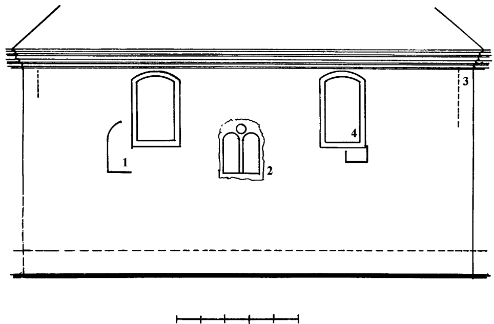
Obr. 4: Všeradice, kostel sv. Bartoloměje, pohled na severní průčelí lodi se zákresem odkrytých otvorů. 1 - zbytky gotických oken, 2 - renesanční okno, 3 - zbytky malovaných lesen, 4 - barokní okna (zaměření a kresba autor).
