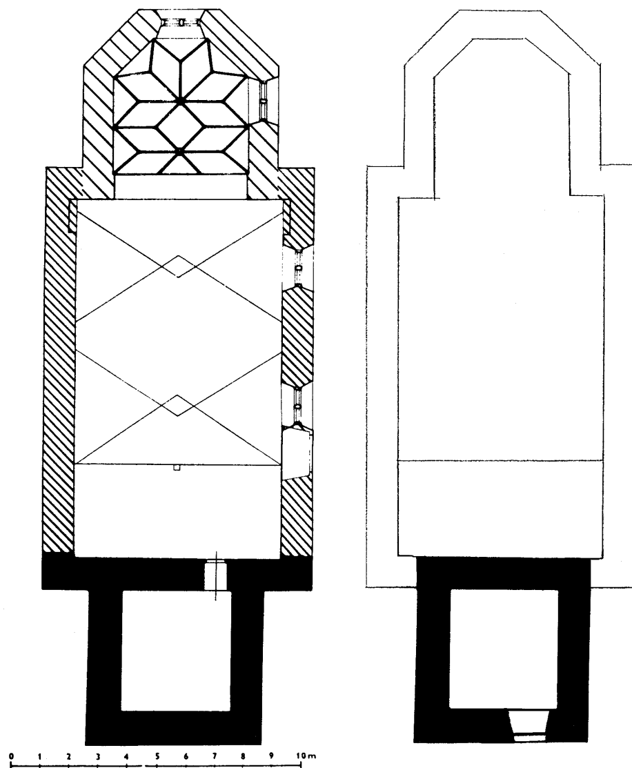
Obr. 2: Půdorys kostela sv. Ducha v Telči s věží, zkoumaná část černě (přízemí, 1. patro).
