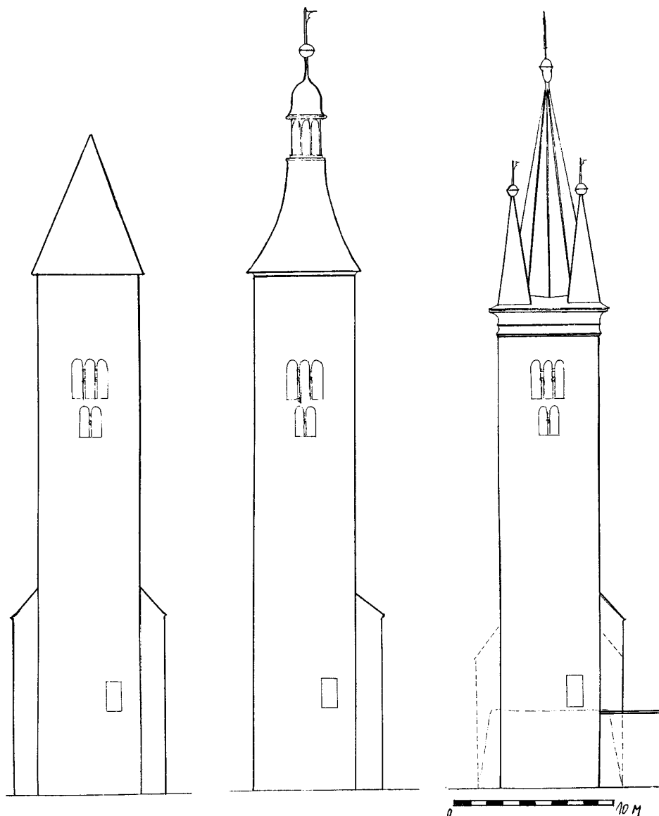
Obr. 7: Telč, kostel sv. Ducha, rekonstrukce vývojových etap věže: vlevo pokus o rekonstrukci románské podoby z konce 13. století, uprostřed stav začátku 18. století s barokní helmicí, vpravo stav současný s tvarem střechy z poloviny 19. století, čárkovaná poloha odstraněného vysokého soklu.
