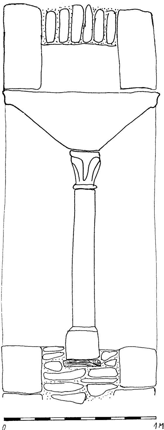
Obr. 5: Telč, kostel sv. Ducha, řez podvojným oknem: patka sloupku spočívá na dřevěné desce v litém zdivu, v nadpraží z obou čel kamenné prvky, uprostřed opět lité zdivo s nosným obloukem skládaným z lomových prvků.
