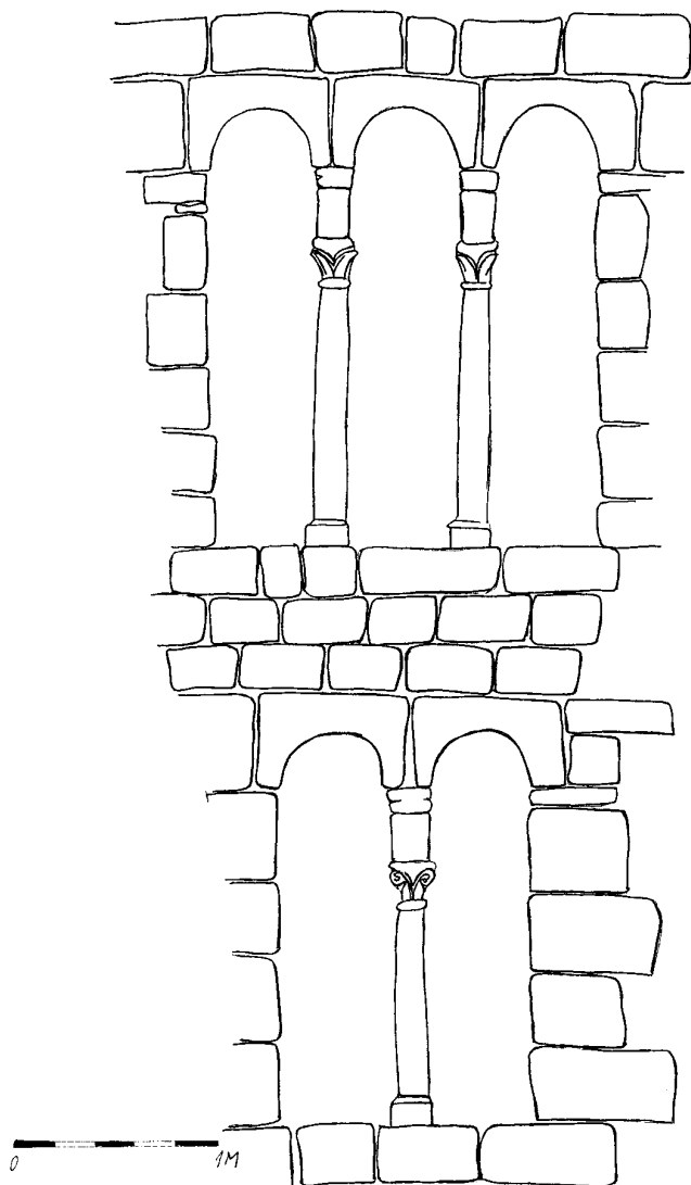
Obr. 4: Telč, kostel sv. Ducha, zaměření polohy podvojného a potrojného okna v západní stěně.
