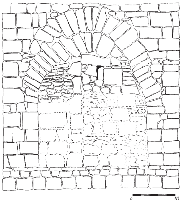
Obr. 3: Telč, kostel sv. Ducha, zaměření patra věže - zdivo východní stěny věže s emporou (dvojitý oblouk postupně zazdívaný, uprostřed ponechaný větrací otvor).
