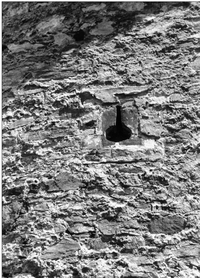
Obr. 13: Český Krumlov. Novoměstská nárožní bašta, čp. 28. Detail klíčové střílny se zbytky omítkové pasparty v 1. patře (foto autor, 1998).
