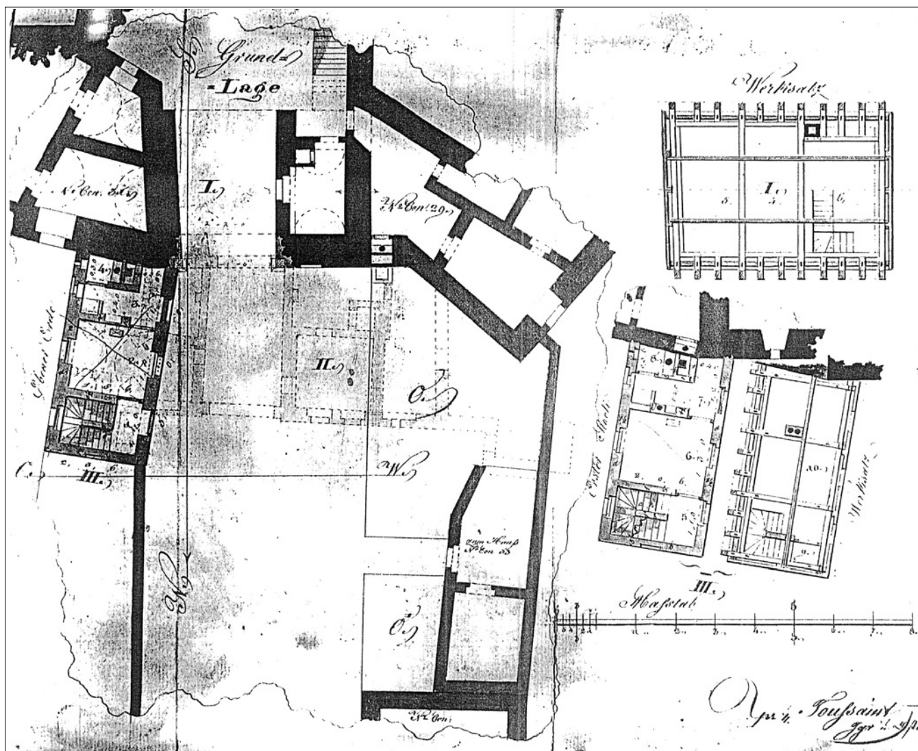
Obr. 30: Český Krumlov. Vnější Latránská brána, zaměření z roku 1841 (OkA Č. Krumlov). Před přízemím brány (vlevo) naznačen půdorys renesančního předbraní. V dolní části je zřejmý způsob návaznosti zdi koridoru směrem k Budějovické bráně.
