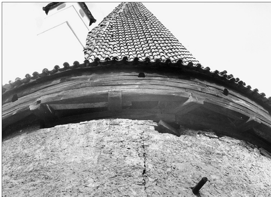
Obr. 17: Český Krumlov. Novoměstská nárožní bašta, čp. 28. Detail konstrukce roubeného podstrešního patra se střílnami a podsebitím. Místo předělu mezi původním a dodatečným zdivem bašty (foto autor, 1998).
