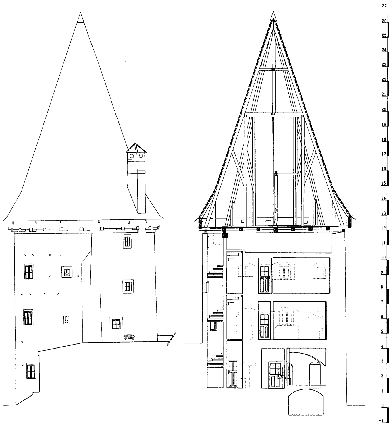
Obr. 19: Český Krumlov. Novoměstská nárožní bašta, čp. 28. Vlevo pohled od západu, upravo svislý řez v pohledu od jihu. 1 - půdorys v úrovni sklepa, 2 - půdorys přízemí, 3 - půdorys 1. patra, 4 - půdorys 2. patra, 5 - půdorys v úrovni horního polopatra, 6 - půdorys v úrovni roubeného patra. Gotické zdi-vo vyznačeno šrafovou pouze v přízemí, z důvodu přehlednosti a nejasných přechodů na pozdější stavební fáze (zaměření Martin Černý a kol., XII/1996).
