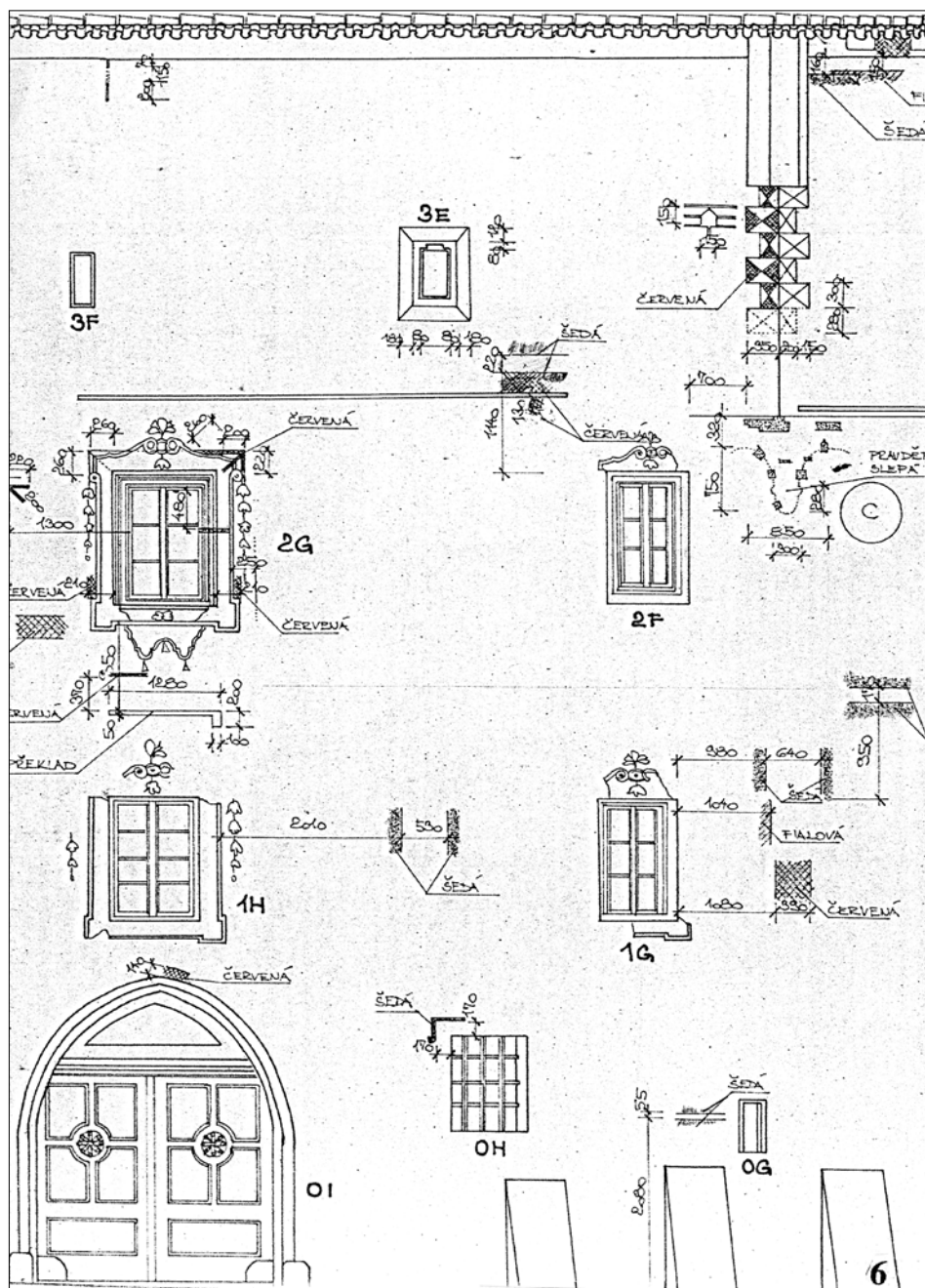
Obr. 1: Český Krumlov, dům čp. 32, výsek severního průčelí (měřická dokumentace SÚRPMO z roku 1967, zakreslení nálezu Arnošt Janke, 1997).
