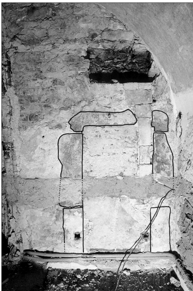
Obr. 8: Praha 1 - Staré Město, Staroměstské náměstí čp. 549/I. Zazděný pravoúhlý portál v interiéru gotické stavby uprostřed parcely. Pohled od severu (foto P. Cajthaml).
