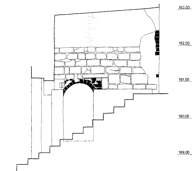
Obr. 3: Praha 1 - Staré Město, Staroměstské náměstí čp. 549/I. Východní bok románské vstupní šije. Černě značený cihly, šrafované část zazdívký románské odkládací niky, porušené mladším vstupním otvorem. Tečkovaná spára v bednění románské valené klenby (kresba M. Semerád, J. Špaček a S. Matoušová).
