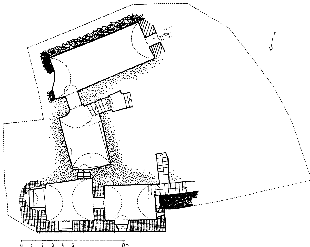
Obr. 3: Skalná (okr. Cheb), půdorys suterénu hradu Vildštejna, černě vyznačeno románské zdivo nejstarší fáze, křížkovane nejmladší fáze, tečkovaně přitěsaná skála. Upravené zaměření z r. 1967, ulož. v projektovém archivu PŮ v Plzni (kresba T. Karel).
