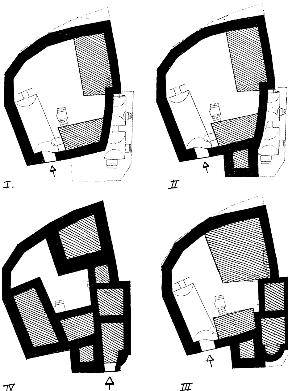
Obr. 6: Skalná (okr. Cheb), hrad Vildštejn, schéma vývoje hradní dispozice, I - nejstarší fáze kol. r. 1200, II - druhá fáze kol. r. 1230, III - třetí navazující fáze, IV - goticko renesanční fáze (kresba T. Karel).
