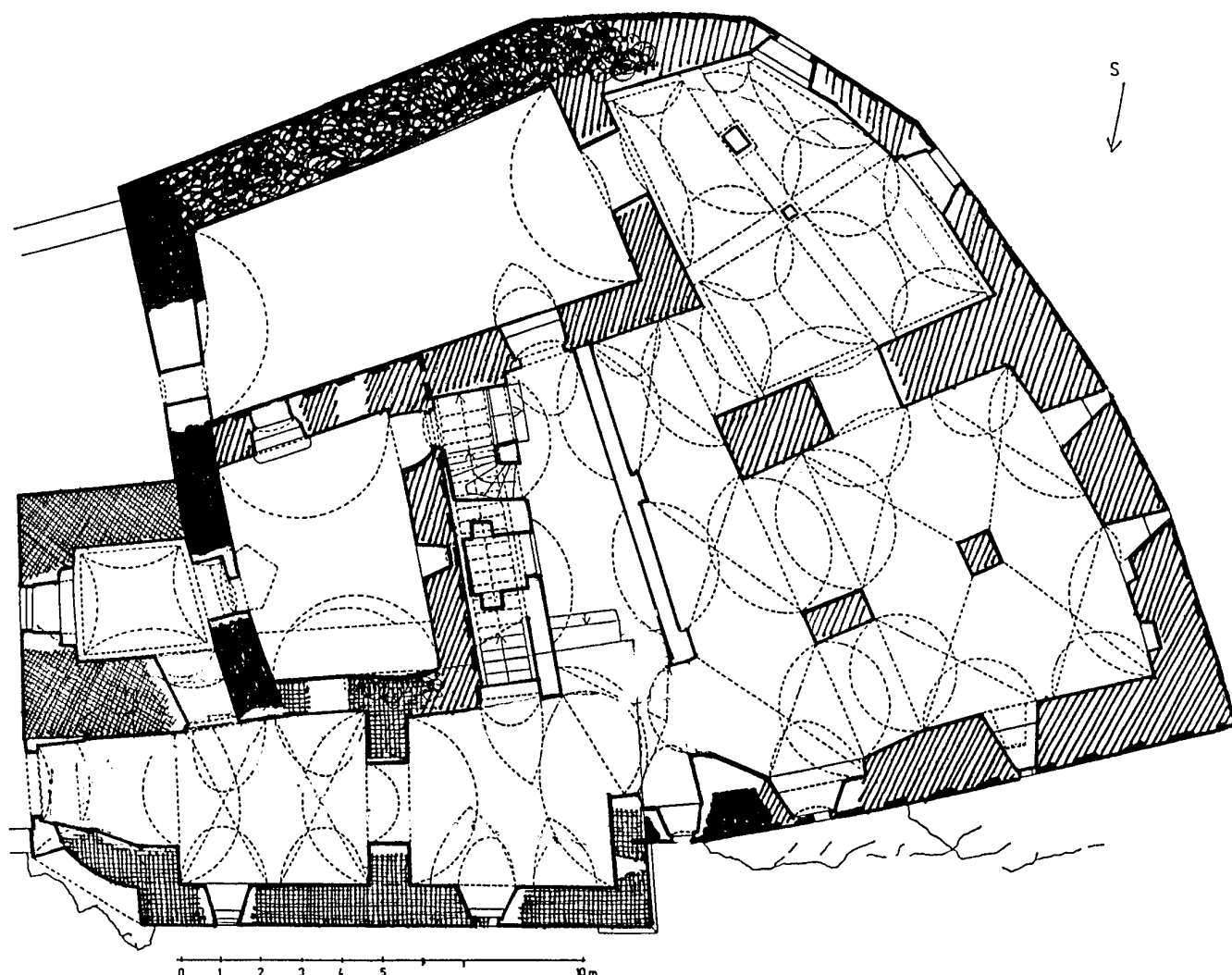
Obr. 4: Skalná (okr. Cheb), hrad Vildštejn, půdorys přizemí, černě vyznačeno románské zdivo nejstarší fáze, přerušovanou čarou naznačen předpokládaný rozsah obvodu, křížkovane šikmo střední fáze, křížkovane kolmo nejmladší románská fáze, šikmo pozdně gotické zdivo. Upravené zaměření z r. 1967, uložen v projektovém archivu PÚ v Plzni (kresba T. Karel).
