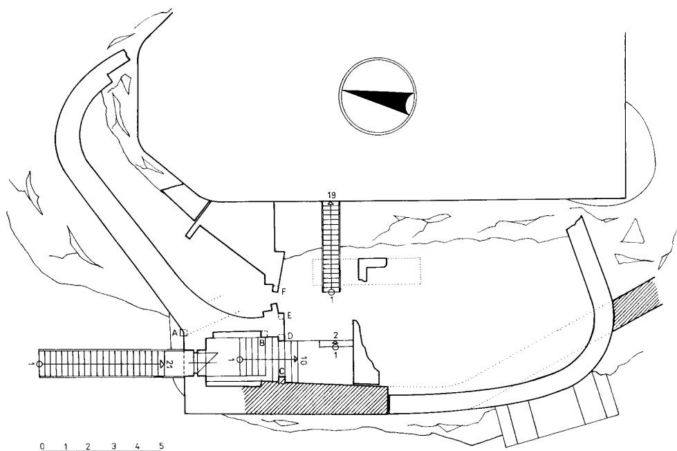
Obr. 7: Hrad Vlčejn (okr. Plzeň - jih). Situace vstupu do příhrádku a paláce, A - pískovcový blok patrně in situ, B až F - druhotně osazené pískovcové prvky, tečkovaně - průběh zdiva na Heberově plánu (zaměření M. Novobilský, P. Rožmberský, H. Slavíková, kresba M. Novobilský, 1999).
