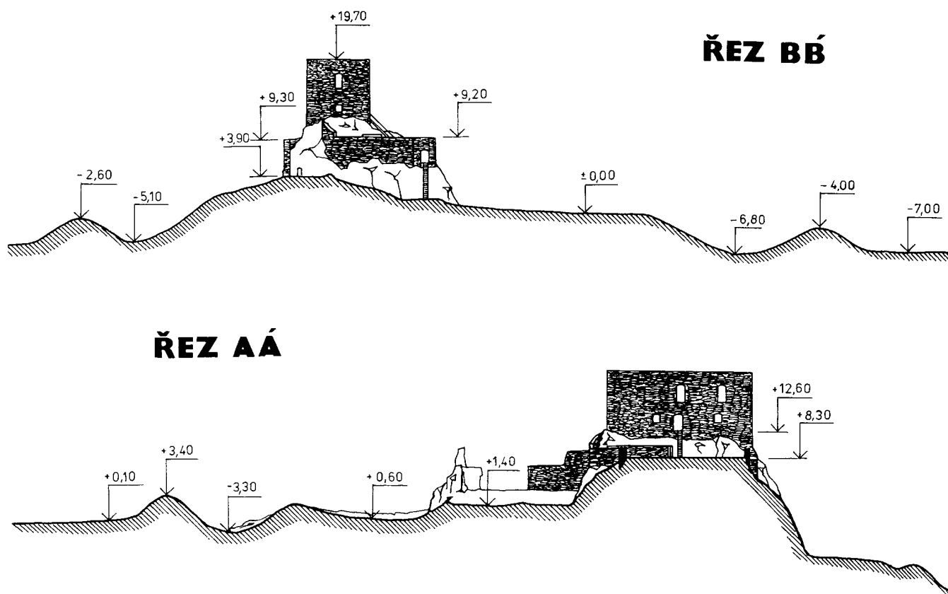
Obr. 4: Hrad Vlčtejn (okr. Plzeň - jih). Pohledové řezy terénem (podle zaměření P. Nožičky kreslil M. Novobilský, 2000).
