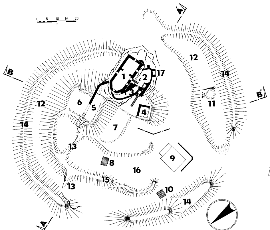
Obr. 3: Hrad Vlčtejn (okr. Plzeň - jih). Podrobná situace hradu. 1 - palác, 2 - dvorek příhrádky, 3 - úzká část příhrádky, 4 - Hejtmánkem objevený „strážní domek“, 5 - velký objekt na předhradí, pozdější sýpka, 6 - širší parkán, 7 - místo upravené na přírodní divadlo, 8 - bývalé WC, 9 - parket, 10 - bývalé obědovnění, 11 - jáma považovaná za studnu, 12 - vnější příkop, 13 - skalnatá hrázka v příkopu, 14 - vnější val, 15 - vnitřní val, 16 - vnitřní příkop, 17 - branka (podle zaměření P. Nožičky kreslil M. Novobilský, 2000).
