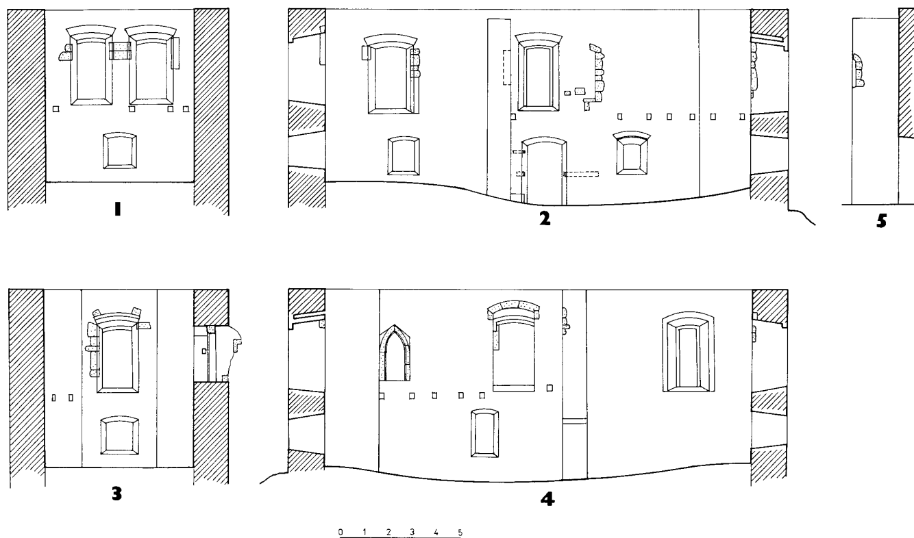
Obr. 6: Hrad Vlčejn (okr. Plzeň - jih). Pohledy do interiéru paláce. Lokalizace pohledů viz obr. č. 5. (kresba M. Novobilský, 2000).
