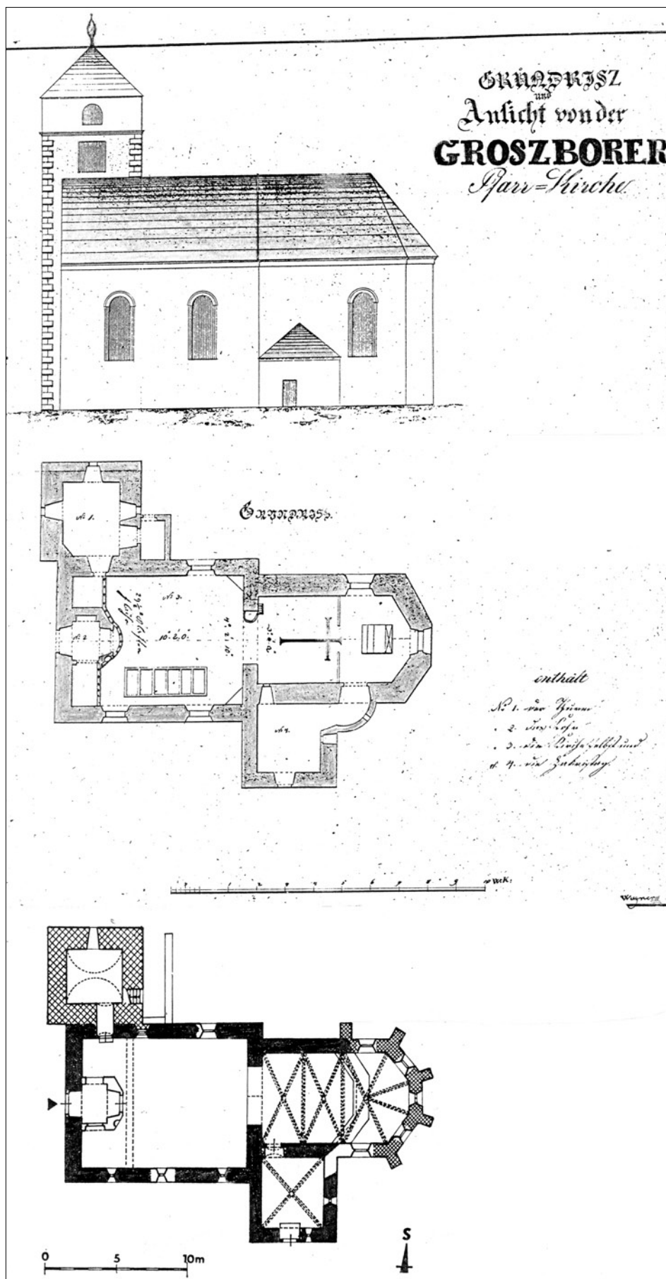
Obr. 9: Kostel sv. Jana Křtitele ve Velkém Boru v roce 1798, dole půdorys kostela dle F. Kašičky a B. Nechvátala (Velký Bor; půdorys farního kostela ve stavebně historické analýze, hustota šrafování označuje 3 základní etapy středověké výstavby památky).
