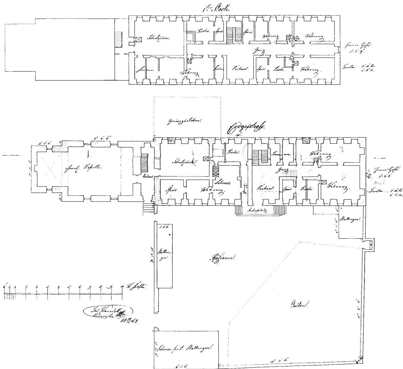
Obr. 11: Plán školy ve Velkém Boru, zpracovaný baumistrem Josefem Vaněčkem 20. 12. 1854.
