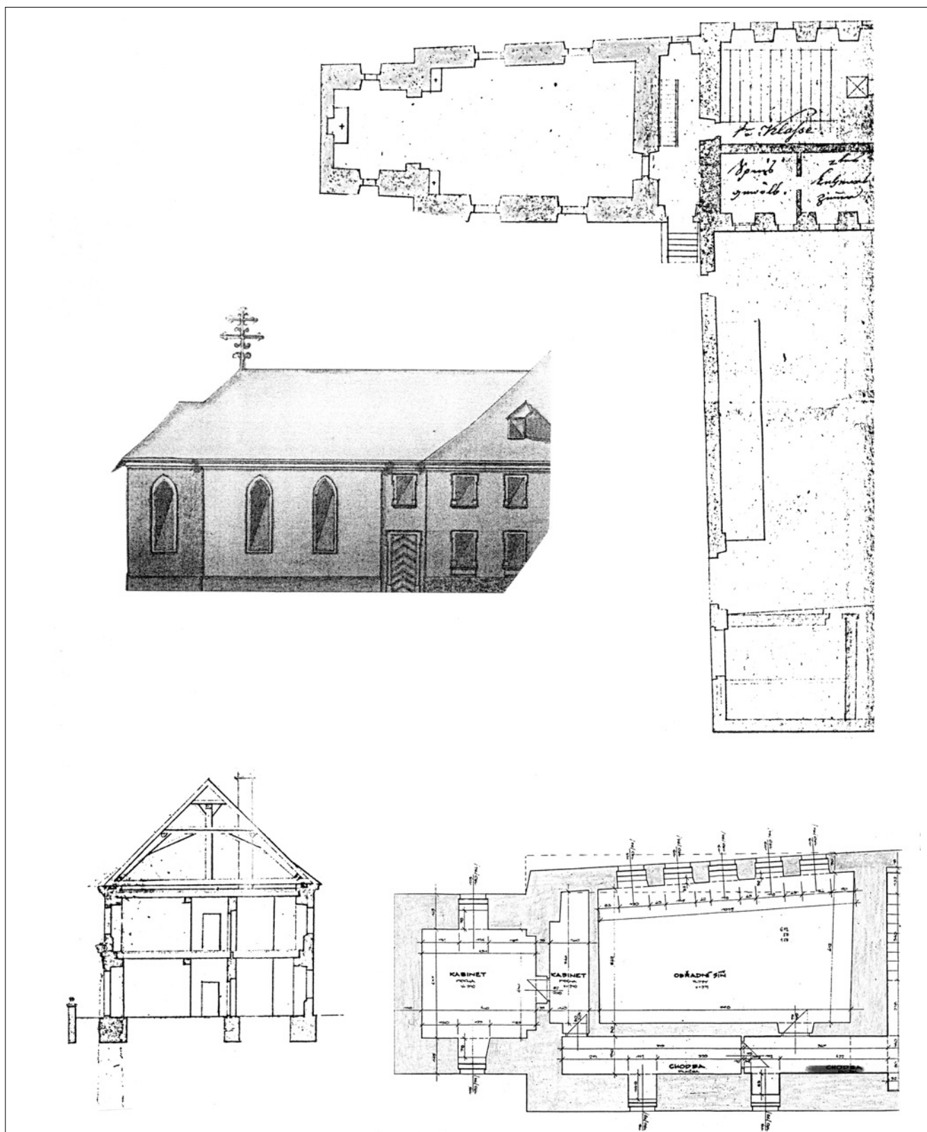
Obr. 10: Kaple sv. Buriana ve Velkém Boru. V horní části půdorys a boční pohled kaple sv. Buriana, dole příčný řez špitálu z r. 1770 a půdorys bívalé kaple, nyní bytu, černě - zdivo renesanční, bíle - novodobé (stav roku 2000).
