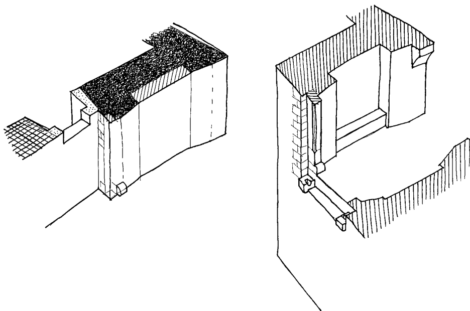
Obr. 3: Svinná (okr. Rokycany), detailní řezy nejstarší částí východní stěny s vyznačením stáří konstrukcí a ideální rekonstrukcí gotického stavu brány.
