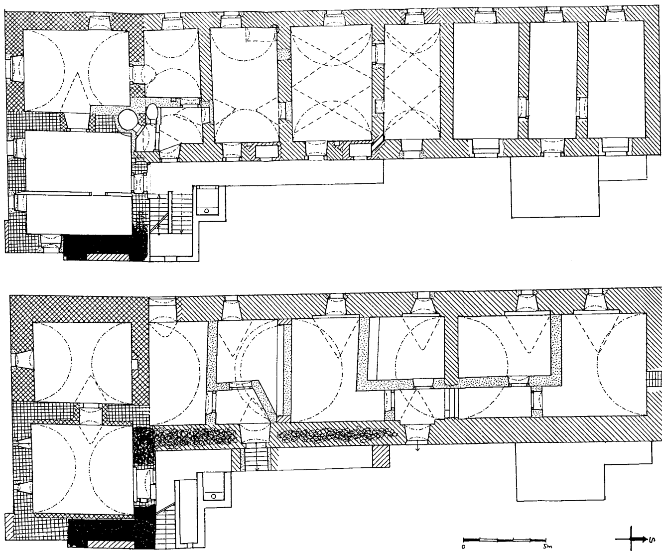
Obr. 2: Svinná (okr. Rokycany), půdorys prvního podlaží - polosuterénu a druhého podlaží s vyznačením stáří konstrukcí. Černě nejstarší gotické zdivo brány a obvodové hradby, křížkovane kolmo zdivo pozdně gotické přístavby, křížkovane šikmo zdivo goticko renesanční přístavby, šikmo zdivo renesanční, šikmo zleva doprava barokní dozdívky, tečkované empírové úpravy, bez označení zdivo mladší.
