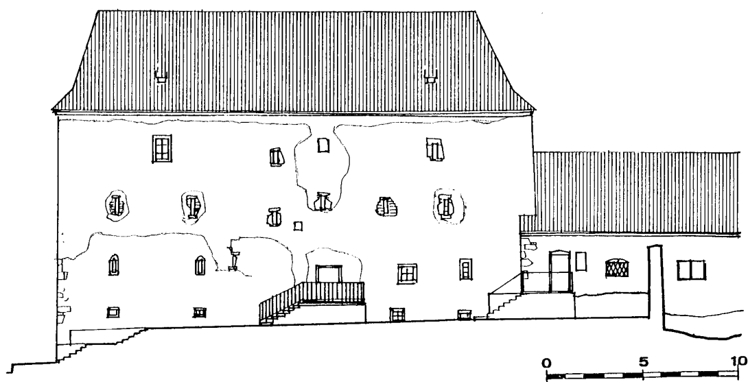
Obr. 9: Volyně, nárys severního průčelí budovy tvrze se schematickým označením hranic odlišné materiálové skladby.
