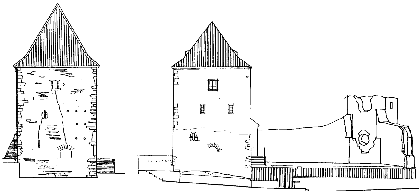
Obr. 8: Volyně, nárys východního průčelí tvrze podle zaměření z roku 1908 (?) a dnešního stavu.
