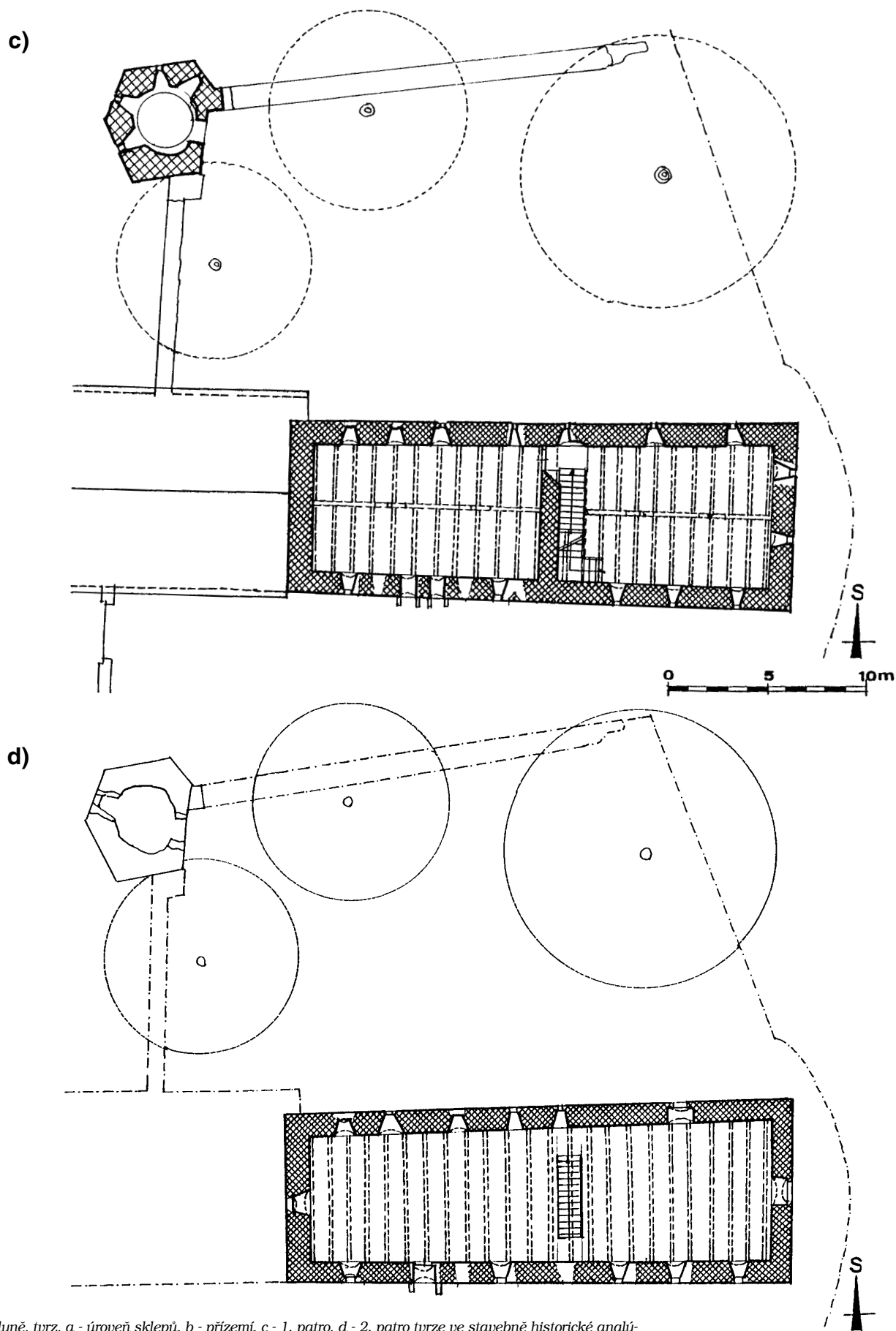
Obr. 7: Volyně, tvrz, a - úroveň sklepů, b - přízemí, c - 1. patro, d - 2. patro tvrze ve stavebně historické analýze. Společná legenda k analytickým plánům: Černě je označeno zdivo hypoteticky zařazené do 13. století, hustě mřížkované - do 14. století, řídko mřížkované - na šedém podkladě - 1. fáze pozdně gotické hradby, bez podkladu - 2. fáze gotické hradby, mřížky kolmé ke konstrukci značí zdivo renesanční a šikmé dvojčáry - klasicistní. Ostatní zásahy byly ponechány bílé.
