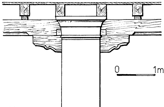
Obr. 13: Plešnice (okr. Plzeň - sever). Detail pilíře a konzol v přízemí sýpky (kresba M. Novobilský, 1999).
