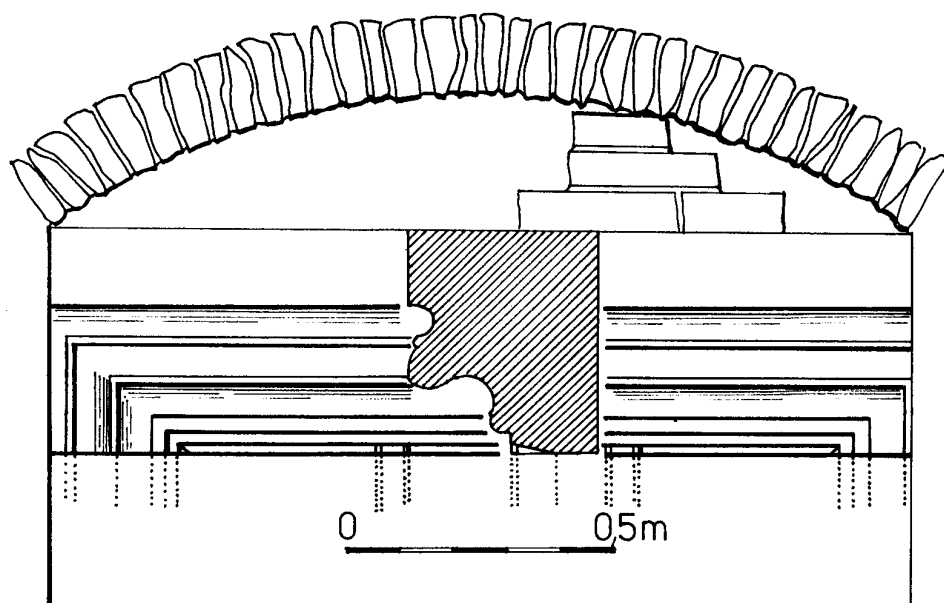
Obr. 11: Plešnice (okr. Plzeň - sever). Nadpraží vstupního portálu do sklepa (zaměření a kresba M. Novobilský, 2000).
