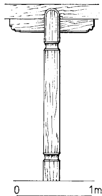
Obr. 12: Plešnice (okr. Plzeň - sever). Detail sloupku a konzol průvlaku v 1. patře sýpky (kresba M. Novobilský, 1999).
