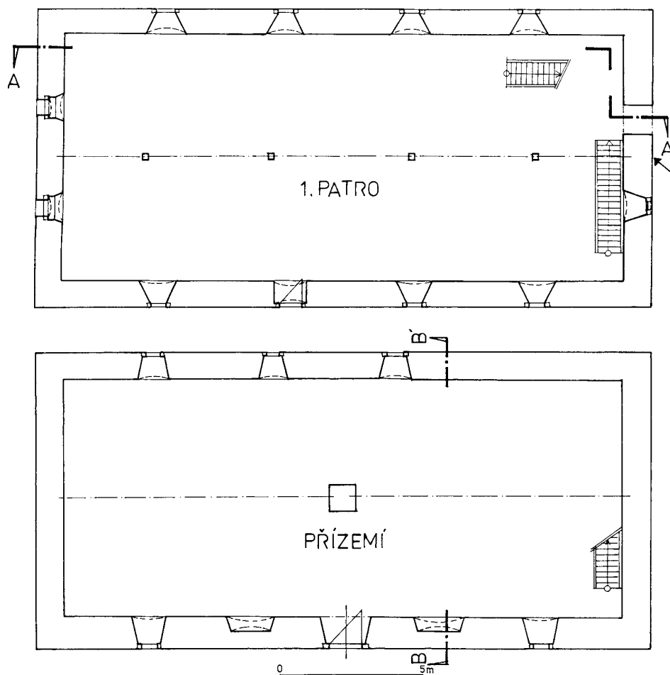
Obr. 8: Plešnice (okr. Plzeň - sever). Půdorys přízemí a 1. patra sýpky (zaměření M. Novobilský, P. Rožmberský, H. Slavíková, kresba M. Novobilský, 1999).
