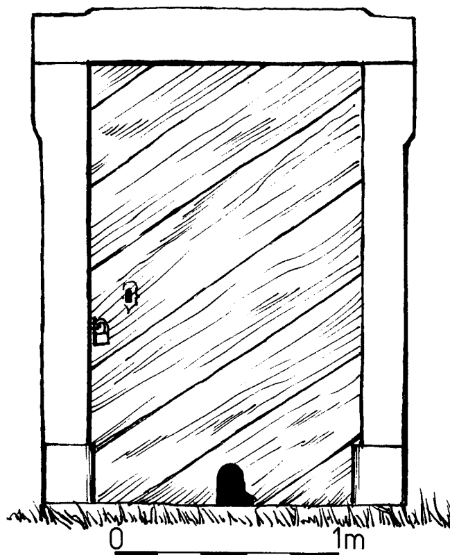
Obr. 5: Plešnice (okr. Plzeň - sever). Vstupní portál sýpky (kresba M. Novobilský, 1999).
