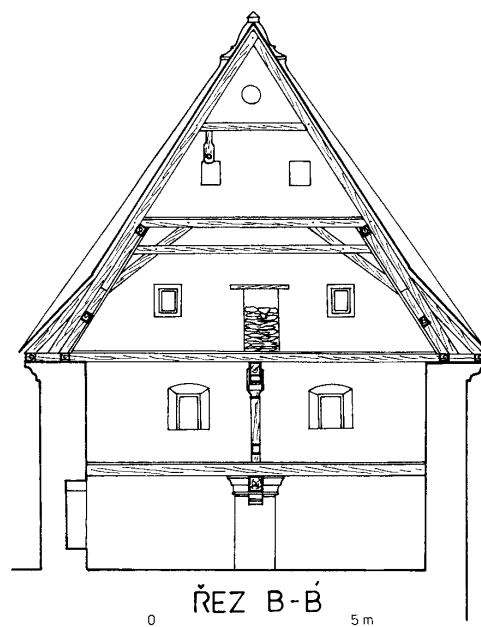
Obr. 9: Plešnice (okr. Plzeň - sever). Řez sýpkou B - B' (kresba M. Novobilský, 2000).
