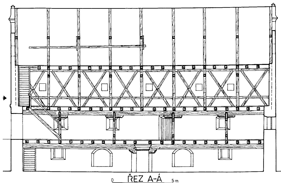
Obr. 10: Plešnice (okr. Plzeň - sever). Řez sýpkou A - A' (kresba M. Novobilský, 2000).
