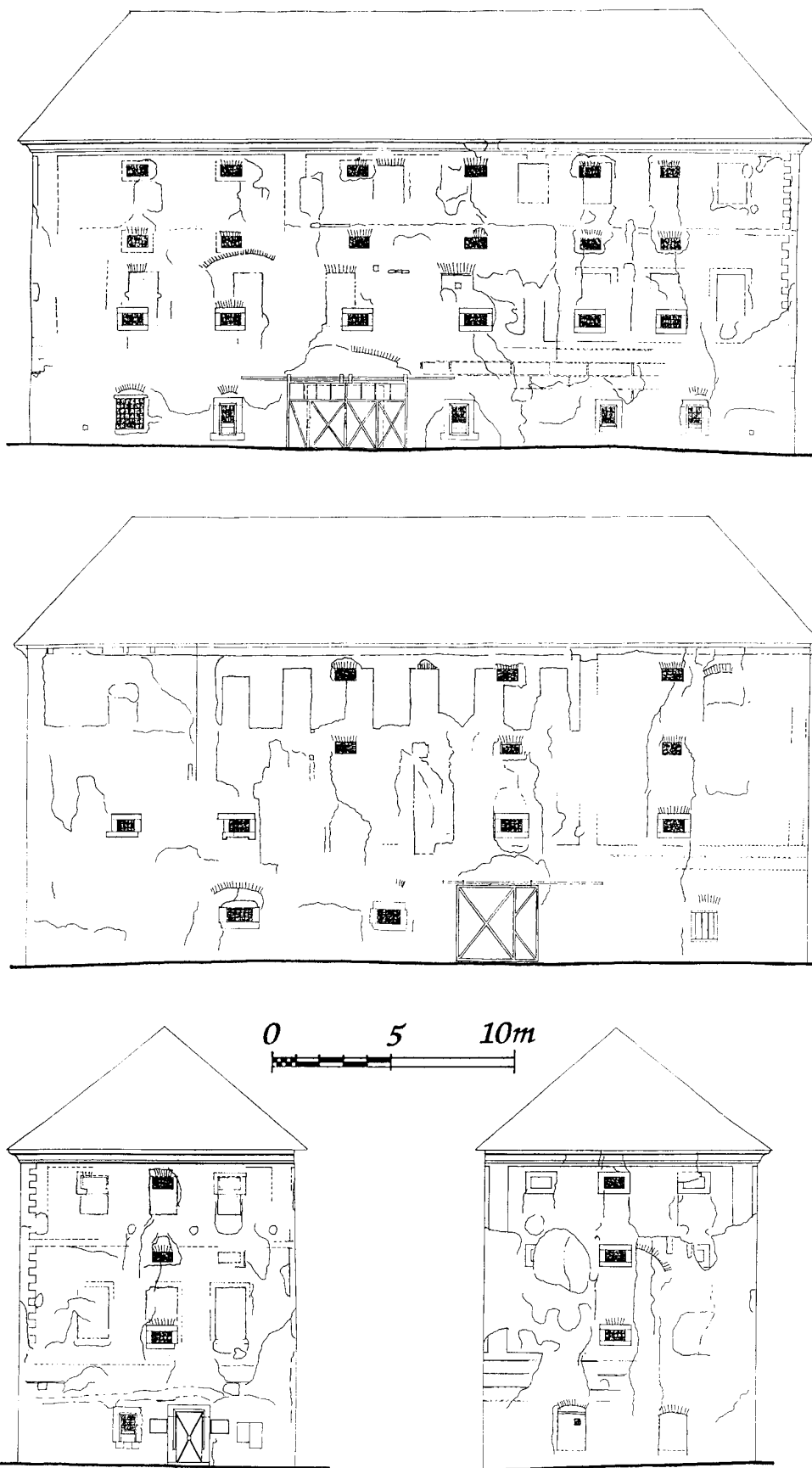
Obr. 4: Dohalice, nárysy (shora) jižního, severního, východního a západního průčelí sýpky (zpracoval L. Svoboda, 1999, s použitím zaměření M. Poura).
