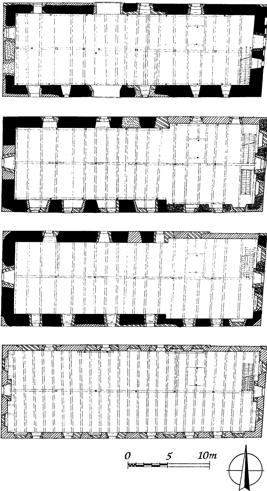
Obr. 3: Dohalice, půdorysy (shora) přízemí, 1., 2. a 3. patra sýpky se stavebně historickou analýzou (zpracoval L. Svoboda, 2000, s použitím zaměření M. Poura). Černě značeno zdivo gotické, šrafovaně barokní, dvojitou šrafovou klasicistní a tečkovaně novodobé; přerušovaně značeno zařízení hypotetické.
