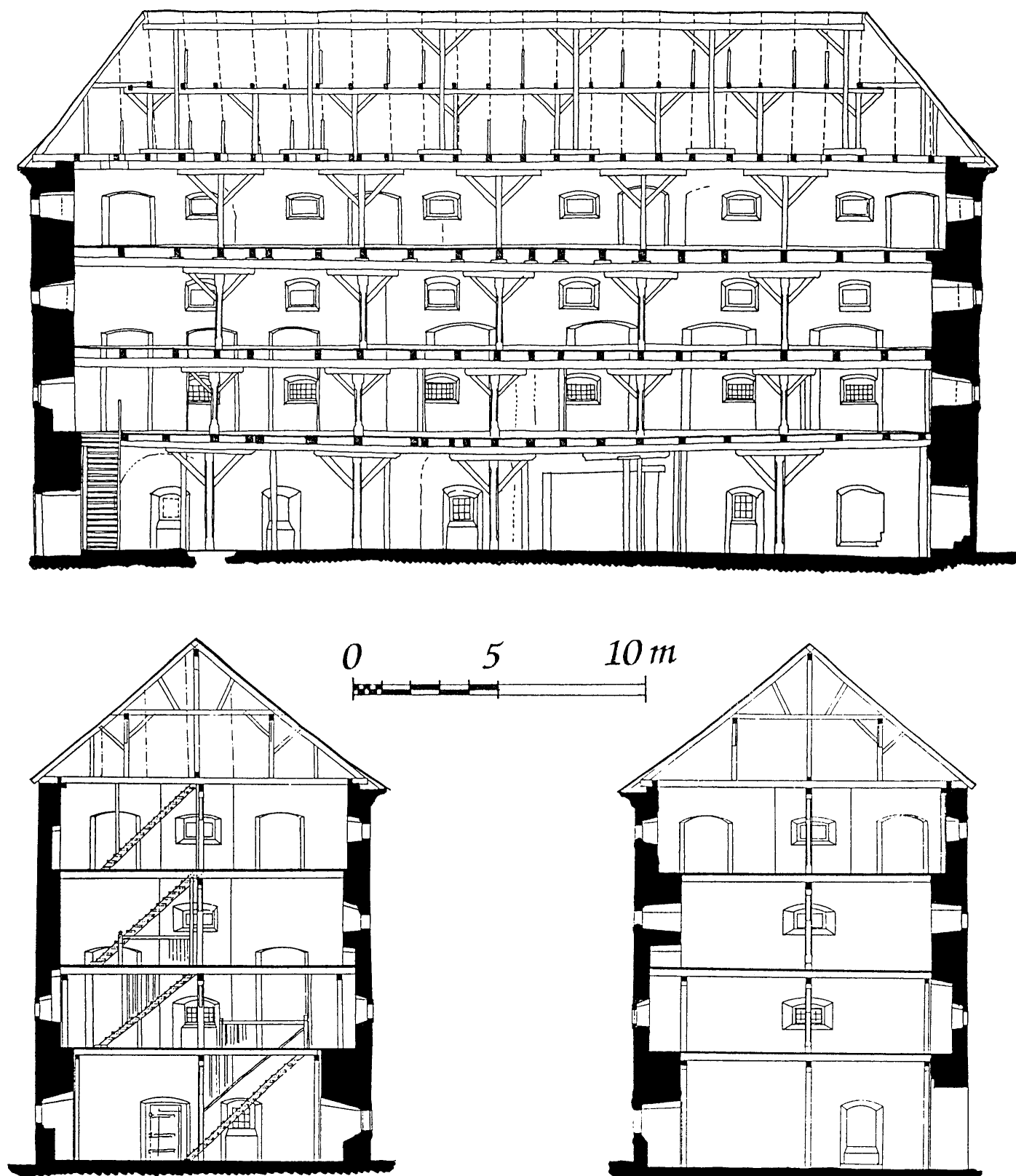
Obr. 5: Dohalice, řezy sýpkou s pohledem (shora) k jihu, k východu a k západu (zpracoval L. Svoboda, 2000, s použitím zaměření M. Poura).
